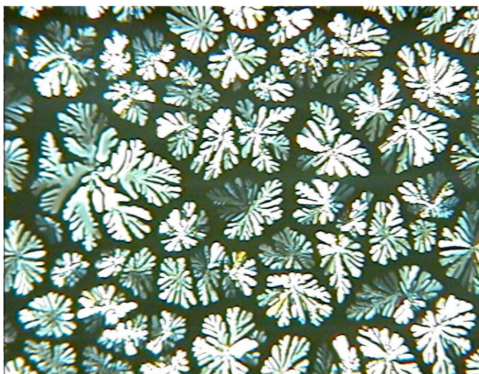
Abbildung 3-17: Polarisationsmikroskopische Aufnahme (x200) eines Filmes von 3-13 , aufgenommen zwischen zwei Glasplättchen und nach Abkühlen auf 30 °C aus der Schmelze mit 1 °C/min. Das Muster zeigt eine flüssigkristalline Phase, bei der die Spalten senkrecht zum Substrat orientiert sind. Gekreuzte Polarisatoren.
