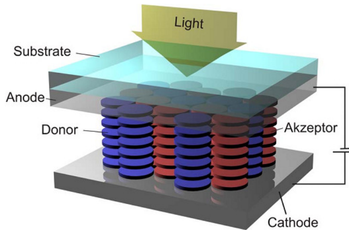
Abbildung 1-15: Schematischer Aufbau einer Solarzelle [53]
