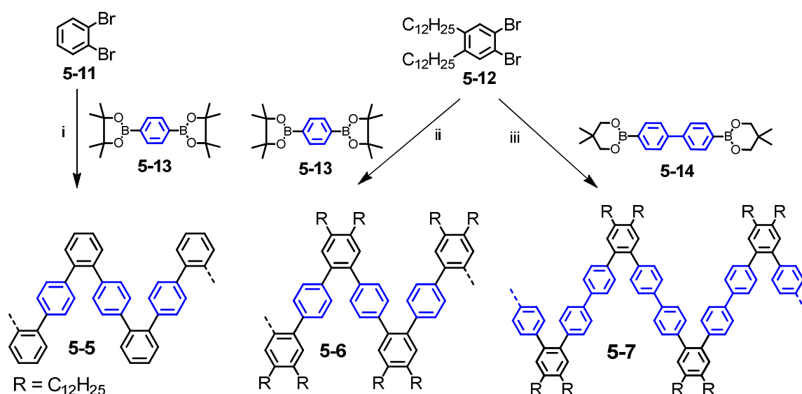
Abbildung 5-6: Synthese der Polyphenylen-Vorläufer 5-5 – 5-7 durch Suzuki-Polymerisation aus einem o -Dibrombaustein und einer p -Diborsäure unter Katalyse durch \text{Pd}(\text{PPh}_3)_4 , Aliquat 336 und \text{K}_2\text{CO}_3 in Toluol/ \text{H}_2\text{O} . i) 74 %; ii) 79 %; iii) 71 %.
