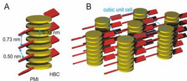
Abbildung 3-36: Schematische Darstellung der supramolekularen Ordnung für das HBC-1PDI 3-36 in der Kolumne (a) und kubische Anordnung der Spalten (b), bestimmt durch 2D-WAXS. [36c, 37]
