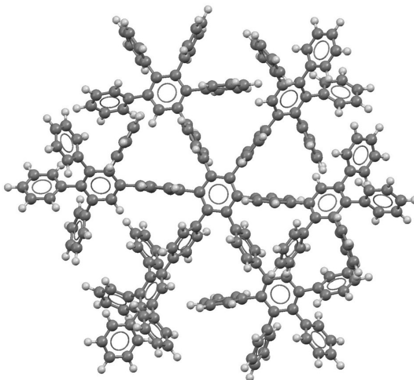
Abbildung 4-3: Computer-simuliertes Modell der dreidimensionalen Struktur der Polyphenylen-Vorstufe 4-1 (Energieminimierung mittels der Software Spartan V1.2.0 von Wavefunction Inc.).
