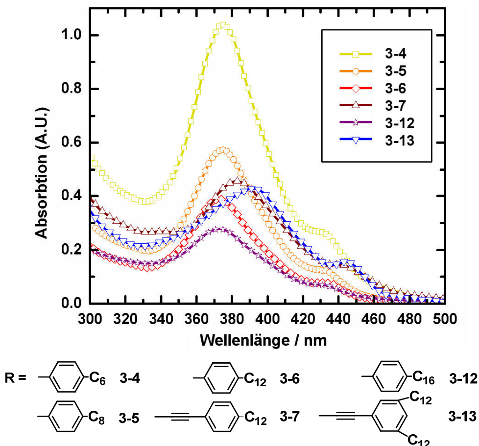
Abbildung 3-32: Absorptionsspektren der HBC-Derivate in Filmen von ca. 100 nm Dicke auf Quarzglas, hergestellt durch Rotationsbeschichtung aus Chloroform-Lösung.
