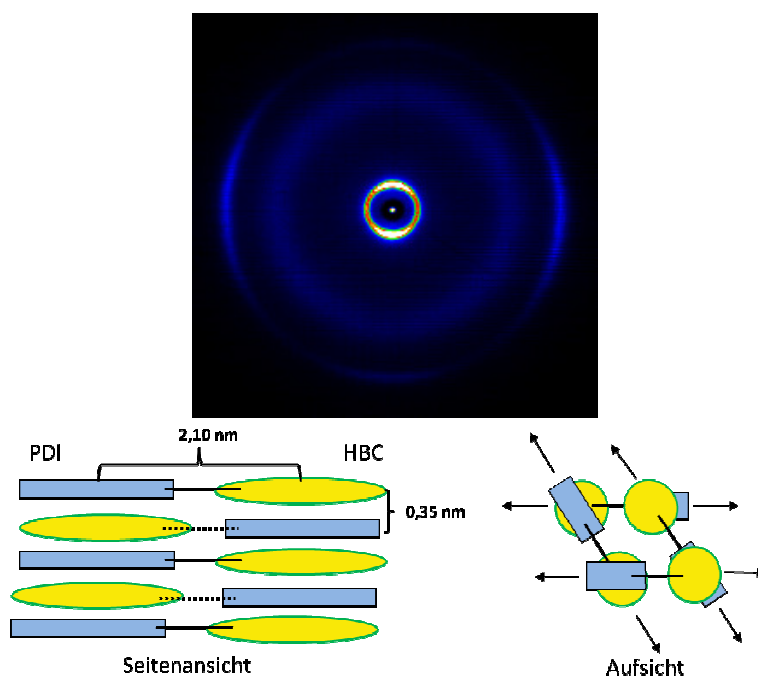
Abbildung 3-52: 2D-WAXS-Muster der Dyaden 3-38 – 3-41, aufgenommen nach Extrusion in eine Faser bei erhöhter Temperatur; Schematische Darstellung der ermittelten Strukturen.
