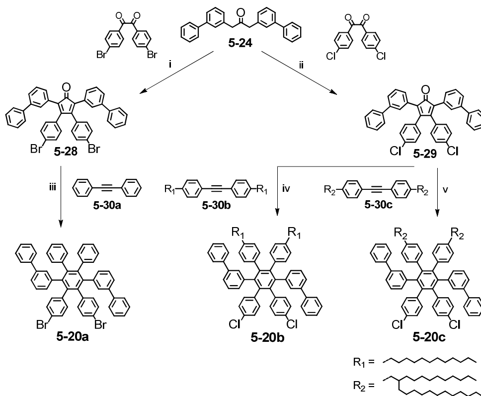
Abbildung 5-33: Syntheseschema zur Darstellung der Monomere 5-20 a-c für die Yamamoto-Polymerisation. i) Tetrabutylammoniumhydroxid, 77 %; ii) Tetrabutylammoniumhydroxid, 53 %; iii) Ph 2 O, 40 %; iv) Ph 2 O, 56 %; v) Ph 2 O, 41 %.
