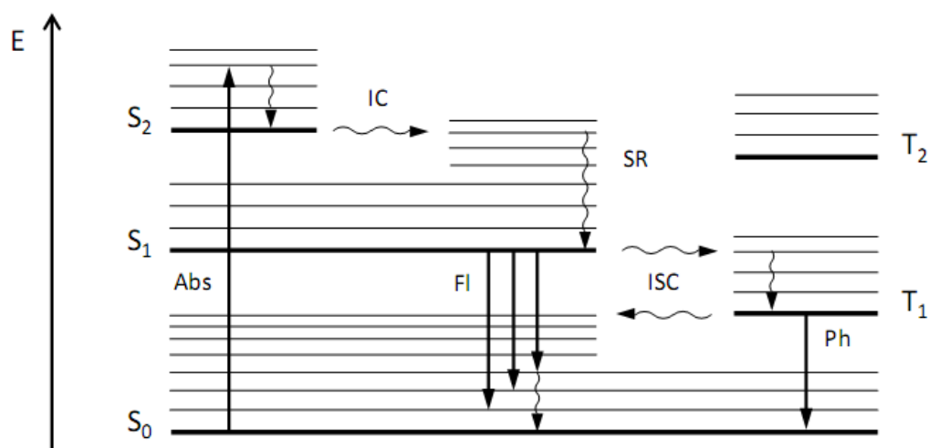
Abbildung 1-17: Jablonski-Diagramm zur Veranschaulichung der Prozesse nach einem Absorptionsprozess. S (Singulett) und T (Triplett) bezeichnen elektronische Zustände, die dünnen waagerechten Linien repräsentieren Schwingungszustände. Mögliche Prozesse zur Rückkehr in den Grundzustand S_0 : Schwingungsrelaxation (SR), Innere Konversion (IC), Intersystemcrossing (ISC) und Emission eines Photons durch Phosphoreszenz (Ph) oder Fluoreszenz (Fl). [81]
