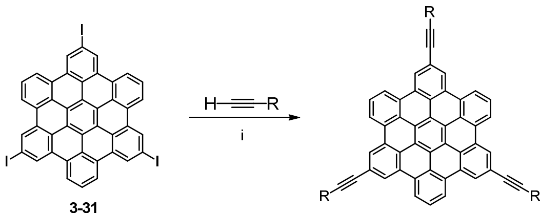
Abbildung 3-11: Syntheschema für Ethynylen-verbrückte HBC-Derivate mit C3-Symmetrie; i) \text{Pd}(\text{PPh}_3)_4 , \text{CuI} , 35-62 %
