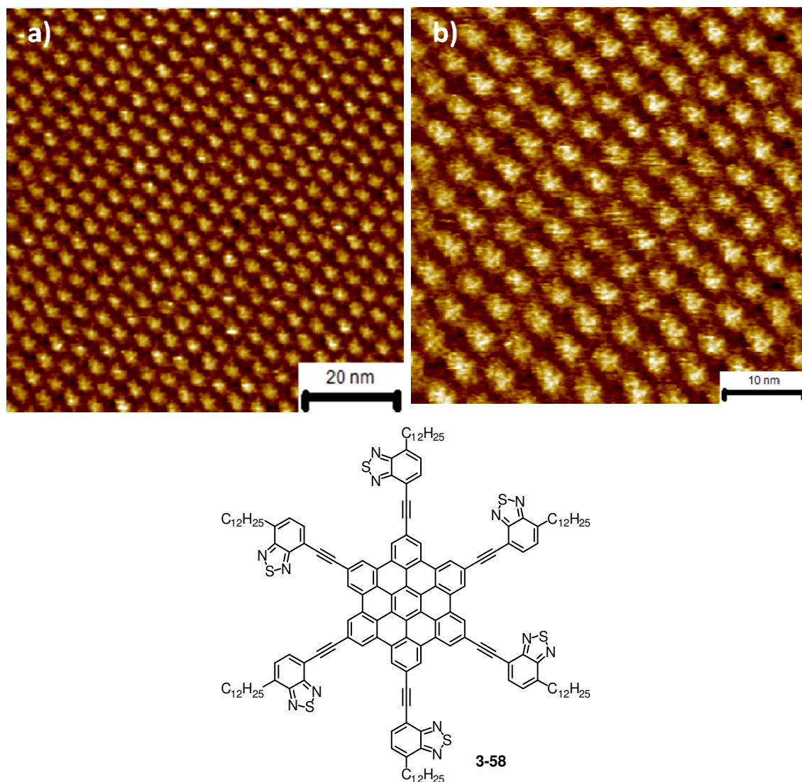
Abbildung 3-66: STM-Aufnahmen des HBC-6BTZ 3-58 , aufgenommen an der Flüssig-Fest-Grenzfläche Trichlorbenzol / HOPG. a) i_T = 80 \text{ pA} , V_S = -800 \text{ mV} ; b) i_T = 80 \text{ pA} , V_S = -900 \text{ mV} .
