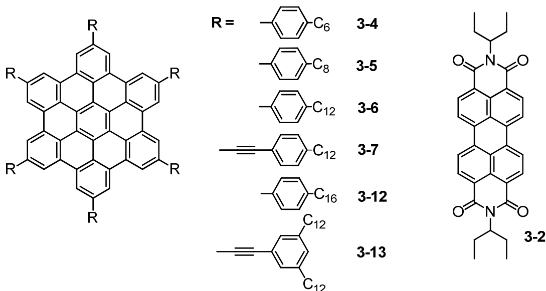
Abbildung 3-28: Chemische Strukturen der untersuchten HBCs und des kommerziellen PDIs (3-2)
