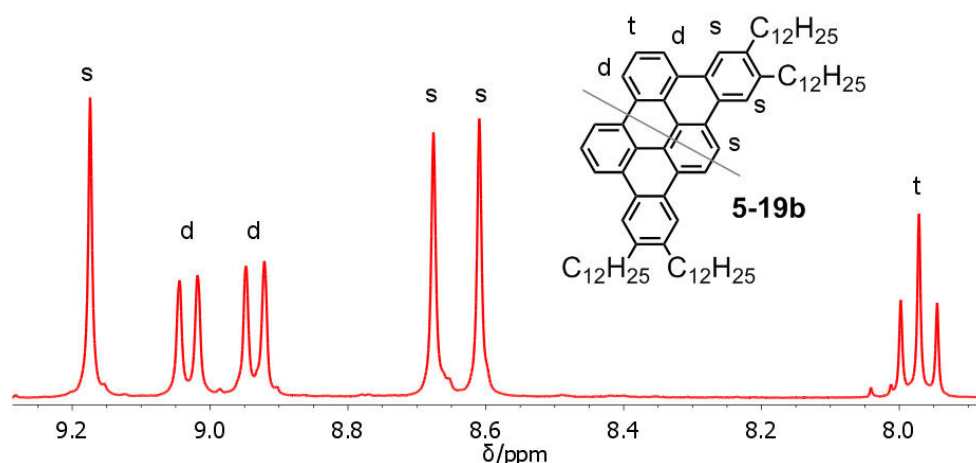
Abbildung 5-8: Relevanter Bereich des ^1\text{H} -NMR-Spektrum der dehydrierten Modellverbindung 5-19b . Aufgenommen in d_8 -THF (300 MHz, RT).
