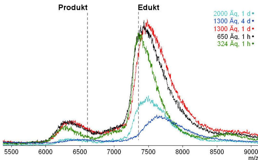
Abbildung 4-19: MALDI-TOF-Massenspektren der Rohprodukte nach Dehydrierung des C_{582} -Vorläufers 4-10 in Abhängigkeit von der Anzahl Äquivalenten an FeCl_3 und der Reaktionsdauer; lösungsmittelfreie Probenvorbereitung mit TCNQ als Matrix, linearer Messmodus.
