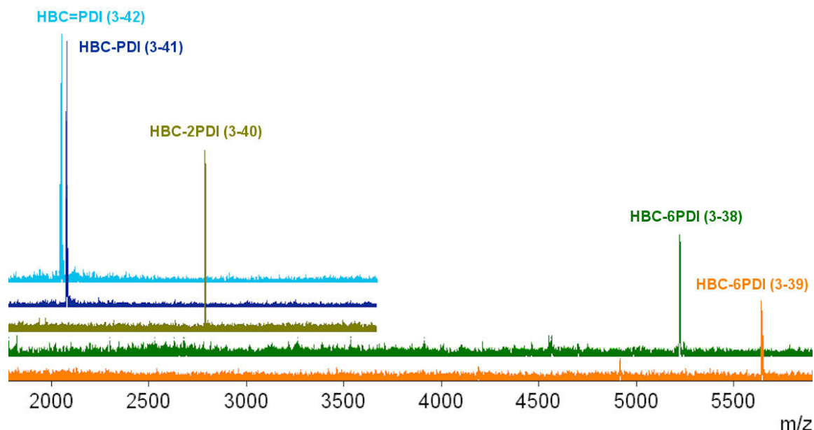
Abbildung 3-50: MALDI-TOF-Massenspektren der Dyaden 3-38 – 3-42 . Messmodus: 3-38 : lösungsmittelfrei mit TCNQ als Matrix; 3-39 : lösungsmittelfrei mit Luftmann-Matrix, negative Ionisierung; 3-40 und 3-41 : aus THF-Lösung mit Dithranol-Matrix; 3-42 : aus DCM-Lösung mit Dithranol-Matrix.
