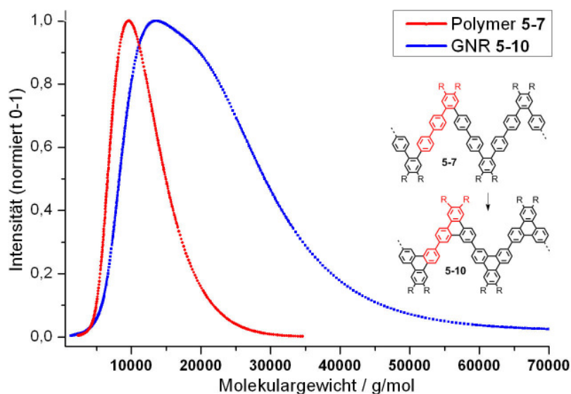
Abbildung 5-20: Durch GPC-Analyse bestimmte Molekulargewichtsverteilungen des Polymer-Vorläufers 5-7 (rot) und des dehydrierten Produktes 5-10 (blau), berechnet gegen einen PS-Standard, Lösungsmittel THF, UV-Detektor.
