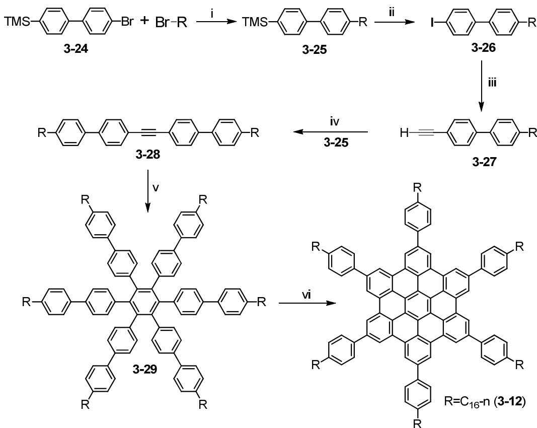
Abbildung 3-5: Syntheseroute zur Darstellung von 3-12 ; i) \text{Zn} , \text{PdCl}_2(\text{dppf}) , 77 %; ii) \text{ICl} , 96 %; iii) TIPS-Acetylen, \text{Pd(PPh}_3)_4 , \text{CuI} , \text{TBAF} , 74 %; iv) \text{Pd(PPh}_3)_4 , \text{CuI} , 62 %; v) \text{Co}_2(\text{CO})_8 , 41 %; vi) \text{FeCl}_3 ; 81 %
