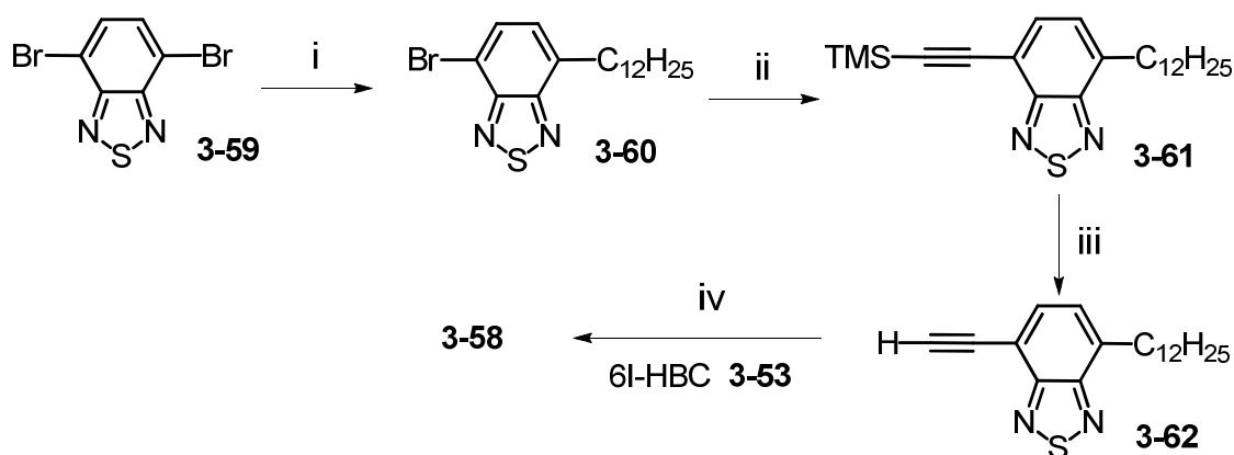
Abbildung 3-63: Syntheseroute zur Darstellung des HBC-6BTZ 3-58 mit einer konjugierten Ethinylen-Brücke; i) 1-Dodecylbromid, Zn, PdCl 2 (dppf), 52 %; ii) TMS-Acetylen, Pd(PPh 3 ) 4 , CuI, 84 %; iii) TBAF, 91 %; iv) Pd(PPh 3 ) 4 , CuI, 64 %.
