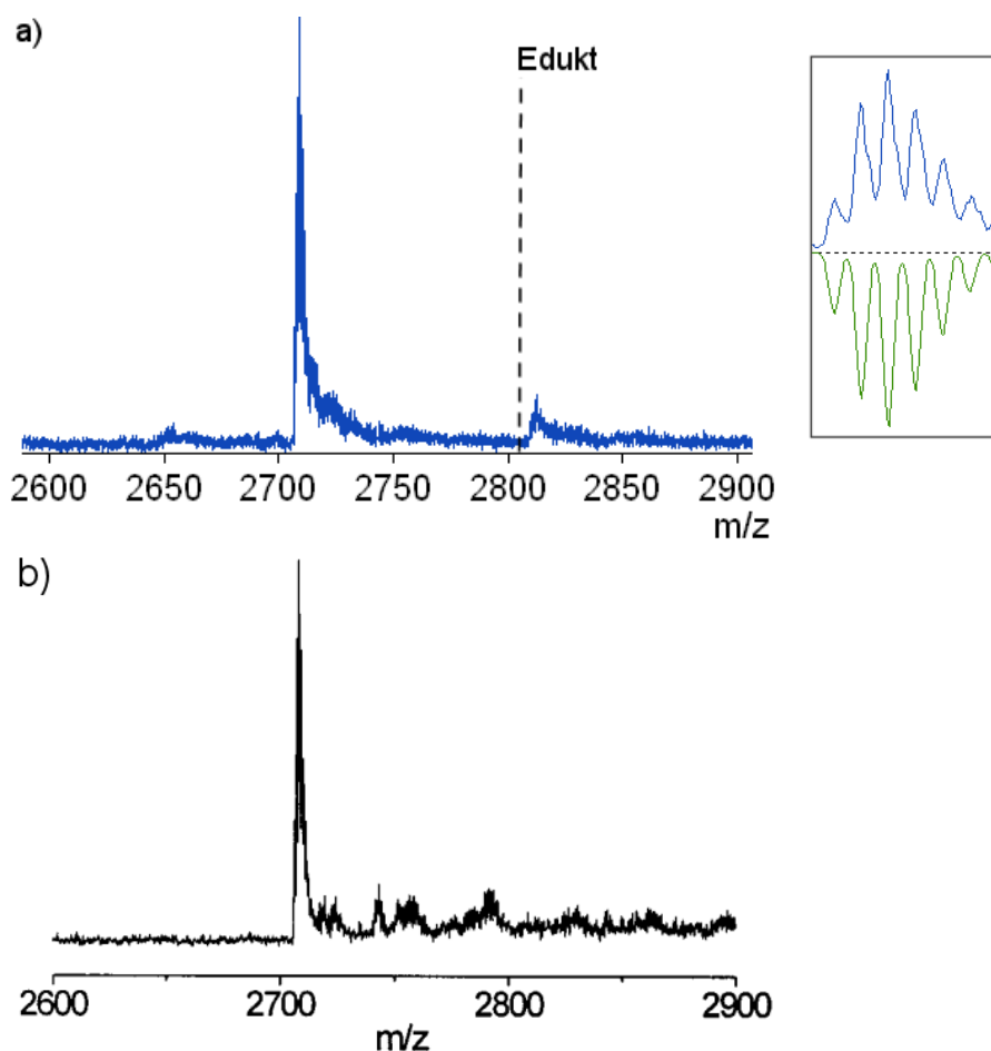
Abbildung 4-10: MALDI-TOF-Massenspektrum des C_{222} -Nanographens 4-2 , Lösungsmittelfreie Proben-vorbereitung mit TCNQ als Matrix. a) neue Syntheseroute über vorplanarisierten Vorläufer 4-3 , Kasten: Vergrößertes Isotopenmuster (gemessen: blau, berechnet: grün); b) alte Route über Vorläufer 4-1 [13, 20] .
