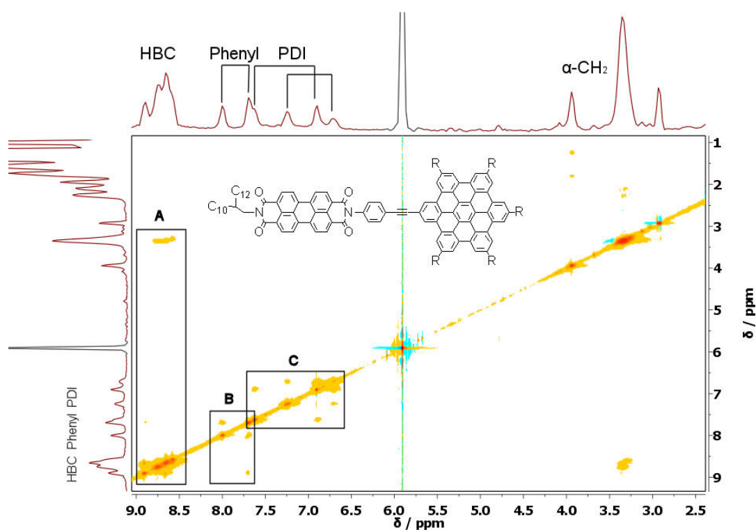
Abbildung 3-49: Relevanter Ausschnitt aus dem ^1\text{H} - ^1\text{H} -NOESY-Experiment der Dyade HBC=1PDI 3-42 . Aufgenommen in \text{d}_2\text{-TCE} (500 MHz, 120 °C). Lösungsmittelsignale in grauer Farbe.
