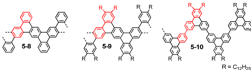
Abbildung 5-15: Strukturen der synthetisierten Nanostreifen 5-5 – 5-8
