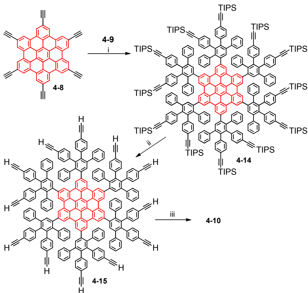
Abbildung 4-16: Syntheseroute zur Darstellung des G2-Dendrimers 4-10 als Vorstufe zur Dehydrierung zu einem C_{546} Nanographen. i) A_2B -Baustein, TCE, Mikrowellenbestrahlung, 61 %; ii) TBAF, 51 %; iii) Tetraphenylcyclopentadienon, Mikrowellenbestrahlung, 8 %.
