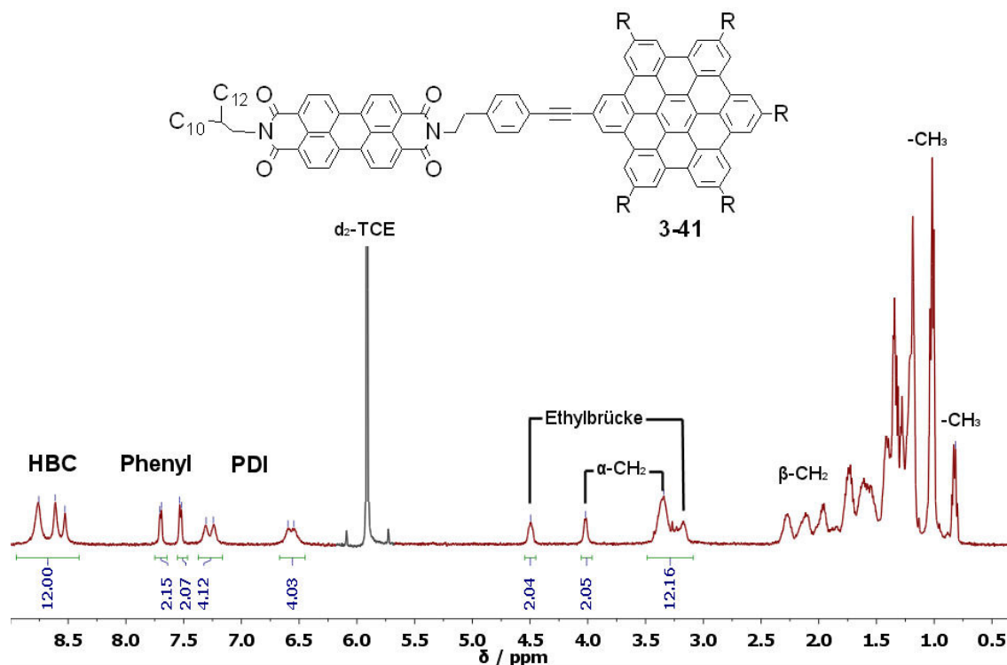
Abbildung 3-45: ^1\text{H} -NMR-Spektrum der Dyade HBC-1PDI 3-41 . Aufgenommen in d_2 -TCE (500 MHz, 120 °C). Lösungsmittelsignale in grauer Farbe.
