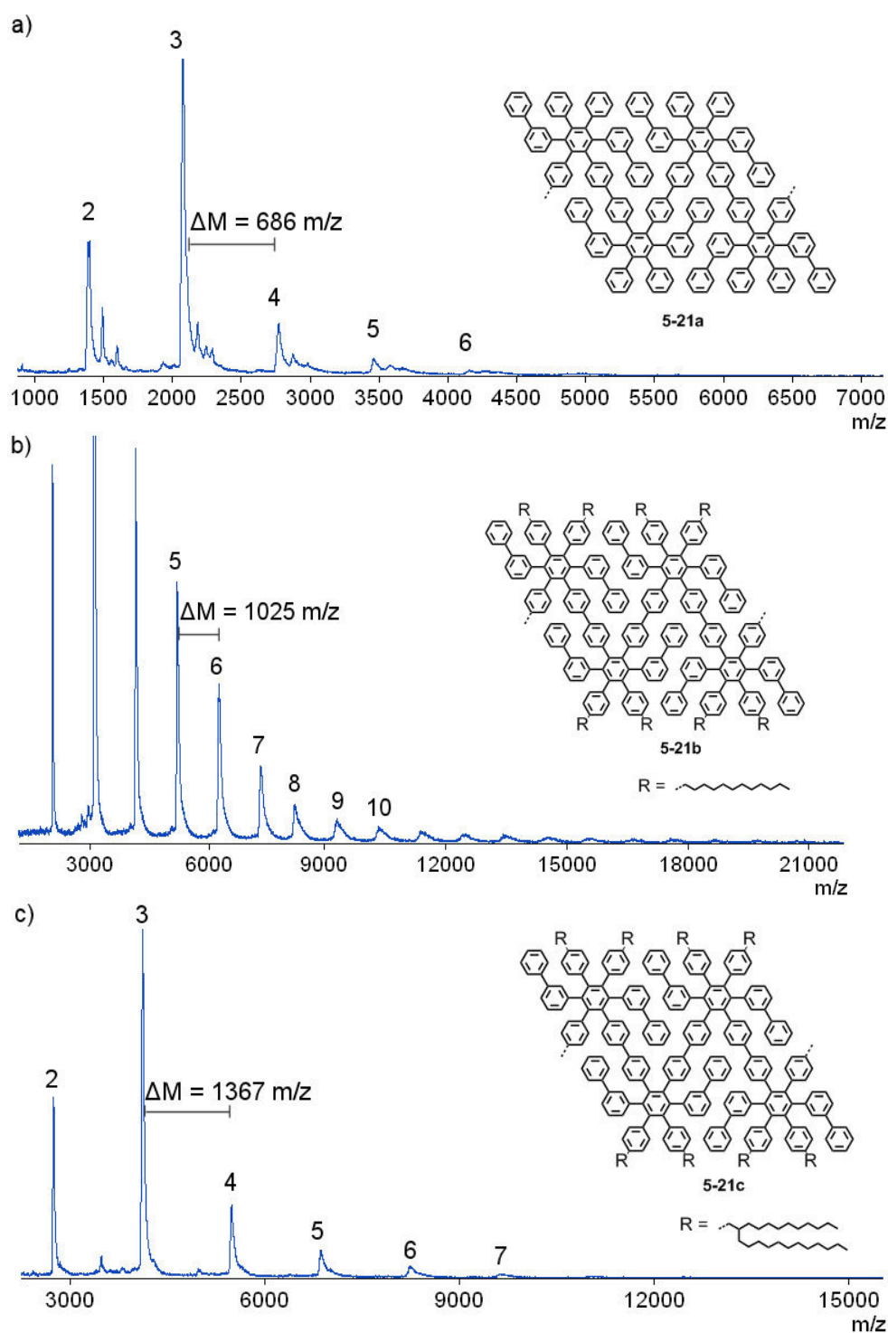
Abbildung 5-38: MALDI-TOF-MS der unfractionierten Polyphenylen-Vorläufer 5-21a (a), 5-21b (b) und 5-21c (c) mit verschiedenen Alkylresten. Lösungsmittelfreie Probenvorbereitung mit TCNQ als Matrix, linearer Messmodus.
