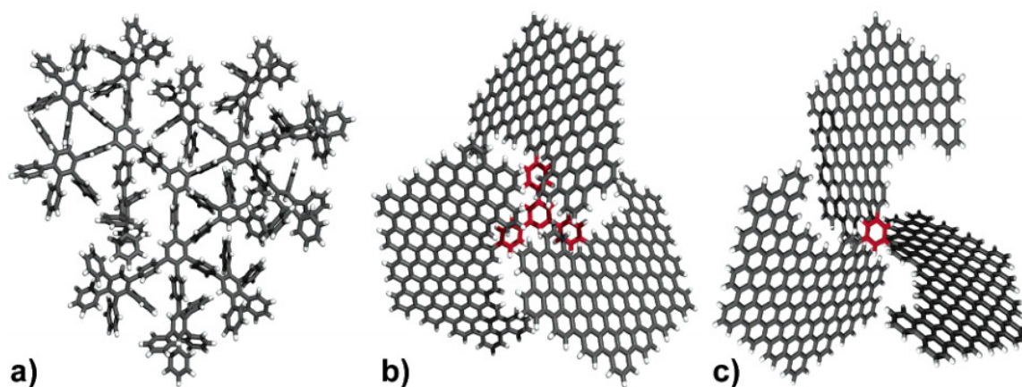
Abbildung 4-4: Computer-simulierte Modelle der dreidimensionalen Struktur der Polyphenylen-Vorstufe eines \text{C}_{474} -Nanographens (a) und der vermutlich entstandenen Produkte bei der Cyclodehydrierung (b, c) (Energiminimierung mittels der Software Spartan V1.0.5 von Wavefunction Inc.). [17]
