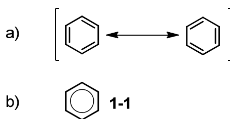
Abbildung 1-1: a) Kekulé- und b) Robinson-Struktur von Benzol
