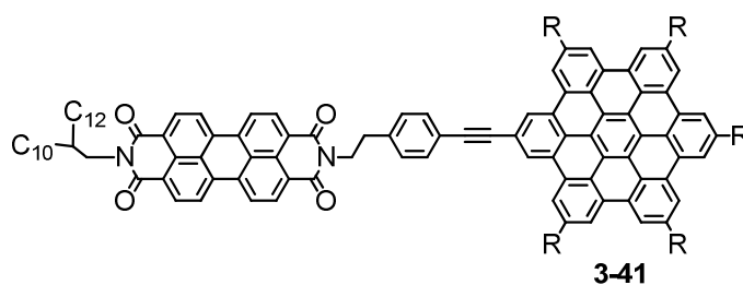
Abbildung 3-57: Konzentrationsabhängige Fluoreszenz des HBC-PDI 3-41 in Toluol mit ( c_1 = 1 \cdot 10^{-7} \text{ mol/L} , c_2 = 5 \cdot 10^{-7} \text{ mol/L} , c_3 = 1 \cdot 10^{-6} \text{ mol/L} , c_4 = 5 \cdot 10^{-6} \text{ mol/L} , c_5 = 1 \cdot 10^{-5} \text{ mol/L} ) bei einer Anregung des HBCs bei \lambda_{\text{exc}} = 488 \text{ nm} (a) und des PDIs bei \lambda_{\text{exc}} = 405 \text{ nm} (b).
