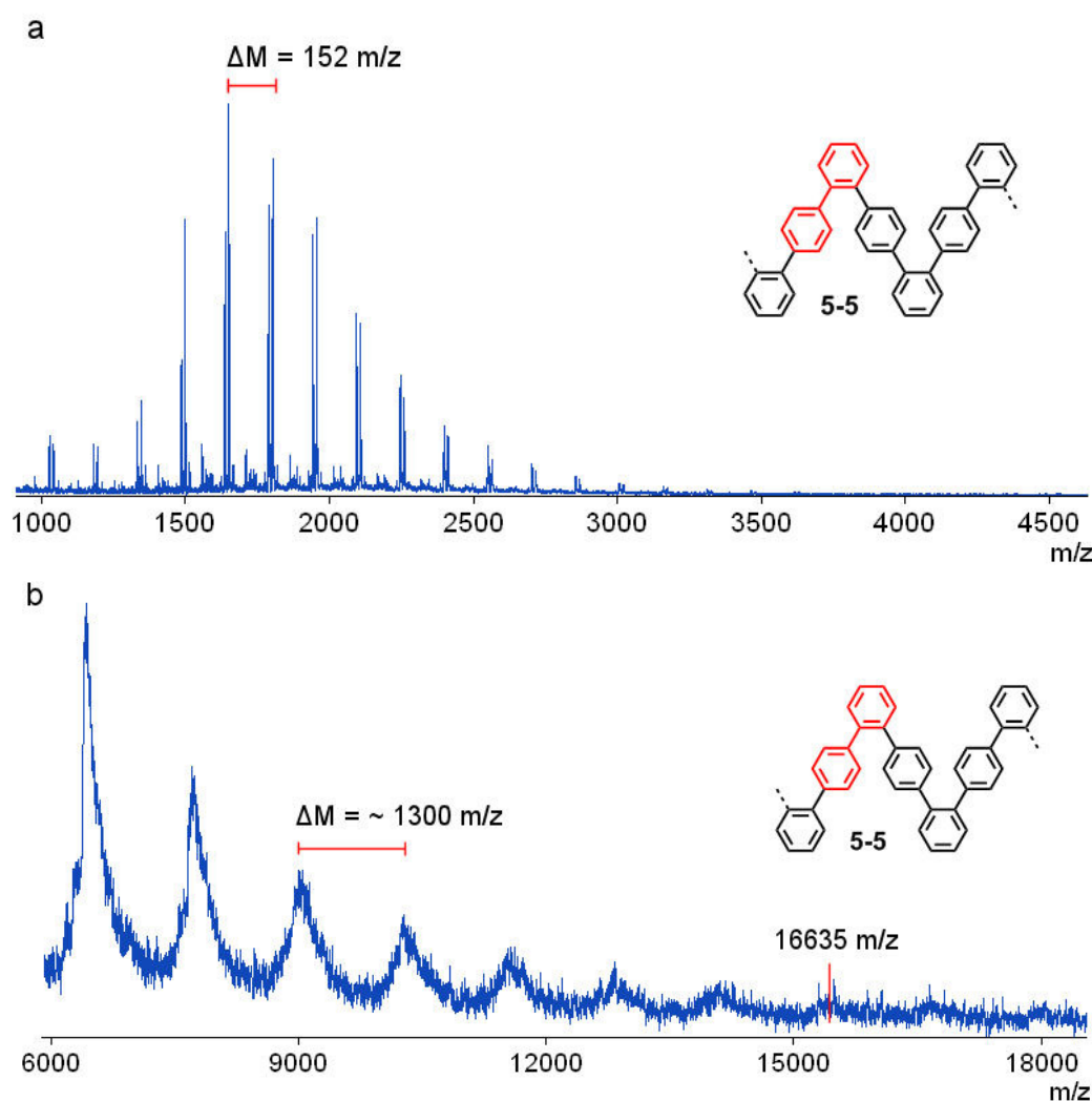
Abbildung 5-11: MALDI-TOF-MS der löslichen ( a , THF, Dithranol-Matrix) und der unlöslichen Fraktion ( b , lösungsmittelfreie Probenvorbereitung, TCNQ-Matrix, linearer Messmodus) des GNR-Vorläufers 5-5 .
