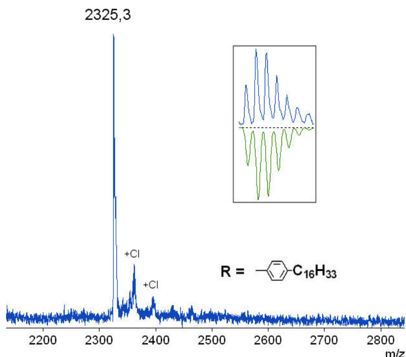
Abbildung 3-6: MALDI-TOF-Massenspektrum von HBC-Ph-C16 3-12 , lösungsmittelfreie Probenvorbereitung mit TCNQ als Matrix. Kasten: Vergrößertes Isotopenmuster (gemessen: blau, berechnet: grün)
