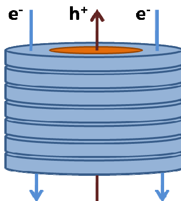
Abbildung 3-40: Schematische Darstellung der Dyaden-Kolumnen 3-38 und 3-39 als „coaxiale Kabel“, die sowohl Transportwege für Löcher als auch für Elektronen aufweisen. Der braune HBC-Kern agiert dabei ein Lochleiter, während das blau dargestellte PDI ein Elektronenleiter ist.
