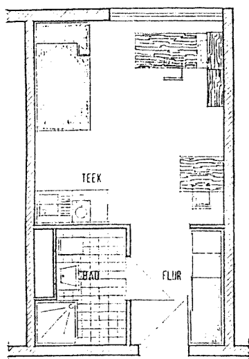
GRUNDRISS
