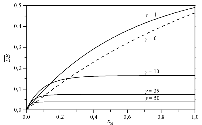
Fig. 1.2-13: Abhängigkeit des Verzweigungsgrads \overline{DB} von x_M für unterschiedliche Comonomerenverhältnisse \gamma ; (---): SCVP
