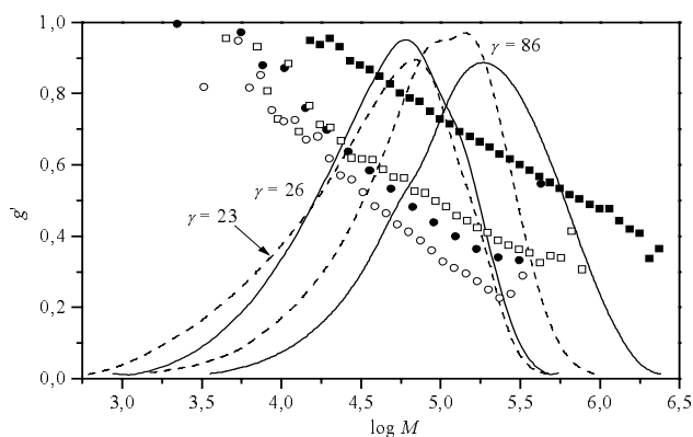
Fig. 4.5-10: Vergleich der Schrumpfungsparmeter der nichtdeuterierten Proben CM11/100 ( \gamma = 86 , ■) und CM12 ( \gamma = 26 , ●), (—): RI-Signal mit den deuterierte Proben CM31 ( \gamma = 86 , □) und CM30 ( \gamma = 23 , ○); (- - -): RI-Signale.
