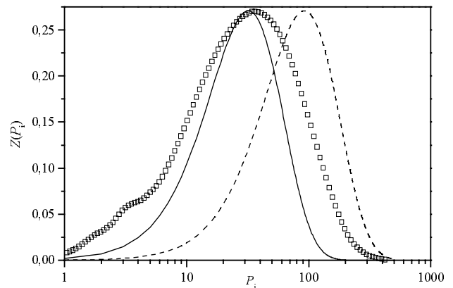
Fig. 4.4-2: Vergleich der höhennormierten z -Verteilung von HIT 20 ( \square ) und nach (4.4-1) berechneten Werten für \bar{P}_n = 16 (—) und \bar{P}_n = 46 (- -)
