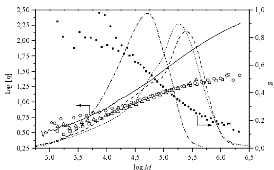
Fig. 4.5-16: intrinsische Viskosität (○, □, △), Schrumpungsparameter (■, ●, ▲) und RI-Signale (· · · ·, - - -, - · - ·) der Copolymerisation von MTSHEMA mit MMA unter Semibatch- und Batch-Bedingungen. Lauf CM14 ( I_0 = 5,2 \cdot 10^{-2} \text{ molL}^{-1} ; \gamma = 10 ; \chi = 2500 , TBABB). Symbole siehe Tab. 4.5-5. (—): intrinsische Viskosität von linearem PMMA .
