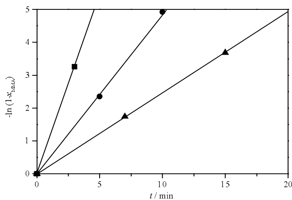
Fig. 4.2-1: Zeit–Umsatz–Auftragung der Copolymerisation von MTSHEMA mit MMA für unterschiedliche Konzentration an TBABB. Experimentelle Bedingungen und Symbole siehe Tab. 4.2-1
