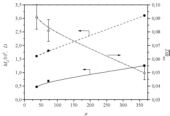
Fig. 4.5-21: Abhängigkeit der Zahlenmittel des Molekulargewichts (—■—), des Polydispersitätsindex (- - ● - -) und des apparenten Verzweigungsgrad (- · - △ · -) vom Initiatorverhältnis \mu eines monofunktionalen Initiators unter Semibatch Bedingungen
