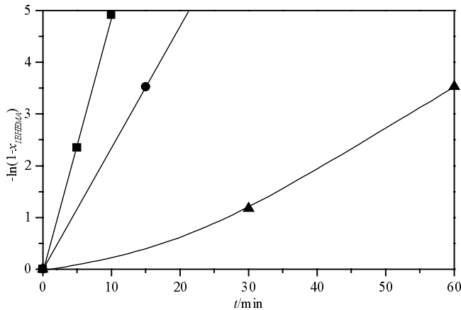
Fig. 4.2-5: Zeit-Umsatz-Auftragung für verschiedene Reaktionstemperaturen. Reaktionsbedingungen und Symbole siehe Tab. 4.2-3.
