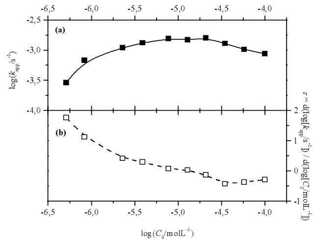
Fig. 4.2-3: Doppellogarithmische Auftragung (a) der apparenten Geschwindigkeitskonstante k_{\text{app}} (—■—) und (b) der Reaktionsordnung \tau = d(\log[k_{\text{app}} / \text{s}^{-1}]) / d(\log[C_0 / \text{molL}^{-1}]) gegen die Katalysatorkonzentration C_0 (—□—) für die GTP mit MMA/MTS/TBABB in THF bei 293 K. Nach Gores. 182
