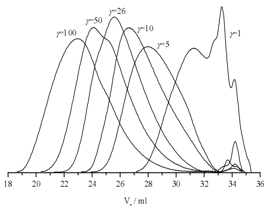
Fig. 4.5-1: Flächennormierte RI-Eluogramme der Copolymerisation von MTSHEMA mit MMA für unterschiedliche Comonomerenverhältnisse \gamma
