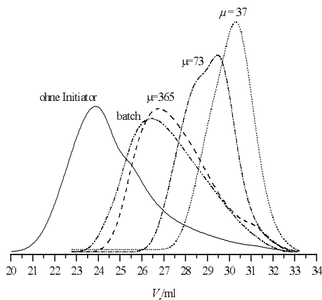
Fig. 4.5-19: Eluogramme der Copolymerisation von MMA mit MTSHEMA im Semibatch in Gegenwart von MTS für verschiedene Initiatorverhältnisse \mu . Linientypen siehe Tab. 4.5-6
