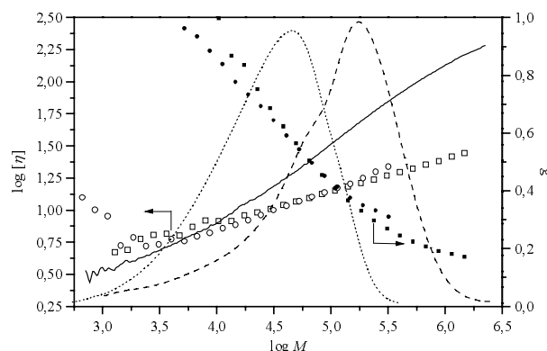
Fig. 4.5-17: Viskositätsergebnisse (○, □), Schrumpungsparameter (■, ●) und RI-Signale (· · · ·, - - -, - · - ·) der Copolymerisation von MTSHEMA mit MMA unter Semibatch- und Batch-Bedingungen; Lauf CM15 ( I_0 = 2,7 \cdot 10^{-2} \text{ molL}^{-1} ; \gamma = 25 ; \chi = 700 ). Symbole siehe Tab. 4.5-5. (—): intrinsische Viskosität von linearem PMMA .
