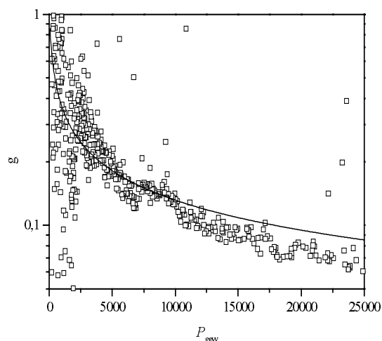
Fig. 4.3-11: Auftragung des Schrumpfungsfaktors g' als Funktion des gewichteten Polymerisationsgrads P_{\text{gew}} zur Bestimmung des Anteils an Verzweigungspunkten. (—): Ausgleichsgerade nach (4.3-11) für (\gamma' + 1) = 28,0 .
