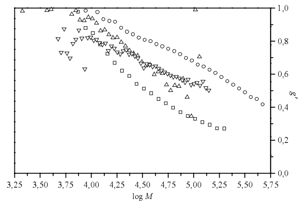
Fig. 4.7-3: Auftragung des Schrumpfungparameters der Viskosität g' als Funktion des Molekulargewichts für die Copolymerisation von MSTHEMA mit tBMA. Symbole siehe Tab. 4.7-1
