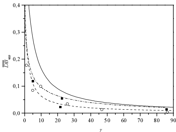
Fig. 4.5-15: Auftragung des Verzweigungsgrads \overline{DB} als Funktion von \gamma und Vergleich mit der Theorie. (○): nichtdeuterierte Polymere; (■): deuteriertes PMMA; (—): Verlauf für identische Reaktivität; (- · - · -): r_1 = 1; \alpha = 0,1 ; (- - -): r_1 = 0,1; \alpha = 0,1 .
