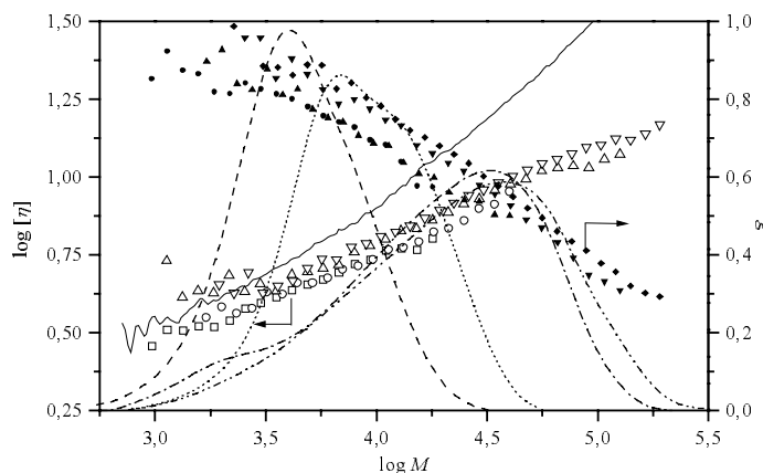
Fig. 4.5-20: Mark-Houwink Auftragung ( \square, \circ, \triangle, \nabla ) und Abhängigkeit des Schrumpfungsp Parameters g^1 ( \blacksquare, \bullet, \blacktriangle, \blacktriangledown ) der Copolymerisation von MMA mit MTSHEMA im Semibatch in Gegenwart von MTS für verschiedene Initiatorverhältnisse \mu . Linientypen des RI-Signals und Symbole siehe Tab. 4.5-6. (—): intrinsische Viskosität von linearem PMMA
