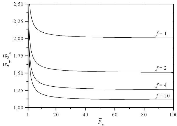
Fig. 1.2-9: Abhängigkeit des Polydispersitätsindex vom Zahlenmittel des Polymerisationsgrad für unterschiedliche Initiatorfunktionalitäten f im Semi-Batch-Verfahren (langsameres Zutropfen)
