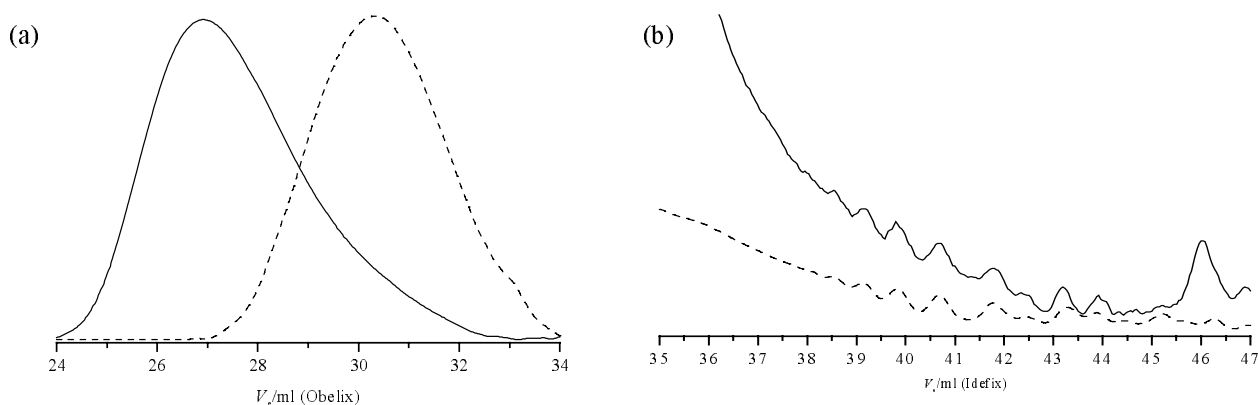
Fig. 4.4-5: (a) höhennormiertes Eluogramm des Precursors (---) und des daraus gebildeten Sterns (—) (Säulenkombination "Obelix") und (b) Vergrößerung des Oligomerenbereichs (Säulenkombination "Idefix")
