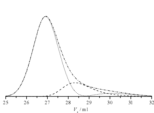
Fig. 4.5-24: Eluogramme der "Lolly-Synthese" (- · - · -): RI-Signal des resultierenden Polymers; (- - -): RI-Signal des linearen PMMA-Precursors; (· · · · ·): berechnetes RI-Signal des "Lollys" nach Abzug des Precursors
