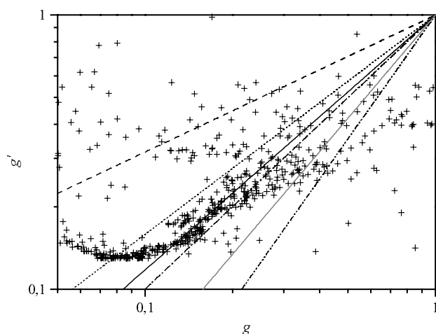
Fig. 4.3-12: Doppellogarithmische Auftragung des Schrumpfungsparemters der Viskosität g' in Abhängigkeit des Schrumpfungsparemters der Trägheitsradien g zur Bestimmung des Flory-Fox Exponenten \varepsilon . Linientyp siehe Tab. 4.3-8.
