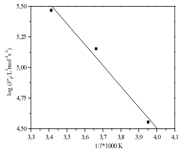
Fig. 4.2-6: Arrhenius-Auftragung für die Copolymerisation von MTSHEMA und MMA. Experimentelle Bedingungen siehe Tab. 4.2-3
