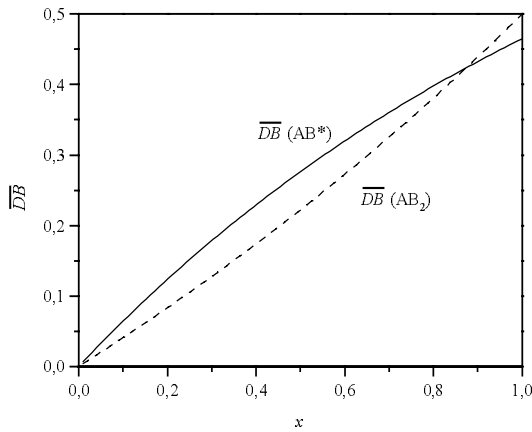
Fig. 1.2-2: Abhängigkeit des Verzweigungsgrads \overline{DB} vom Umsatz für Kondensation eines AB_2 -Monomers und die SCVP ( AB^* )
