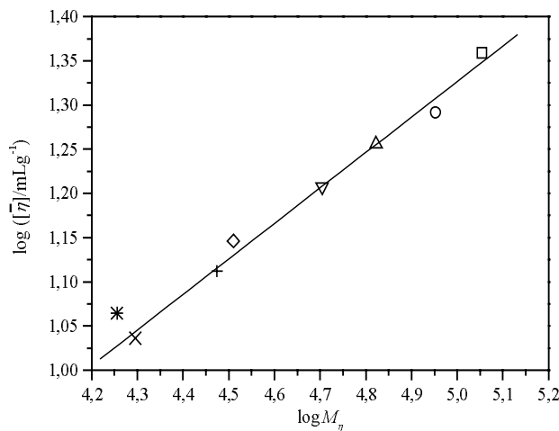
Fig. 4.6-4: Mark–Houwink Plot der intrinsischen Viskosität der einzelnen Fraktionen. Symbole siehe Tab. 4.6-1
