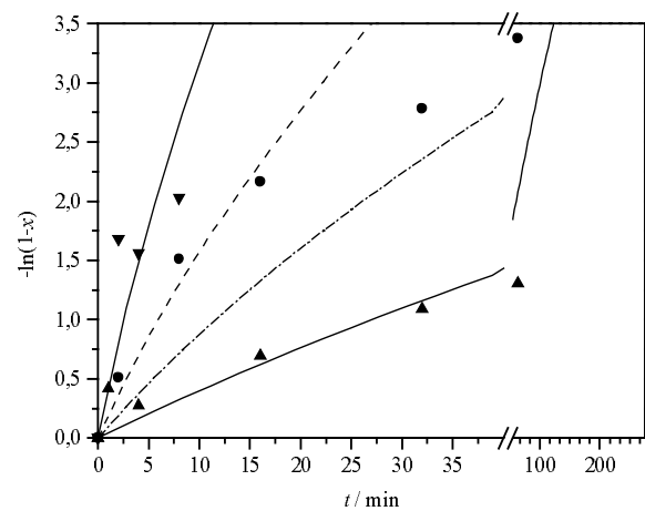
Fig. 4.1-4: Zeit-Umsatz-Auftragung erster Ordnung der Homopolymerisation von MTSHEMA unter Katalyse von TBABB bei Variation der Temperatur. Reaktionsbedingungen und Symbole siehe Tab. 4.1-2
