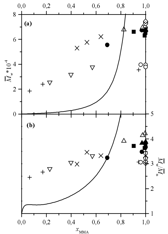
Fig. 4.2-8: Auftragung (a) des Massenmittel des Molekulargewichts M_w und (b) des Polydispersitätsindex als Funktion des Umsatzes an MMA alle Versuche; \gamma = 25,2 ; (■): CM20/20; (●): CM20/20 und (▲): CM20/0, (▽): CM21M04 und (◇): CM21M8; (○): CM23/5C und (△): CM23/5K; (+): CM22C1 und (×): CM22F, (—): eine ideale SCVCP vgl. (1.2-23) und (1.2-25)).
