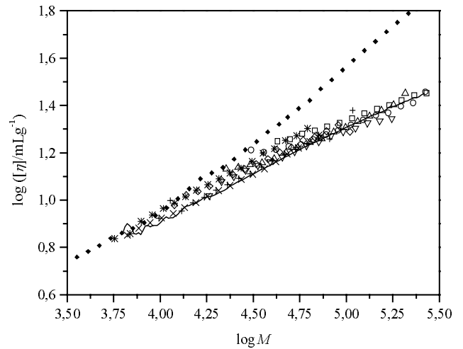
Fig. 4.6-5: Mark–Houwink Auftragung für die Fraktionen an verzweigtem PMMA (Symbole siehe Tab. 4.6-1).
