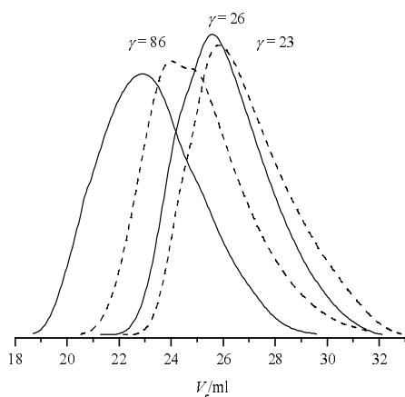
Fig. 4.5-8: Vergleich der RI-Eluogramme. (—): nichtdeuterierte Proben CM11/100 ( \gamma = 86 ) und CM12 ( \gamma = 26 ); (- - -): deuterierte Proben CM31 ( \gamma = 86 ) und CM30 ( \gamma = 23 )
