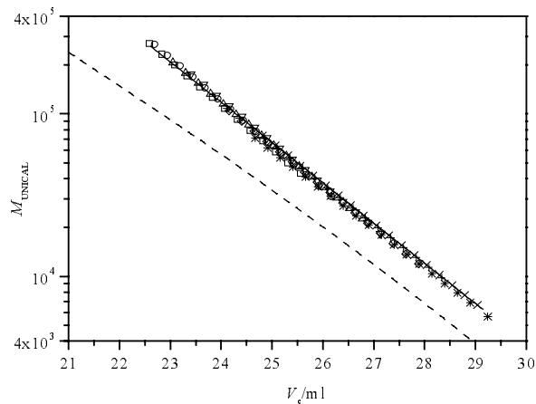
Fig. 4.6-2: UNICAL-Kalibrationskurve der unterschiedlichen Fraktionen und Vergleich mit dem Feed (—). Symbole siehe Tab. 4.6-1. (- - -): lineares PMMA
