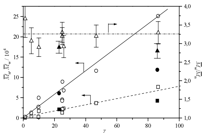
Fig. 4.5-11: Abhängigkeit des Zahlen- ( \square, \blacksquare ) und Massenmittels ( \circ, \bullet ) des Molekulargewicht und des Polydispersitätsindex ( \triangle, \blacktriangle ) vom Comonomerenverhältnis \gamma . Daten nach Tab. 4.5-1 und Tab. 4.5-4 für deuterierte ( \blacksquare, \bullet, \blacktriangle ) und nichtdeuterierte ( \square, \triangle, \circ ) Proben.
