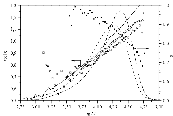
Fig. 4.5-27: Mark-Houwink Auftragung (○) und Abhängigkeit des Schrumpfungsparmeters g' (■) vom Molekulargewicht bei der SCVCP von MMA mit MTSHEMA im Semibatch RI-Signal: (- · - · -) mit bifunktionellem PMMA Precursor RI-Signal: (· · · · ·). Zum Vergleich (—):intrinsic Viskosität von linearem PMMA
