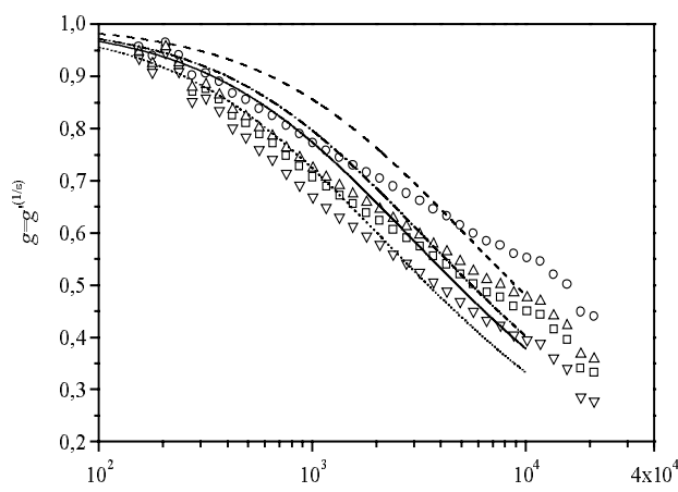
Fig. 4.5-6: Doppellogarithmische Auftragung des Schrumpfungparameters g' in Abhängigkeit des gewichteten Polymerisationsgrads P_{gew} für verschiedene Flory-Fox Parameter \varepsilon . Probe CM11/100. Symbole siehe Tab. 4.5-2.
