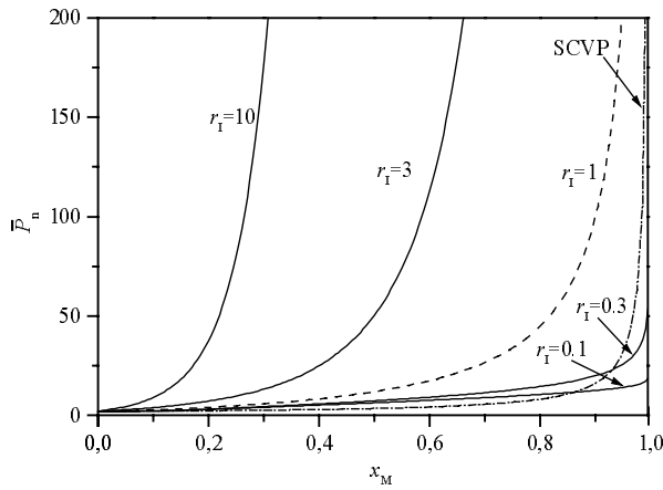
Fig. 1.2-15: Abhängigkeit des Zahlenmittels des Polymerisationsgrads vom x_M für verschiedene Reaktivitätsverhältnisse r bei \gamma = 10 . (- - -): SCVP
