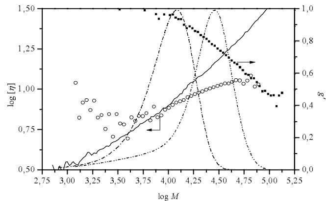
Fig. 4.5-25: Mark-Houwink Auftragung (O) und Abhängigkeit des Schrumpfungsp Parameters g' (■) vom Molekulargewicht bei der Copolymerisation von MMA mit MTSHEMA im Semibatch RI-Signal: (- · - · -) mit monofunktionalen PMMA Precursor RI-Signal: (· · · · ·). Zum Vergleich (—): intrinsische Viskosität von linearem PMMA
