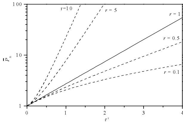
Fig. 1.2-5: Halblogarithmische Auftragung des Zahlenmittels des Polymerisationsgrads \bar{P}_n in Abhängigkeit der reduzierten Zeit \tau' für unterschiedliche r = k_A/k_B (- - -); zum Vergleich SCVP mit r = 1 (—)
