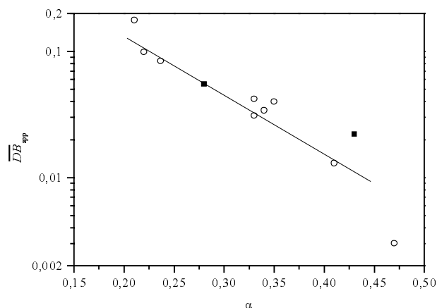
Fig. 4.5-14: Auftragung des apparenten Verzweigungsgrads \overline{DB}_{app} als Funktion des Mark-Houwink Exponenten \alpha für nichtdeuteriertes (○) und deuteriertes (■) PMMA.
