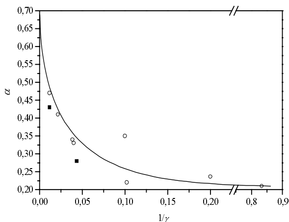
Fig. 4.5-12: Abhängigkeit des Mark-Houwink Exponenten \alpha vom reziproken Comonomerenverhältnis. (○): nichtdeuterierte Polymere (■): deuteriertes PMMA. Zum Vergleich ist für \gamma = 0 der Exponent von linearem PMMA \alpha = 0,688 dargestellt.
