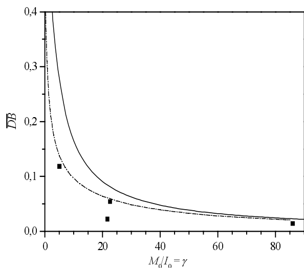
Fig. 4.3-8: Auftragung des Verzweigungsgrads \overline{DB} als Funktion von \gamma und Vergleich mit der Theorie. (■): \overline{DB} nach Tab. 4.3-5 und Tab. 4.3-7. (—): Verlauf für identische Geschwindigkeitskonstanten; (- -): Anpassung für r_1 = 1 ; \alpha = 0,1 .
