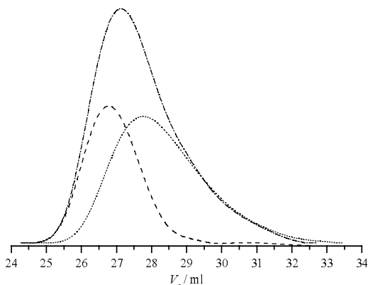
Fig. 4.5-26: Eluogramme der Synthese des Hantelmoleküls CM27. (- · - · -): RI-Signal CM27; (- - -): RI-Signal des linearen PMMA-Precursors; (· · · · ·): berechnetes RI-Signal des Hantelmoleküls nach Abzug des Precursors
