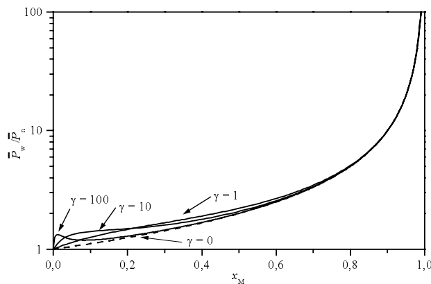
Fig. 1.2-11: Abhängigkeit des Polydispersitätsindex vom Umsatz am Monomer x_M für verschiedene Comonomerenverhältnisse \gamma
