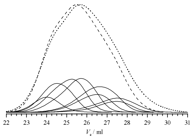
Fig. 4.6-1: Trennung des Polymers CM 12 (Feed) in einzelne Fraktionen durch präparative GPC. (—): RI-Signale der Fraktionen; (- - -): berechnetes RI-Signal des Feeds, (· · · ·): gefundenes RI-Signal des Feeds.
