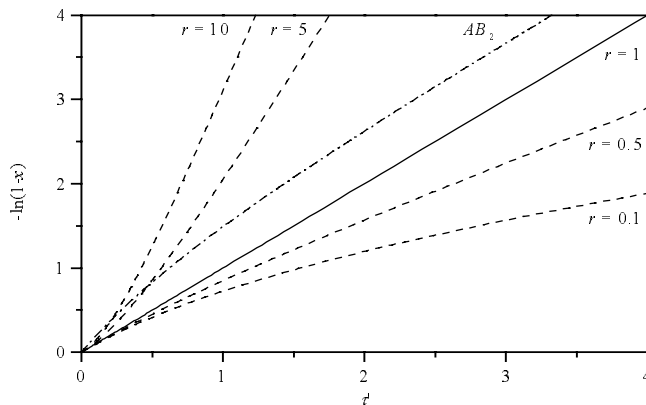
Fig. 1.2-4: Auftragung des Umsatzes an Vinyl-Gruppen x in Abhängigkeit der reduzierten Zeit \tau' = k_B I_0 t für verschieden Reaktivitätsverhältnisse r = k_A/k_B (- - -). Zum Vergleich SCVP mit r = 1 (—) und Polykondensation eines AB_2 -Monomeren (- · -)
