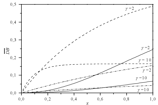
Fig. 1.2-20: Abhängigkeit des Verzweigungsgrads vom Umsatz für ein PMI (—) und für SCVCP (---). Zum Vergleich \overline{DB}_{SCVP}/(\gamma+1) (- · -).
