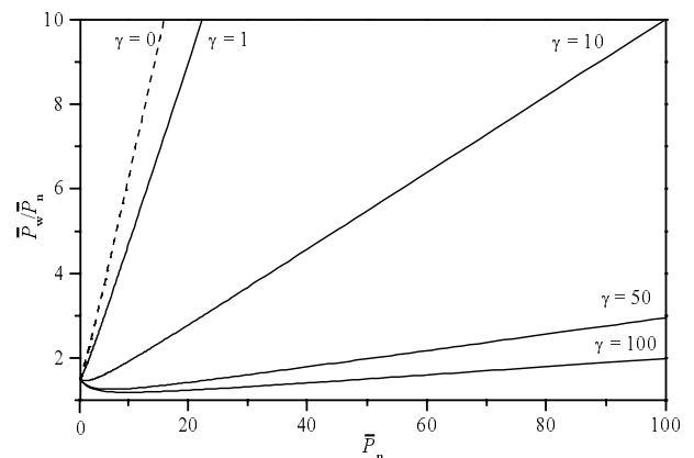
Fig. 1.2-12: Abhängigkeit des Polydispersitätsindex vom Zahlenmittel des Molekulargewichts für verschiedene Comonomerenverhältnisse \gamma
