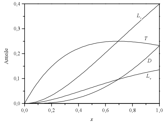
Fig. 1.2-3: Anteile struktureller Einheiten als Funktion des Umsatzes an Vinylgruppen in SCVP (vgl. Tab. 1.2-2)
