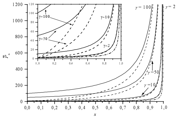
Fig. 1.2-18: Abhängigkeit des Zahlenmittels des Polymerisationsgrads vom Umsatz für die SCVCP, ein PMI (—), für die SCVCP (---), und für die SCVCP (- · -)
