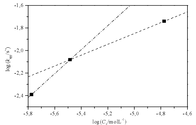
Fig. 4.2-2: Bestimmung der Reaktionsordnung bezüglich der Katalysatorkonzentration C_0 für das GTP–System MTSHEMA/MMA/TBABB in THF.
