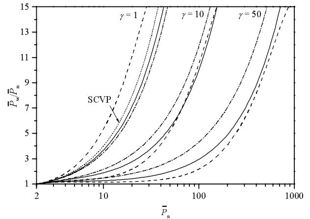
Fig. 1.2-16: Auftragung des Polydispersitätsindex als Funktion des Zahlenmittels für unterschiedliche Reaktivitätsverhältnisse. (- - -): r_I = 0,3 ; (—): r_I = 1 ; (- · - · -): r_I = 3 .
