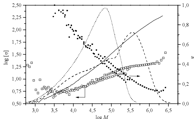
Fig. 4.5-18: intrinsische Viskosität (O, □), Schrumpfungparameter (■, ●) und RI-Signale (· · · ·, - - -) der Copolymerisation von MTSHEMA mit MMA 8 unter Semibatch- und Batchbedingungen ( I_0 = 1,5 \cdot 10^{-2} \text{ molL}^{-1} ; \gamma = 22 ; \chi = 700 , TBABB). Symbole siehe Tab. 4.5-5. (—): intrinsische Viskosität von linearem PMMA
