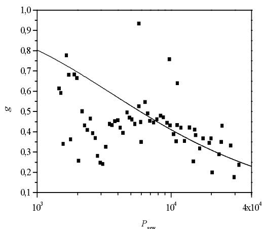
Fig. 4.5-4 Auftragung des Schrumpfungparameters g in Abhängigkeit des gewichteten Polymerisationsgrads P_{gew} (vgl. Gleichung (4.3-10) zur Ermittlung der Anzahl der tatsächlich eingebauten Verzweigungen Polymer CM11/100.
