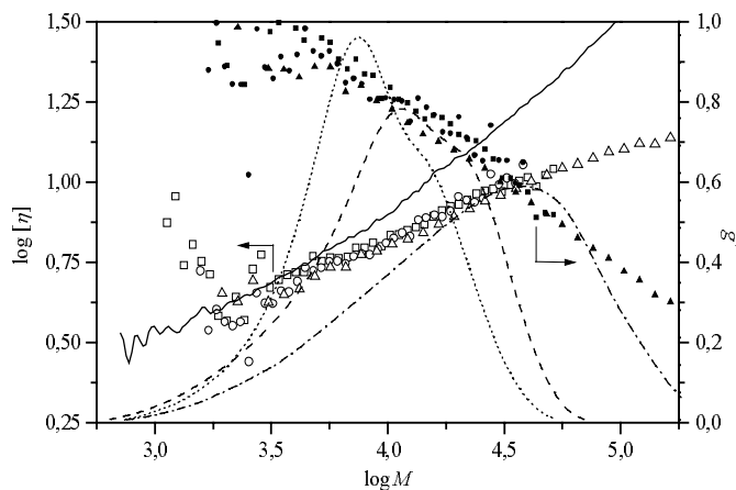
Fig. 4.5-23: Mark-Houwink Auftragung ( \square, \circ, \triangle ) und Abhängigkeit des Schrumpfungparameters g' ( \blacksquare, \bullet, \blacktriangle ) der Copolymerisation von MMA mit MTSHEMA im Semibatch in Gegenwart von MTS für verschiedene Initiatorfunktionalitäten f . Linientypen des RI-Signals und Symbole siehe Tab. 4.5-7. (—): intrinsische Viskosität von linearem PMMA.
