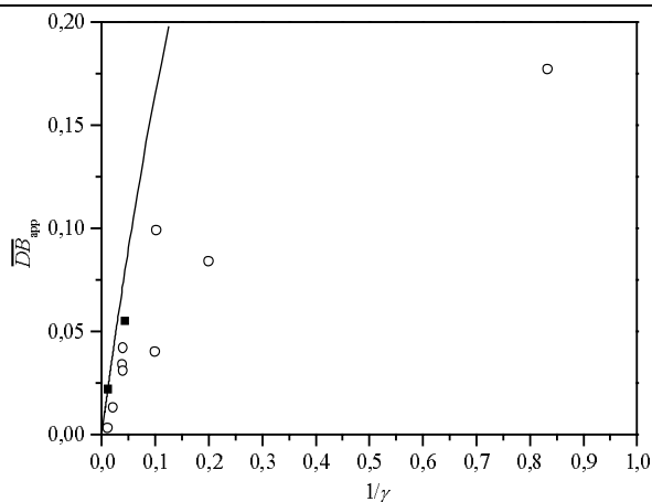
Fig. 4.5-13: Zusammenhang zwischen apparenten Verzweigungsgrad und reziproken Comonomerenverhältnis für nichtdeuteriertes (○) und deuteriertes (■) Polymer; (—): Theorie nach Gleichung (1.2-30); (- - -): Ausgleich für \overline{DB} = 1/\gamma .
