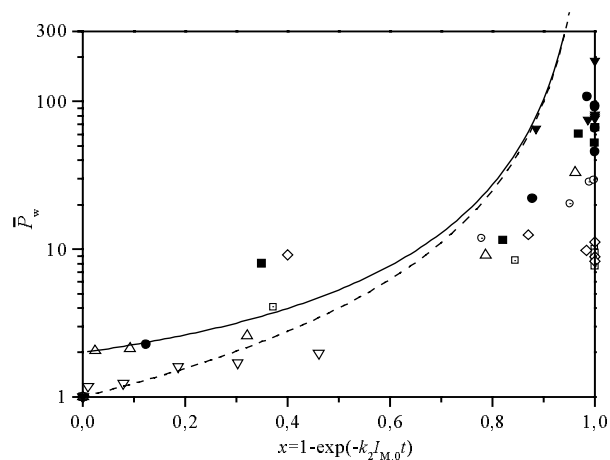
Fig. 4.1-9: Auftragung des Massenmittel des Polymerisationsgrads als Funktion des Umsatzes an Doppelbindungen x . (□): H10 und (⊙): H16; vgl. Tab. 4.1-3; (■): H II, (●): H III und (▼): H IV; (△): H11 (▽): H12 (◇): H13, vgl. Tab. 4.1-4 Theorie für ideale SCVP (—).
