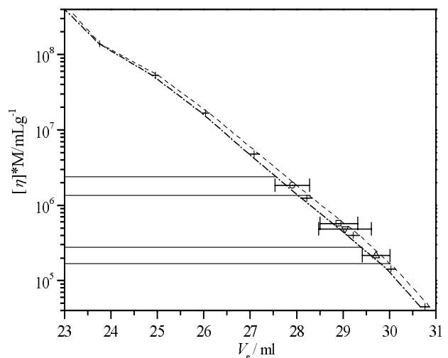
Fig. 4.7-4: Ergebnisse der wässrigen GPC-Messung. Universelle Kalibrationskurve für Pullulane (+) bei Flüssen von 1 ml/min (- - -) und 0,5 ml/min (- - -). Die offenen Symbole (vgl. Tab. 4.7-2) gegeben den Mittelwert des bei \dot{V} = 1 ml/min und \dot{V} = 0,5 ml/min bestimmten Peakmaximums der verzweigten Polymethacrylsäuren an.
