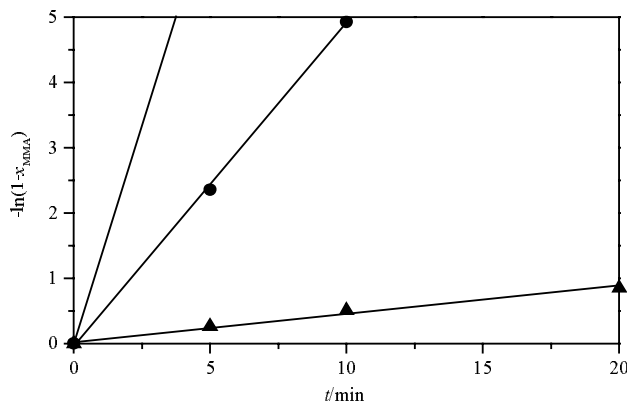
Fig. 4.2-4: Zeit-Umsatz-Auftragung für unterschiedliche Absolutkonzentration an Comonomeren. Katalysator TBABB, \gamma = 25 ; \chi = 2600 ; Raumtemperatur. Das Erreichen des vollständigen Umsatzes bei Versuch CM21M8 nach t = 5 min wird durch die durchgezogene Linie angedeutet. Übrige Symbole und Ergebnisse siehe Tab. 4.2-2.
