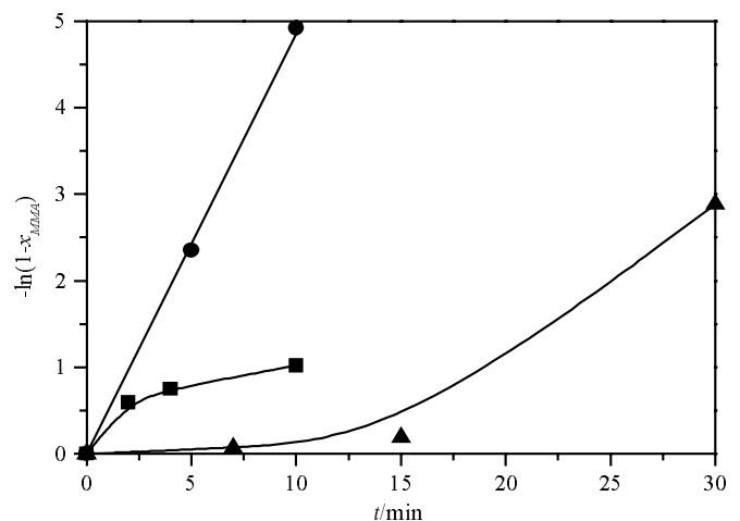
Fig. 4.2-7: Zeit-Umsatz-Auftragung für Katalyse mit TBAB3CIB (▲), TASHF 2 (■) und TBABB (●). Alle Versuche \gamma = 25 , bzw. \chi = 2500 ( I_0 = 8,41 \cdot 10^{-3} \text{ molL}^{-1} ; C_0 = 3,22 \cdot 10^{-6} \text{ molL}^{-1} 293 K.
