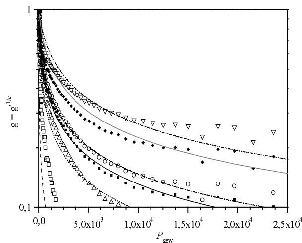
Fig. 4.3-13: Auftragung des nach (4.3-14) aus g' berechneten Schrumpfungsfaktors g als Funktion des gewichteten Polymerisationsgrads P_{\text{gew}} zur Bestimmung des Anteils an Verzweigungspunkten für verschiedene \varepsilon . Polymer CM32. Symbole und Linientypen siehe Tab. 4.3-8
