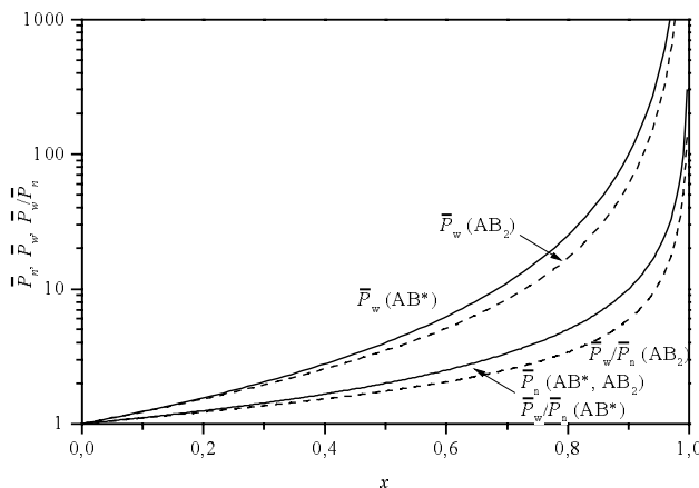
Fig. 1.2-1: Auftragung der Mittelwerte des Molekulargewichts und des Polydispersitätsindex in Abhängigkeit vom Umsatz x an Doppelbindungen für SCVP (—) und AB_2 -Kondensation (---)
