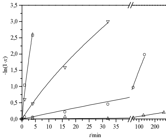
Fig. 4.1-3: Zeit-Umsatz-Auftragung erster Ordnung der Homopolymerisation von MTSHEMA unter Katalyse von TBAB3CIB bei Variation der Temperatur. Reaktionsbedingungen und Symbole siehe Tab. 4.1-2
