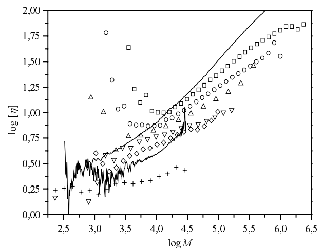
Fig. 4.5-2: Mark-Houwink Auftragung für verschiedene Comonomerenverhältnisse \gamma . (—): lineares PMMA; (---): lineares PIBHEMA. Symbole siehe Tab. 4.5-1
