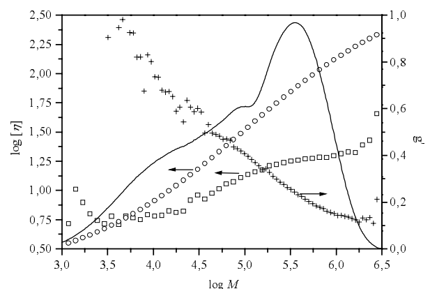
Fig. 4.3-10 Auftragung der intrinsischen Viskosität [\eta] von verzweigtem ( \square ) und linearem ( \circ ) PMMA und des Schrumpfungsparmeters (+) in Abhängigkeit des Molekulargewichts (—): RI-Signal.
