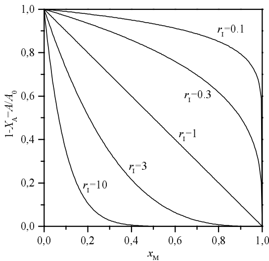
Fig. 1.2-14: Abhängigkeit des Umsatzes an Vinylgruppen des A vom Umsatz an Monomer x_M für SCVCP und verschiedene Reaktivitätsverhältnisse
