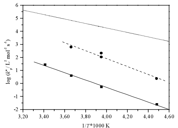
Fig. 4.1-5: Arrhenius-Auftragung für die mit TBAB3ClB (—■—) und mit TBABB (-●-) katalysierte SCVP von MTSHEMA. Zum Vergleich MTS initiierte Homopolymerisation von MMA unter Katalyse von TBABB (····) nach Gores. 248
