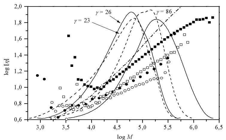
Fig. 4.5-9: Vergleich der intrinsischen Viskosität der nichtdeuterierten Proben CM11/100 ( \gamma = 86 , ■) und CM12 ( \gamma = 26 , ●), RI-Signal (—) mit den deuterierten Proben CM31 ( \gamma = 86 , □) und CM30 ( \gamma = 23 , ○) RI-Signal (- - -). Viskosität von linearem PMMA (- · - · -)
