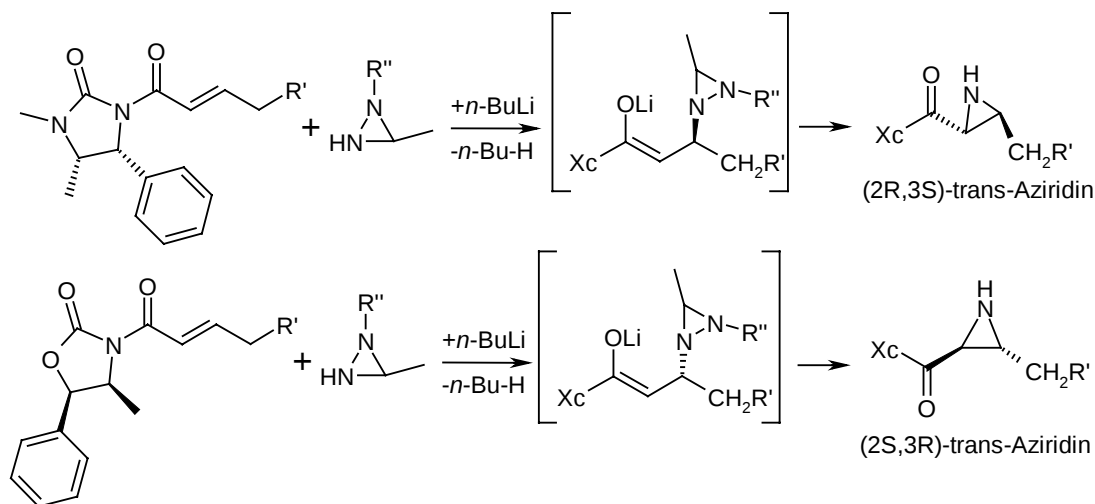
Schema 39 (bevorzugter Angriff oben von der si-Seite, unten von der re-Seite)
