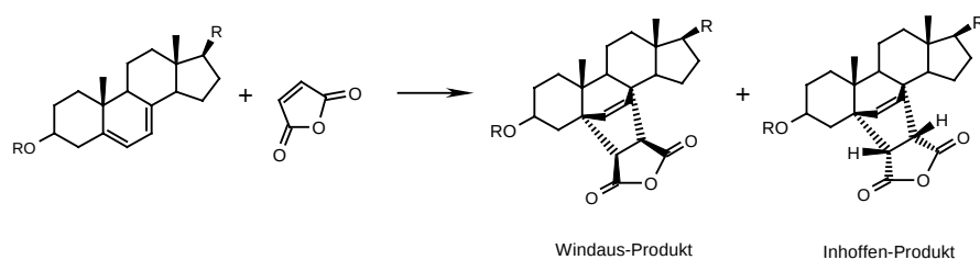
Schema 178 Windaus-Addukt, Inhoffen-Addukt
