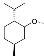
Menthol-(Ester-)Derivat
