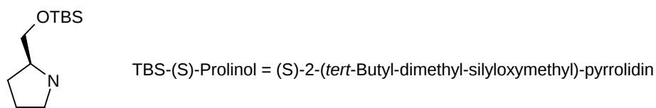
Bild 4 (Prolinol-Auxiliar)
