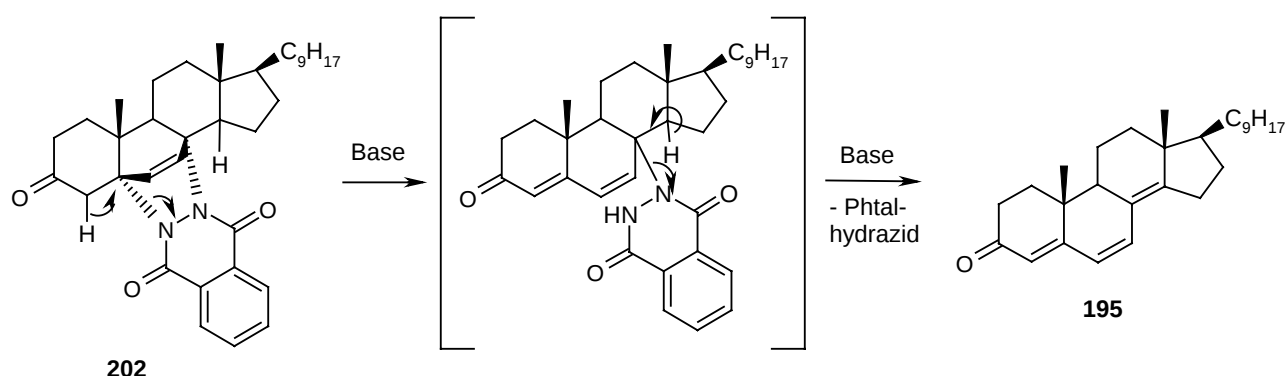
Bild 33 β-Eliminierung in 3-Oxo-5,8-phthalazindiono-ergosterolderivaten
