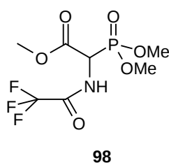
Bild 7 Trifluoracetyl-geschütztes Glycinphosphonat 98
