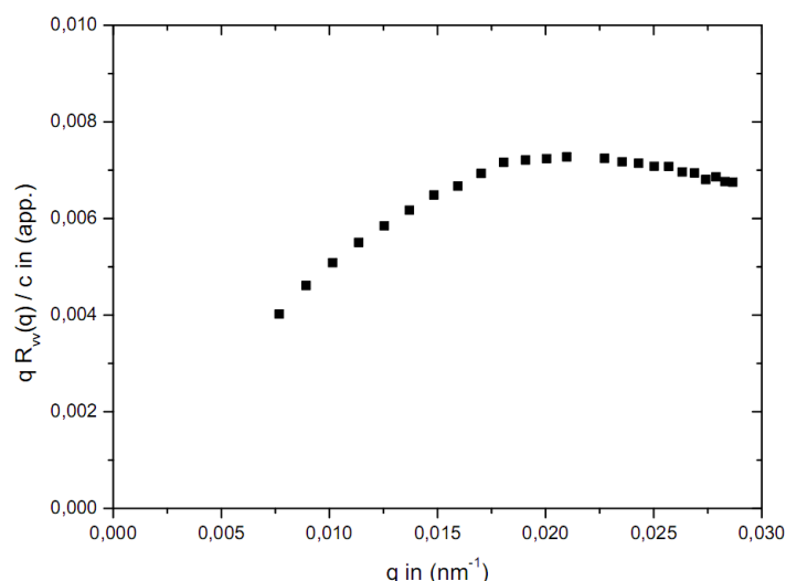
Abb. 2.16: Holtzer-Auftragung der Probe ZnO-6 .
