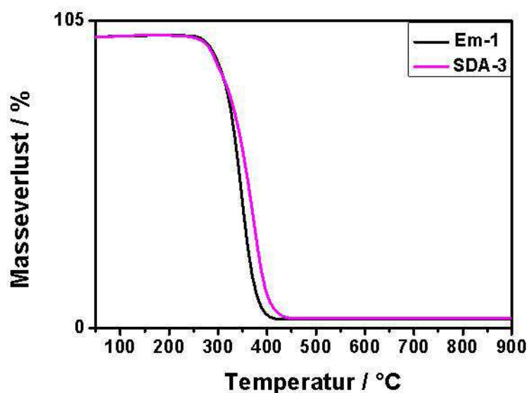
Abb. 4.8: Ergebnisse der TGA der Polymere Em-1 und SDA-3 .
