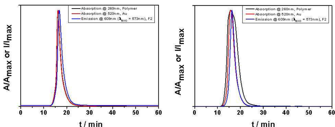
Abb. 8.37: GPC-Kurven der Partikel Au1(+)-F2 (links) und Au1(-)-F2 (rechts). Daten AK Parak.
