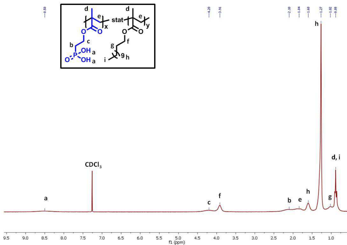
Abb. 8.7: ^1\text{H} -NMR-Spektrum von CN2(-) in \text{CDCl}_3 .
