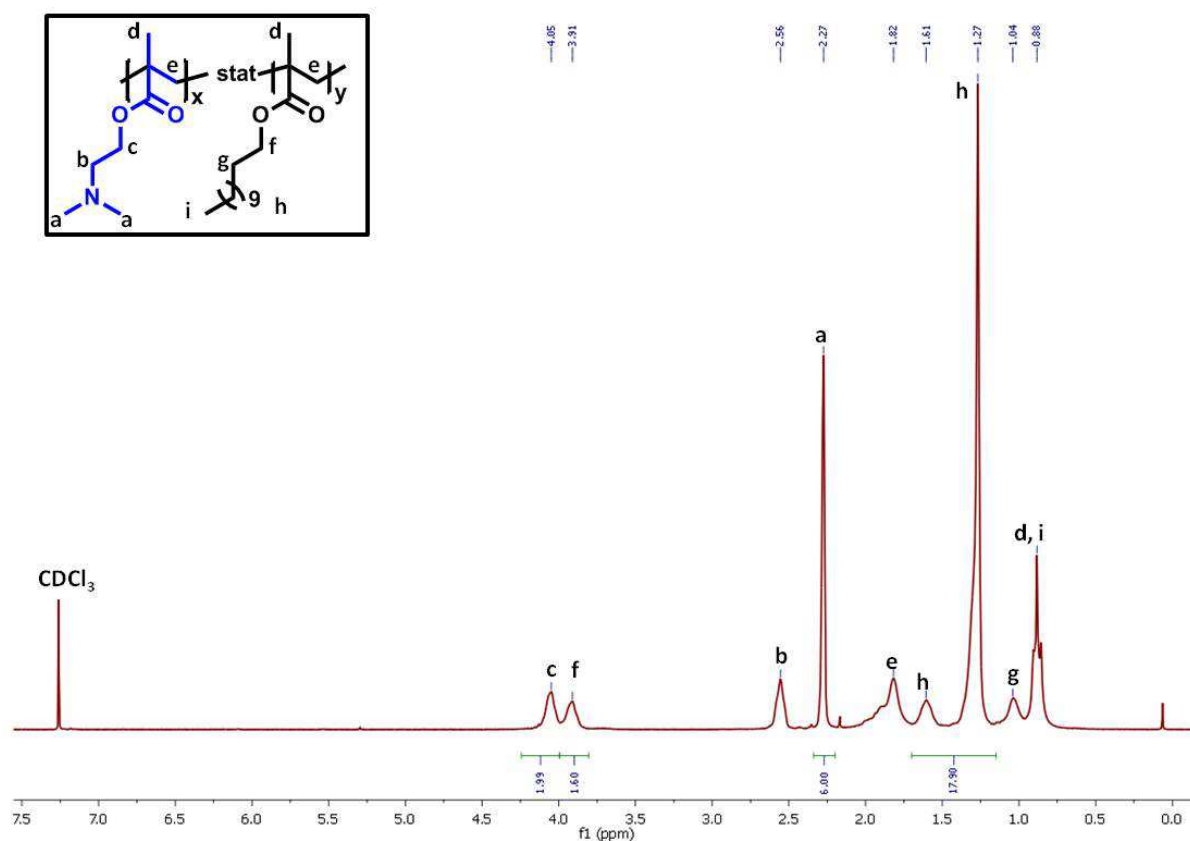
Abb. 8.2: ^1\text{H} -NMR-Spektrum von CP4 in \text{CDCl}_3 .
