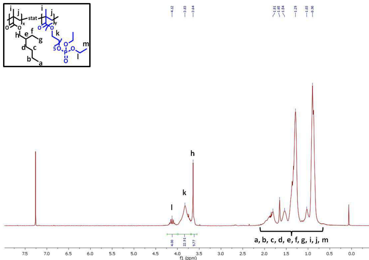
Abb. 2.4: ^1\text{H} -NMR-Spektrum von PEHMA- stat -PDPEOMA-2.
