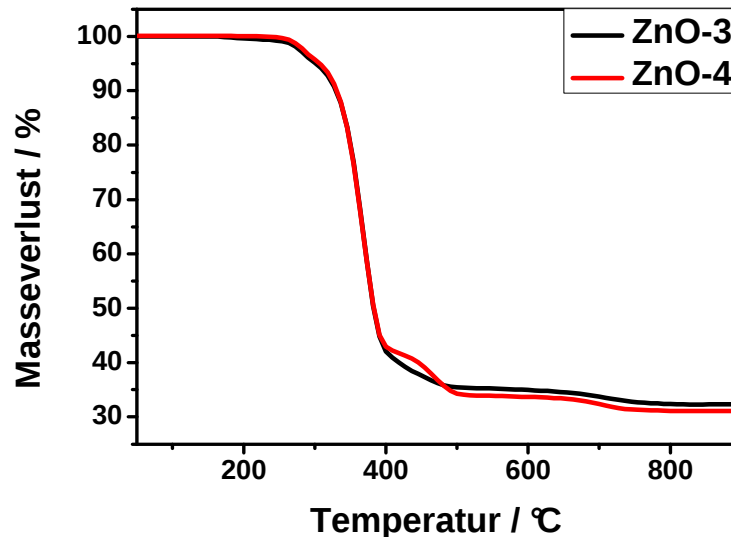
Abb. 2.11: Thermogravimetrische Untersuchung der in-situ hydrophobierten Partikel der Proben ZnO-3 und ZnO-4 .
