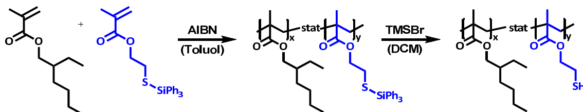
Abb. 3.6: Synthese von Em2 bis Em4 .
