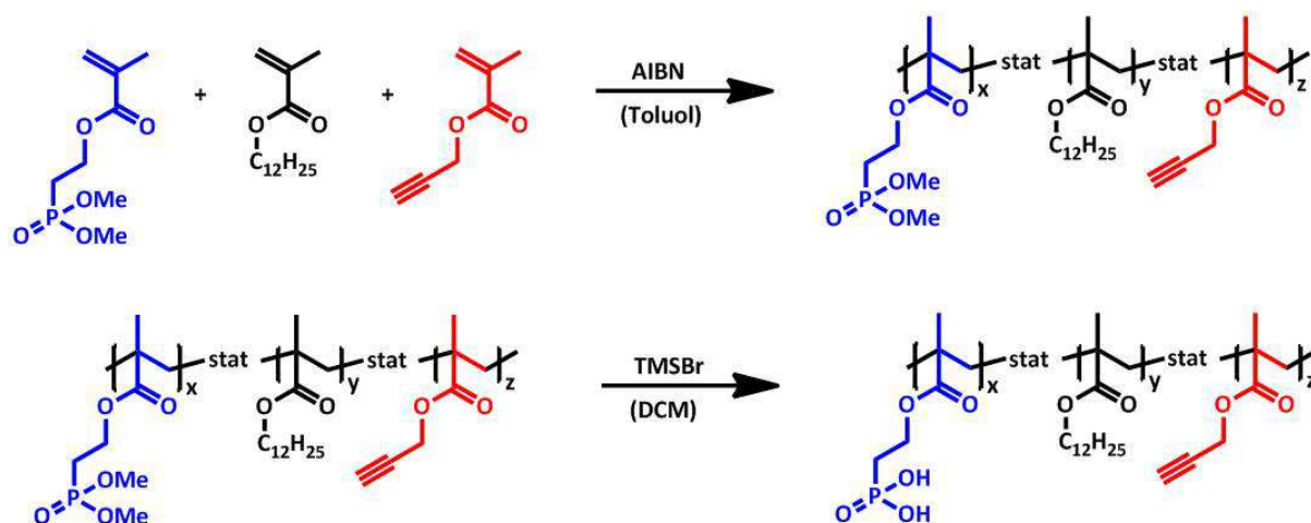
Abb. 8.24: Synthese von TN1(-) bis TN5(-) durch freie radikalische Terpolymerisation von LMA, MAPHOS(OMe) 2 und PgMA mit anschließendem Entschützen zur freien Säure.
