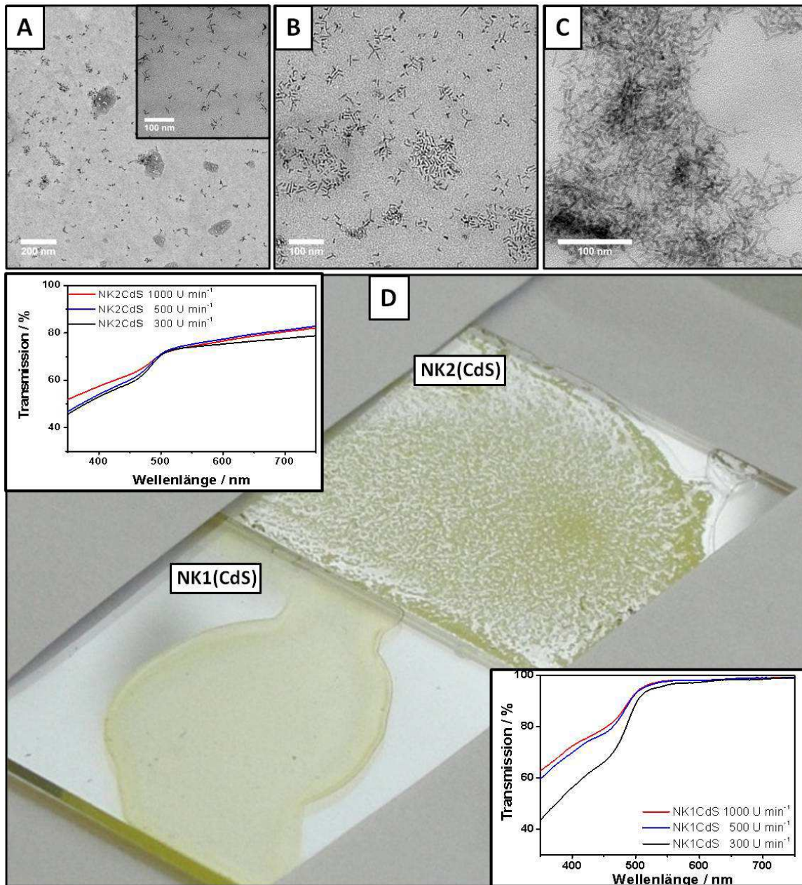
Abb. 5.2: a) TEM-Bild von NK1(CdS) 1000 U min -1 b) TEM-Bild von NK1(CdS) 300 U min -1 c) TEM-Bild von NK2(CdS) 300 U min -1 d) UV-Vis-Spektren von NK1(CdS) und NK2(CdS) sowie digitale Fotos von NK1(CdS) 300 U min -1 und NK2(CdS) 300 U min -1 .
