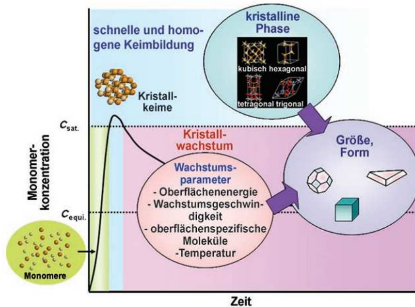
Abb. 1.3: Schematische Darstellung der Kristallisation anorganischer Nanopartikel. C_{\text{sat}} = Sättigungskonzentration, C_{\text{equi}} = Gleichgewichtskonzentration. Abbildung aus [41].
