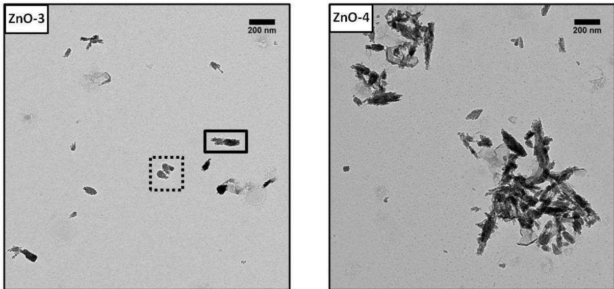
Abb. 2.9: TEM-Aufnahmen der in Toluol redispersierten Partikel der Proben ZnO-3 und ZnO-4 .
