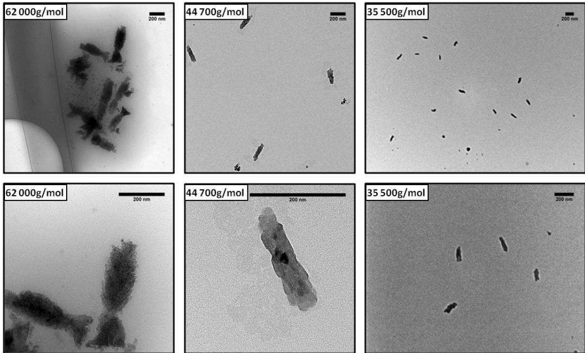
Abb. 2.18: TEM-Aufnahmen der in Toluol redispergierten Partikel der Proben ZnO-7 , ZnO-9 und ZnO-10 .
