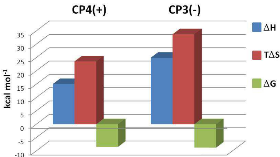
Abb. 8.16: Thermodynamische Profile der Wechselwirkungen zwischen den Copolymeren CP4(+) bzw. CP3(-) und den hydrophoben Au-Nanopartikeln.
