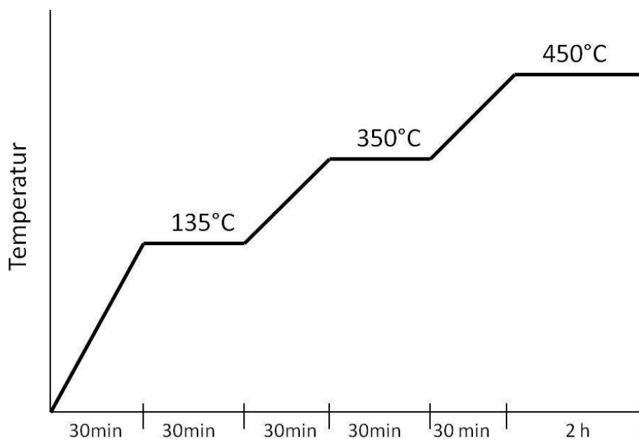
Abb. 6.6: Temperaturprogramm für das Sintern der \text{TiO}_2 -Nanopartikel.
