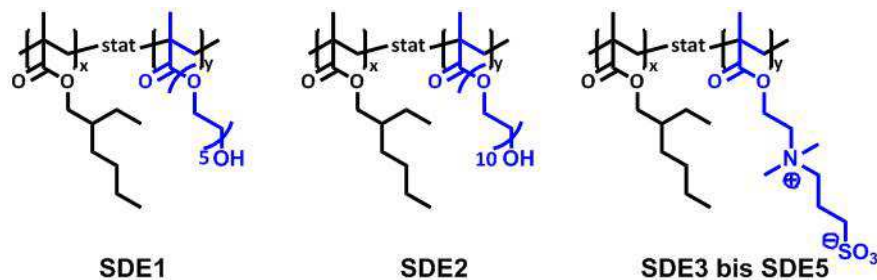
Abb. 6.3: Die für die Darstellung poröser \text{TiO}_2 -Nanopartikel verwendeten SDE1 bis SDE5 .
