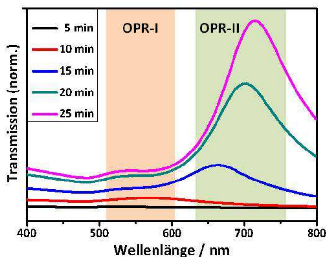
Abb. 3.4: Darstellung der UV-Vis-Spektren der Probe Au-9 während der Reaktion.
