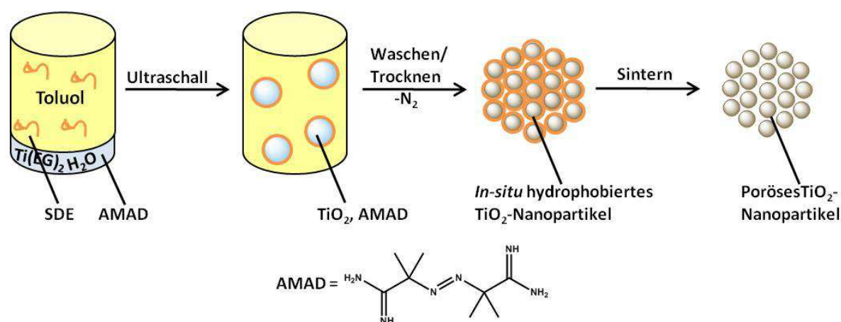
Abb. 6.10: Reaktionsschema zur Darstellung poröser \text{TiO}_2 -Nanopartikel über das inverse Emulsionsverfahren unter Zugabe von AMAD.
