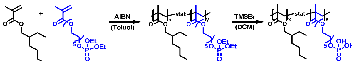
Abb. 2.3: Synthese von PEHMA- stat -PPPEOMA.
