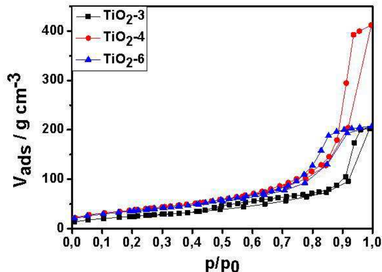
Abb. 6.13: Stickstoff-Sorptionen der gesinterten Proben TiO 2 -3 , TiO 2 -4 und TiO 2 -6 .
