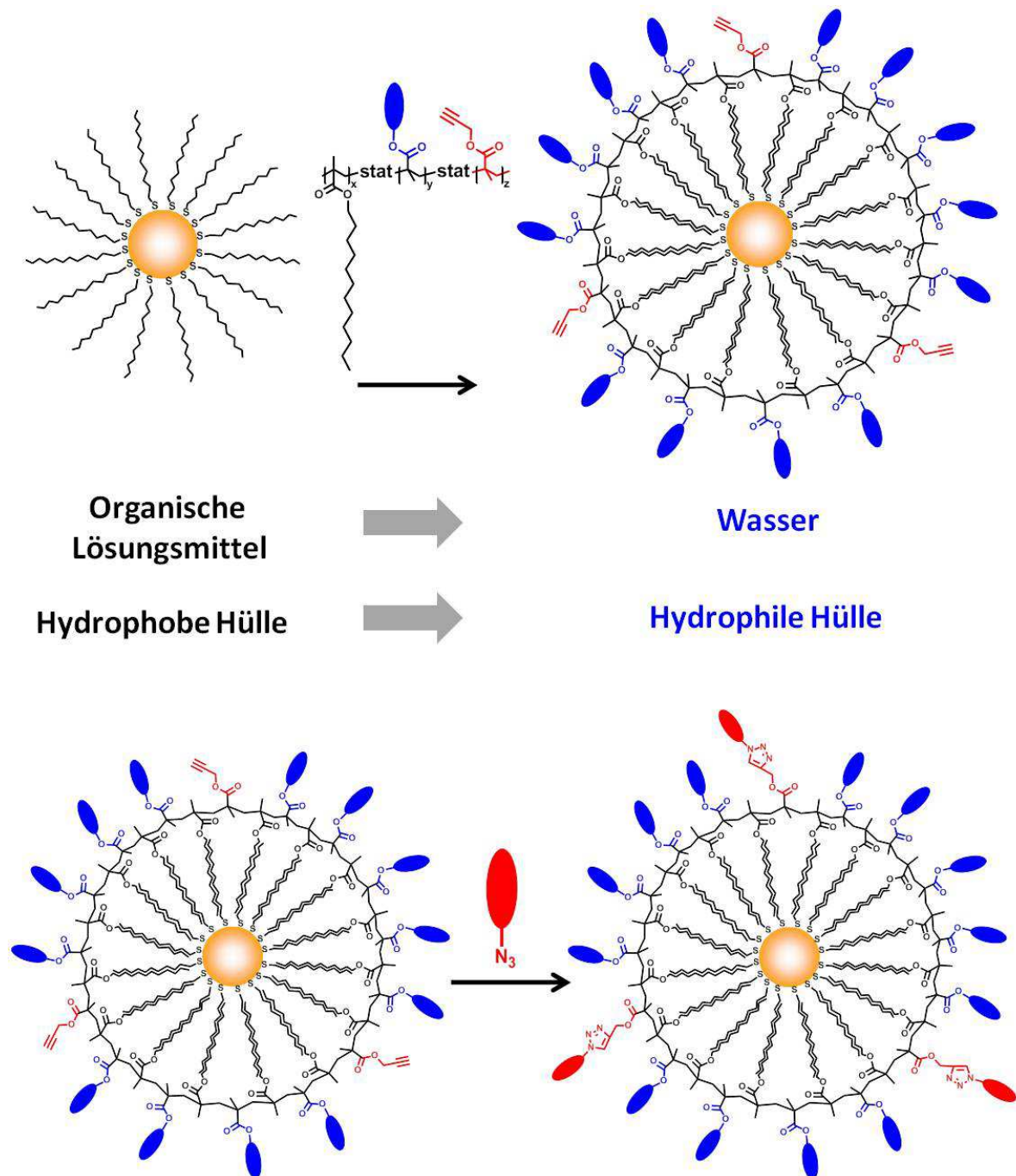
Abb. 8.21: Schematische Abbildung der Hydrophilierung anorganischer Nanopartikel mit amphiphilen, statistischen Terpolymeren und anschließender Postfunktionalisierung.
