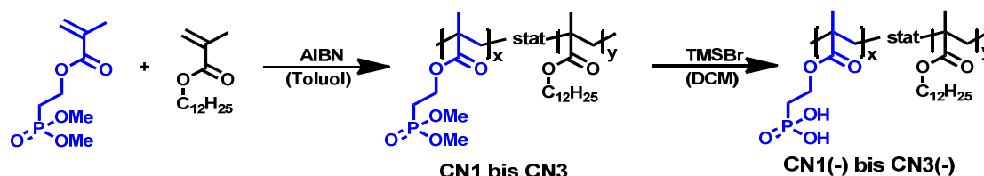
Abb. 8.5: Synthese von CN1(-) bis CN3(-) über freie radikalische Copolymerisation von LMA und MAPHOS(OMe) 2 mit anschließender Entschüttung zur freien Säure.
