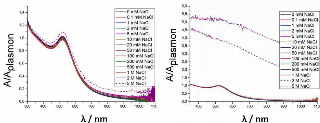
Abb. 8.15: UV-Vis-Spektren der Partikel Au4(+) (links) bzw. Au3(-) (rechts) in Salzlösungen verschiedener Konzentrationen. Daten von AK Parak.
