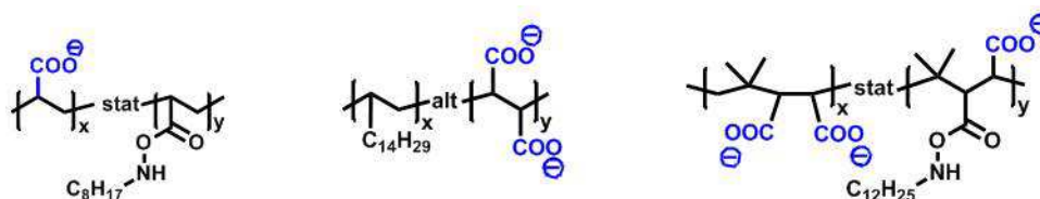
Abb. 1.7: Zur Hydrophilierung anorganischer Nanopartikel verwendete Copolymere.
