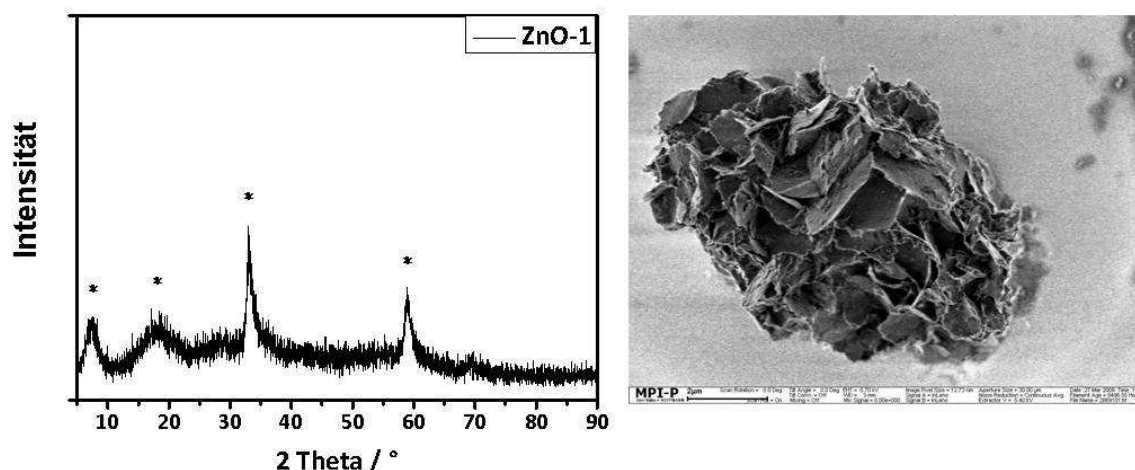
Abb. 2.7: Pulverdiffraktogramm (links) und REM-Aufnahme eines redispersierten Partikels der Probe ZnO-1 (rechts).
