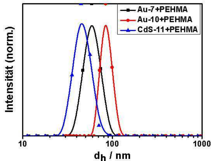
Abb. 5.1: Mittels DLS bestimmte, ungewichtete Durchmesser-Verteilung (Winkel von 90°) der Partikel Au-7 , Au-10 und CdS-11 in einer Toluol-PEHMA-Lösung.
