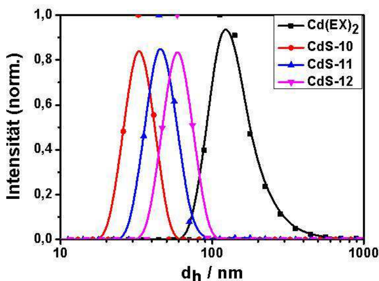
Abb. 4.11: Mittels DLS bestimmte, ungewichtete Durchmesser-Verteilung der Partikel Cd(EX) 2 , CdS-10 bis CdS-12 bei einem Winkel von 90°.
