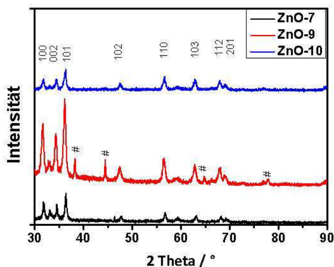
Abb. 2.17: Pulverdiffraktogramme der Proben ZnO-7 , ZnO-9 und ZnO-10 . # ... Signale des Al-Probenhalters.
