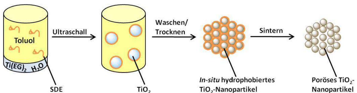
Abb. 6.5: Reaktionsschema zur Darstellung poröser TiO 2 -Nanopartikel über das inverse Emulsionsverfahren.
