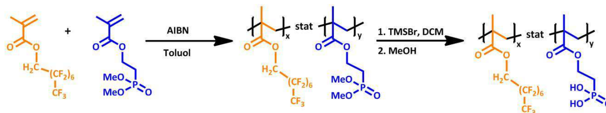
Abb. 7.9: Synthese von CP-MAPHOS.
