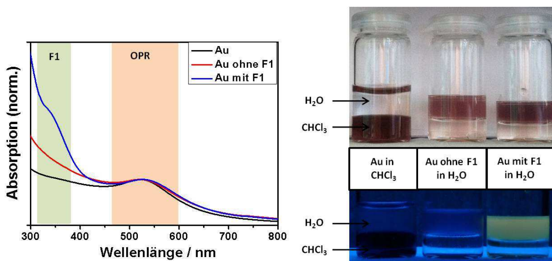
Abb. 8.28: UV-Vis Spektren (a) und Fotos der Au-Nanopartikel (b) während bzw. nach der Postfunktionalisierung.
