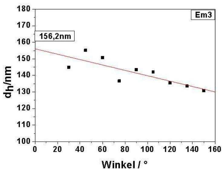
Abb. 3.9: Grafische Darstellung der Ergebnisse der DLS-Experimente von Em3 .
