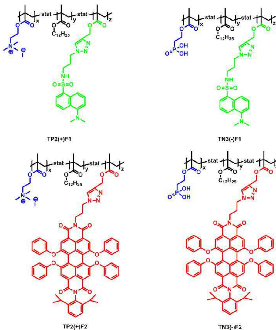
Abb. 8.33: Dargestellte farbstofffunktionalisierte Terpolymere TP2(+)-F1 , TP2(+)-F2 , TN3(-)-F1 und TN3(-)-F2 .
