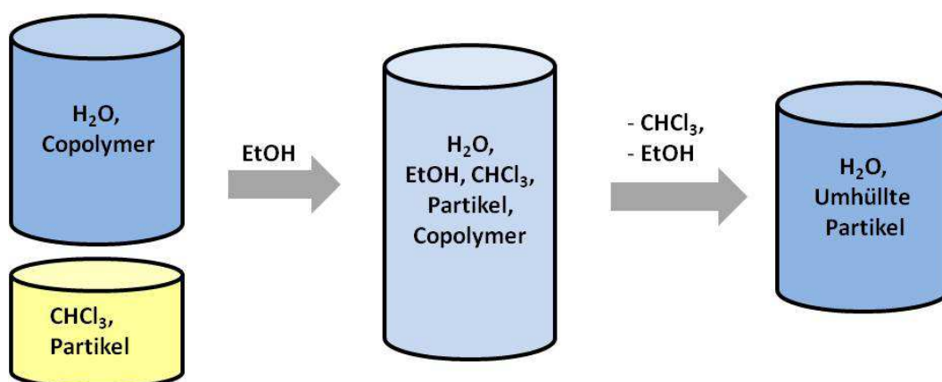
Abb. 8.11: Schematische Darstellung des Umhüllungsprozesses für hochgeladene nur in Wasser lösliche Copolymere.
