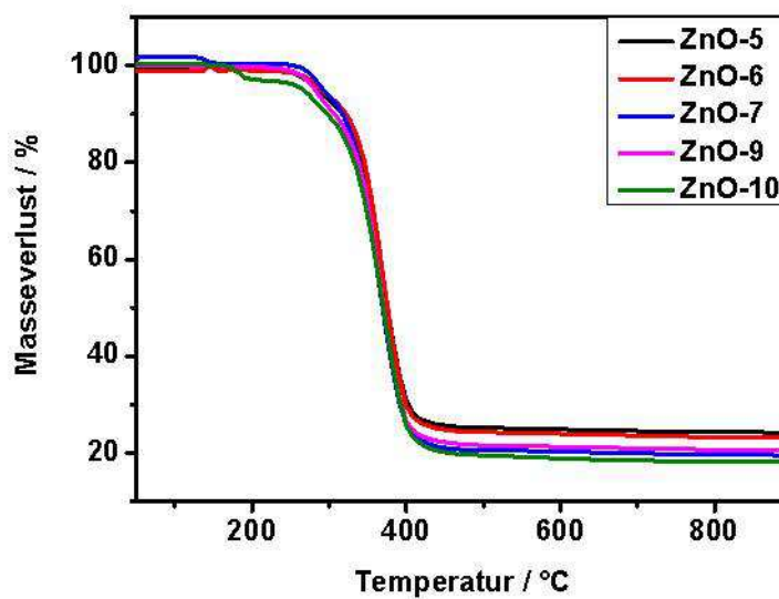
Abb. 2.21: Thermogravimetrische Untersuchung der in-situ hydrophobierten Partikel der Proben ZnO-5 , ZnO-6 , ZnO-7 , ZnO-9 und ZnO-10 .
