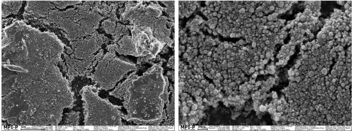
Abb. 6.14: REM-Aufnahmen von \text{TiO}_2 -Film4. nach dem Sintern.
