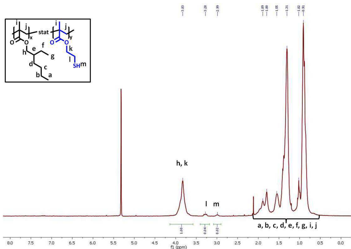
Abb. 3.8: ^1\text{H} -NMR-Spektrum von Em3 .
