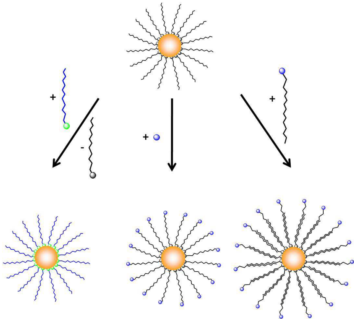
Abb. 1.6: Verschiedene Methoden zur Hydrophilierung anorganischer Nanopartikel.
