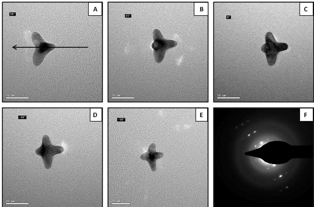
Abb. 3.3: TEM-Bilder eines verzweigten, in-situ hydrophobierten Gold-Nanopartikels mit 4 Spitzen der Probe Au-9 , welches um verschiedene Winkel in Pfeilrichtung gekippt wurde. (A) 50°, (B) 15°, (C) 0°, (D) -10°, (E) -50° und (F) Elektronenbeugung eines Bereiches des Partikels.
