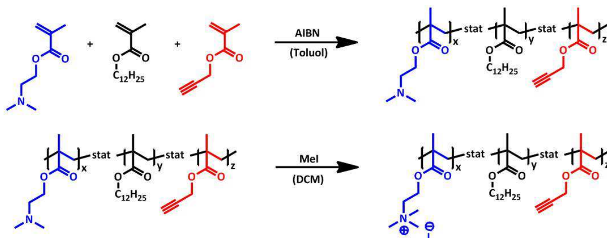
Abb. 8.22: Synthese von TP1(+) und TP2(+) durch freie radikalische Terpolymerisation von LMA, DMAEMA und PgMA mit anschließender Quaternisierung der Aminogruppen.
