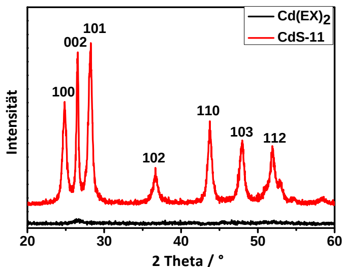
Abb. 4.9: Pulverdiffraktogramme der Partikel Cd(EX) 2 und CdS-11 .
