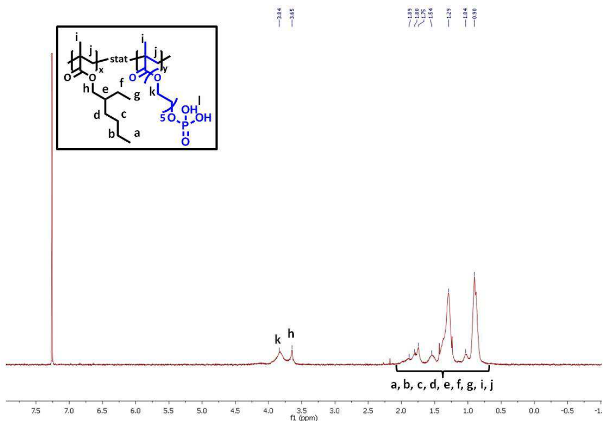
Abb. 2.5: ^1\text{H} -NMR-Spektrum von PEHMA-stat-PPPEOMA-2.
