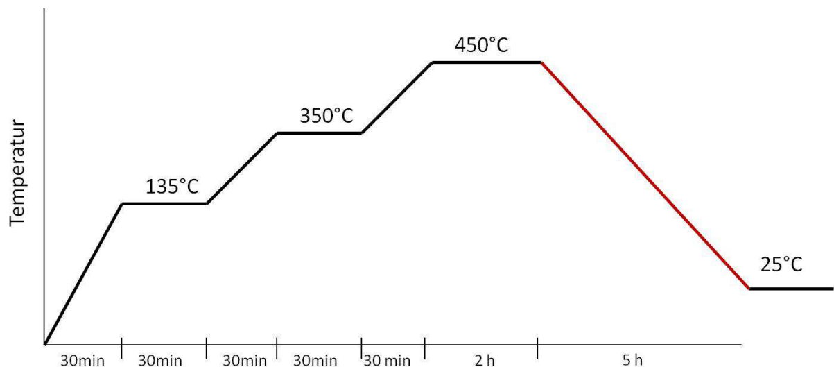
Abb. 6.15: Verändertes Temperaturprogramm zum Sintern der \text{TiO}_2 -Partikel.
