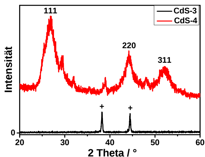
Abb. 4.2: Pulverdiffraktogramm der Proben CdS-3 und CdS-4 .
