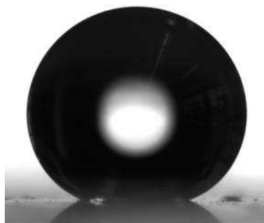
Abb. 7.8: Kontaktwinkelmessung: Wassertropfen auf mit CP-PEOMA1 fluorophilierten SiO 2 -Oberflächen.
