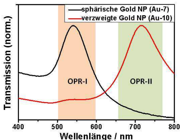
Abb. 3.10: Darstellung der UV-Vis-Spektren der Probe Au-7 und Au-10 während der Reaktion.
