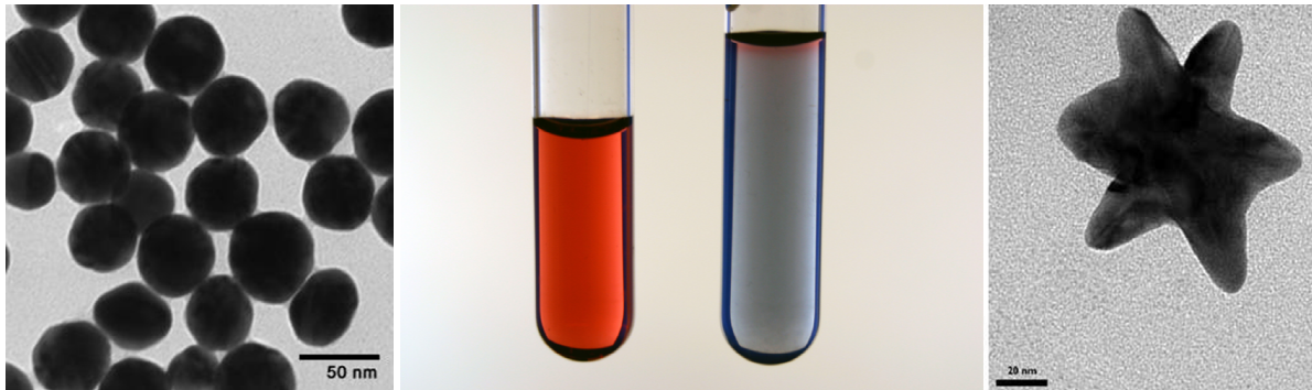
Abb. 1.2: Wässrige Dispersionen von sphärischen (links) und verzweigten (rechts) Au-Nanopartikeln sowie zugehörige TEM-Bilder. [14]
