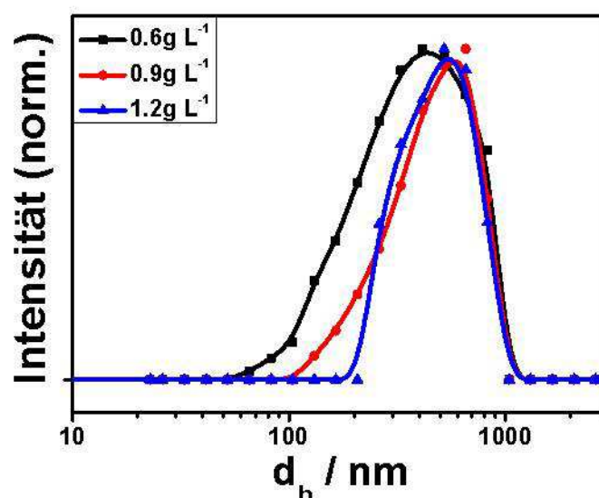
Abb. 2.15: Mittels DLS bestimmte, ungewichtete Durchmesser-Verteilung der Proben ZnO-5 , ZnO-6 und ZnO-7 bei einem Winkel von 90^\circ .
