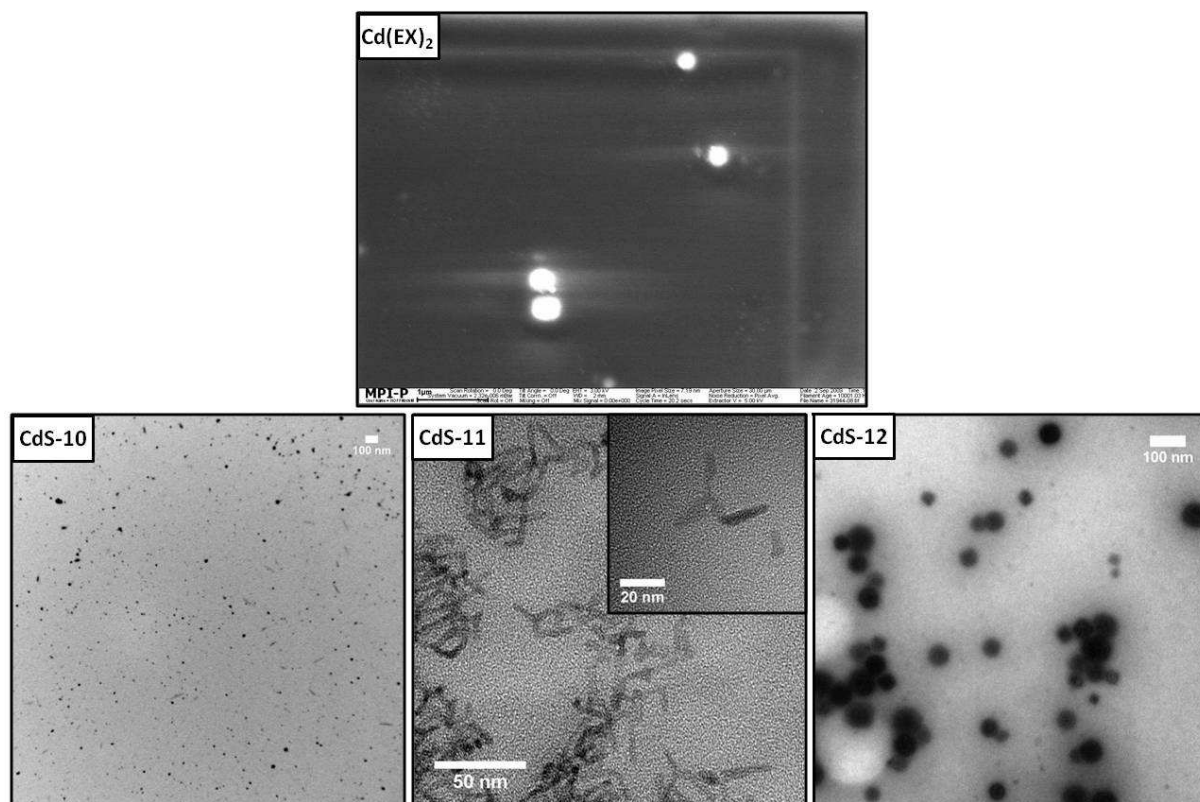
Abb. 4.10: Elektronenmikroskopische Aufnahmen der Partikel Cd(EX) 2 , CdS-10 , CdS-11 und CdS-12 .
