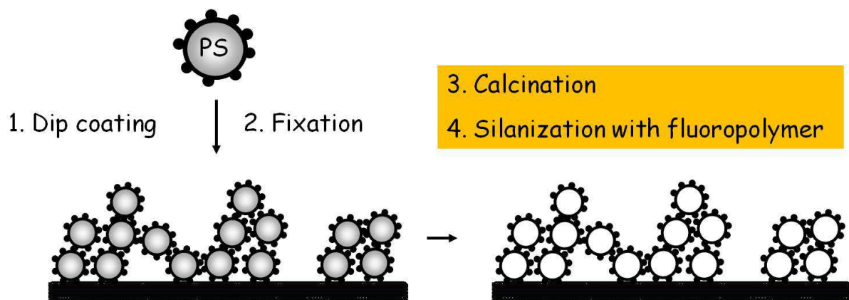
Abb. 7.5: Darstellung der superhydrophoben Oberflächen.
