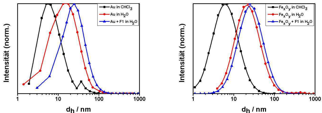
Abb. 8.30: Über DLS bestimmte, ungewichtete Durchmesser-Verteilung, gemessen bei 90 °, der Au- und \text{Fe}_x\text{O}_y -Nanopartikel in den 3 Etappen der Postfunktionalisierung.
