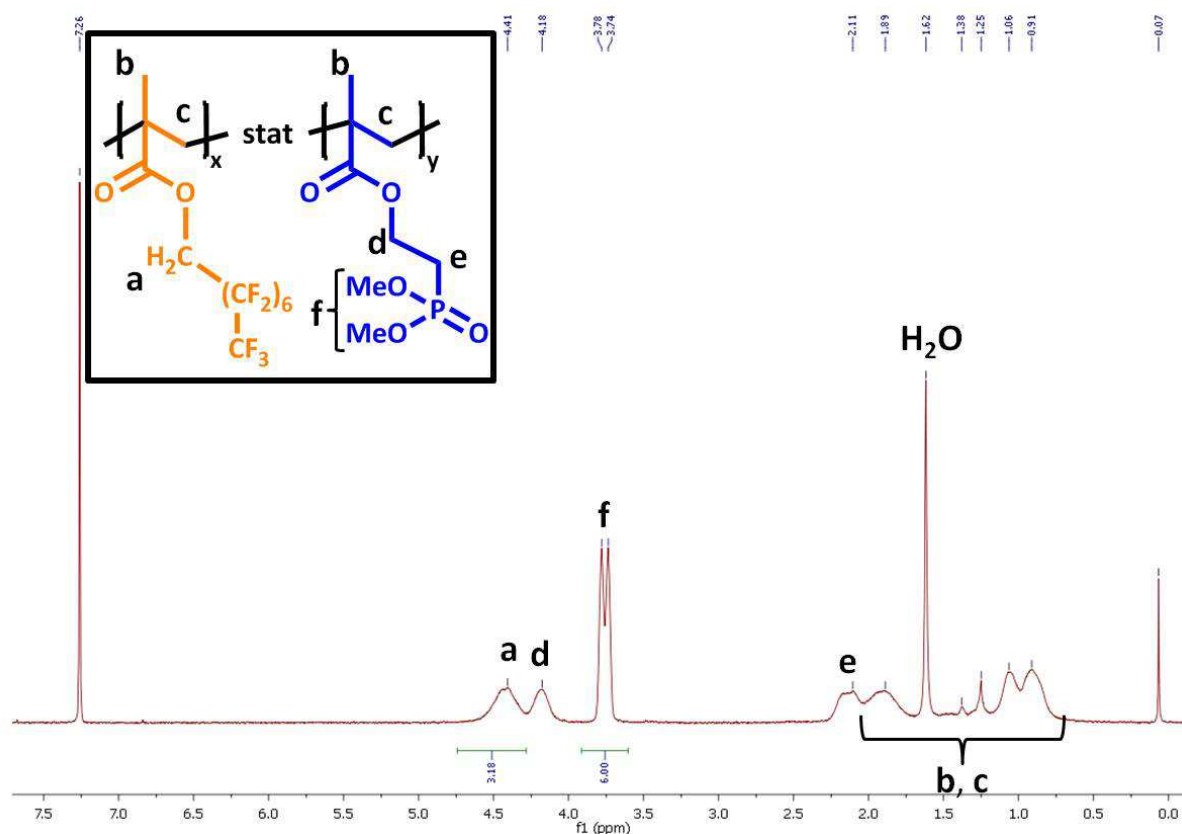
Abb. 7.10: ^1\text{H} -NMR-Spektrum des geschützten CP-MAPHOS1.
