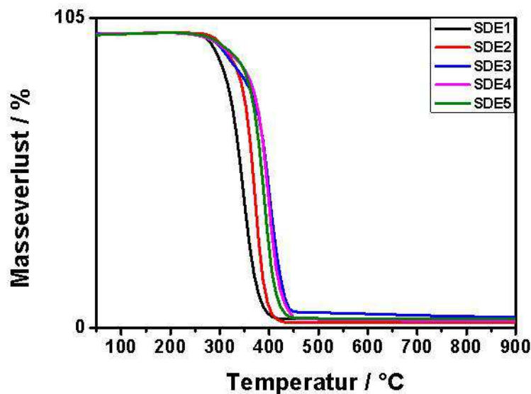
Abb. 6.4: TGA der Emulgatoren SDE1 bis SDE5 .
