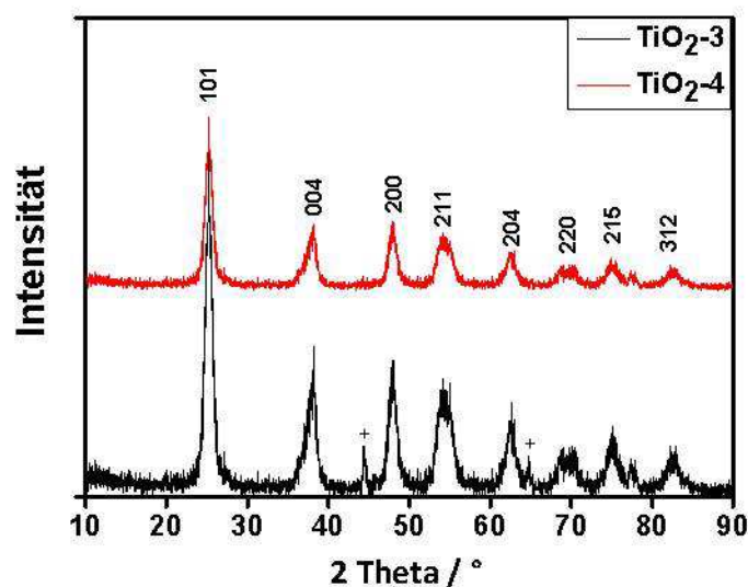
Abb. 6.11: Pulverdiffraktogramme der Probe TiO 2 -3 und TiO 2 -4 .
