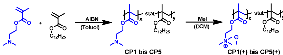
Abb. 8.1: Synthese von CP1(+) bis CP5(+) über freie radikalische Copolymerisation von LMA und DMAEMA mit anschließender Quaternisierung der Aminogruppen.
