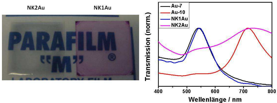
Abb. 5.2: Digitales Foto von NK1(Au)-1000 U min -1 und NK2(Au)-300 U min -1 (links) UV-Vis-Spektren von Au-7 , Au-10 , NK1(Au)-1000 U min -1 und NK2(Au)-300 U min -1 (rechts).
