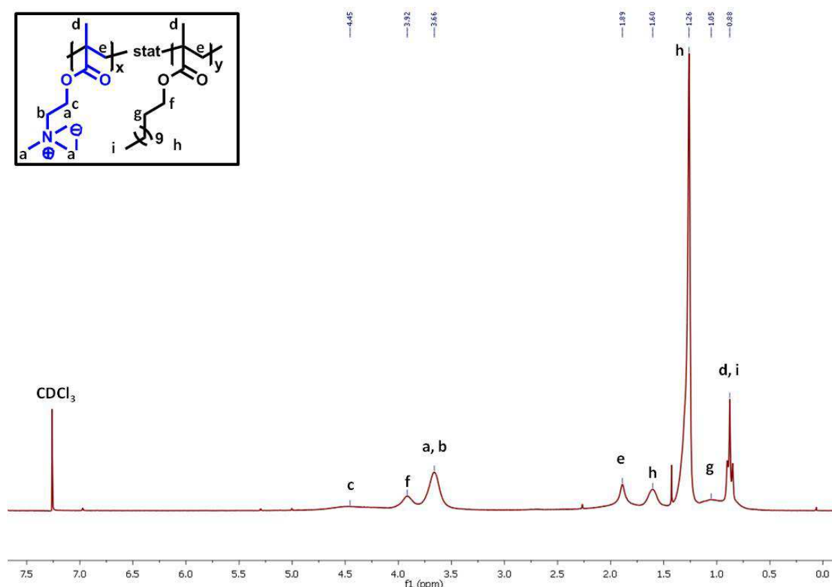
Abb. 8.3: ^1\text{H} -NMR-Spektrum von CP4(+) in \text{CDCl}_3 .
