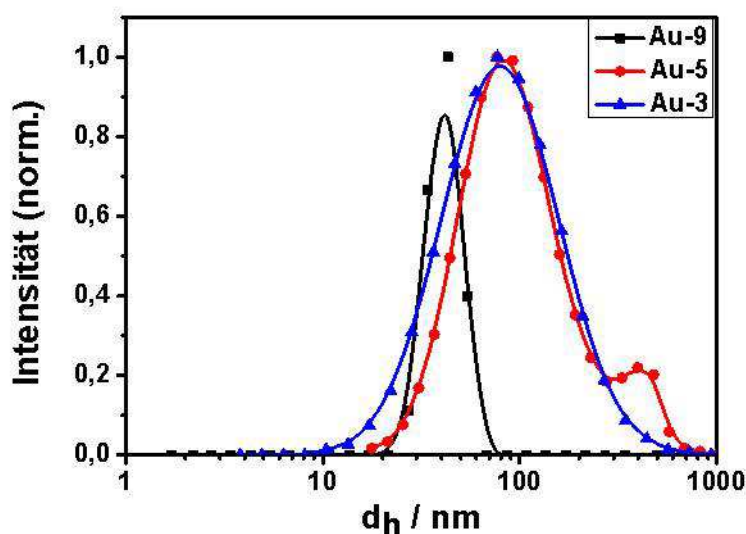
Abb. 3.5: DLS-Experimente der Proben Au-3 , Au-5 und Au-9 .
