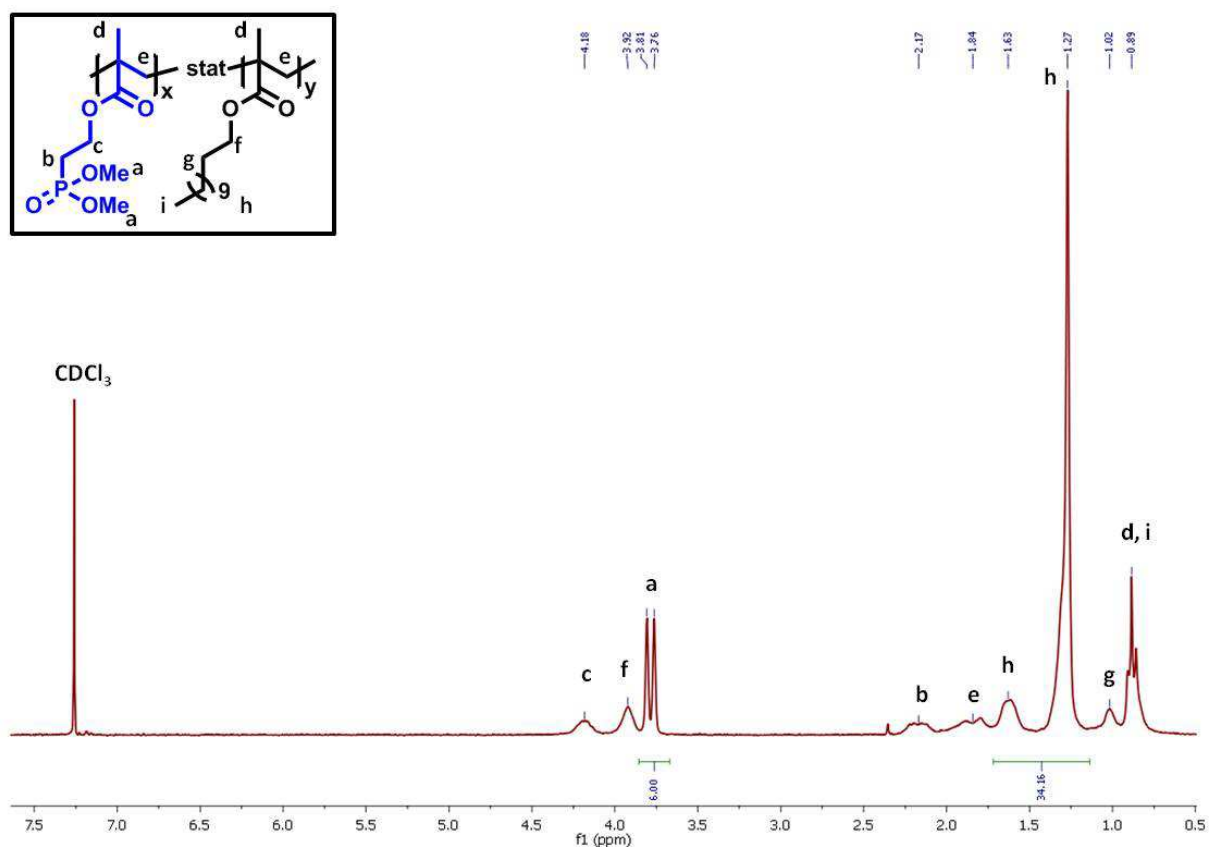
Abb. 8.6: ^1\text{H} -NMR-Spektrum von CN2 in \text{CDCl}_3 .
