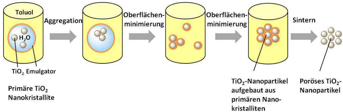
Abb. 6.2: Schematische Darstellung der Synthese poröser \text{TiO}_2 -Nanopartikel in der inversen Emulsion.
