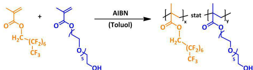
Abb. 7.6: Synthese von CP-PEOMA .
