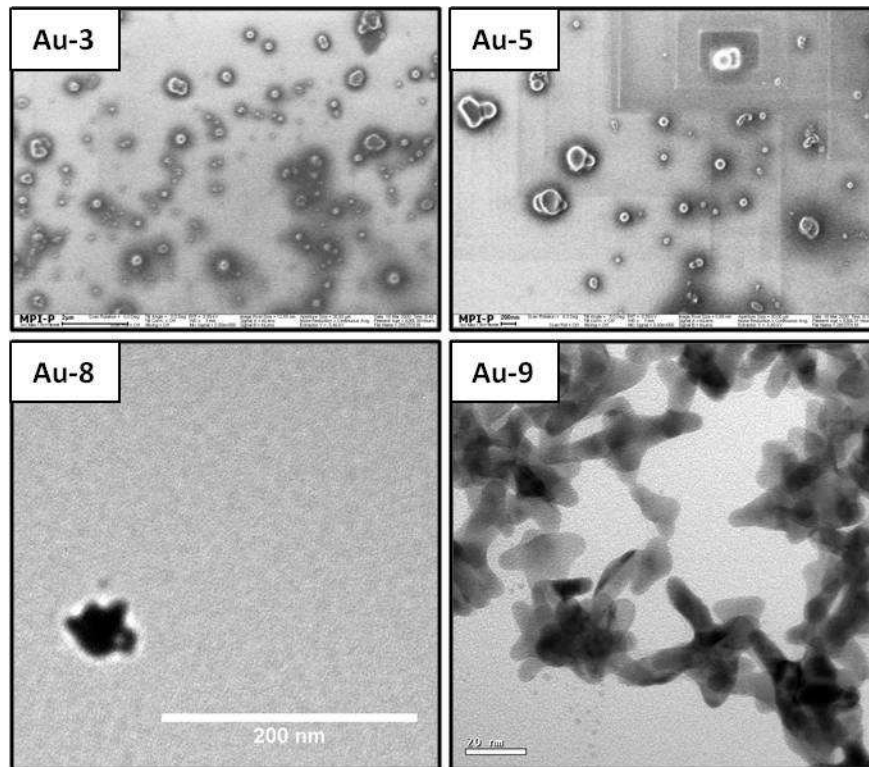
Abb. 3.2: Elektronenmikroskopische Aufnahme der Proben Au-3 , Au-5 , Au-8 und Au-9 .
