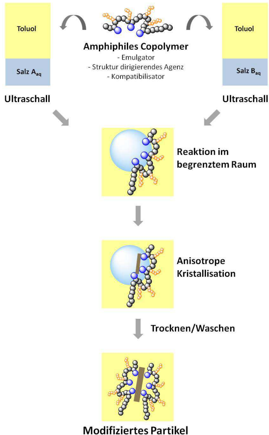
Abb. 2.1: Schematische Abbildung der inversen Emulsionstechnik bei Verwendung Struktur-dirigierender Emulgatoren (SDE).
