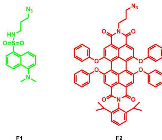
Abb. 8.32: Strukturformeln der Farbstoffe F1 und F2 .
