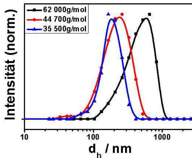
Abb. 2.20: Mittels DLS bestimmte, ungewichtete Durchmesser-Verteilung der Proben ZnO-7 , ZnO-9 und ZnO-10 bei einem Winkel von 90°.
