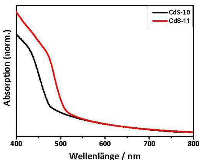
Abb. 4.12: UV-Vis-Spektren der Partikel CdS-10 und CdS-11 dispergiert in Toluol.
