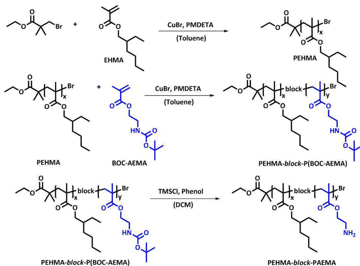
Abb. 4.6: Synthese der Polymere PEHMA, SDA-1 bis SDA-3.
