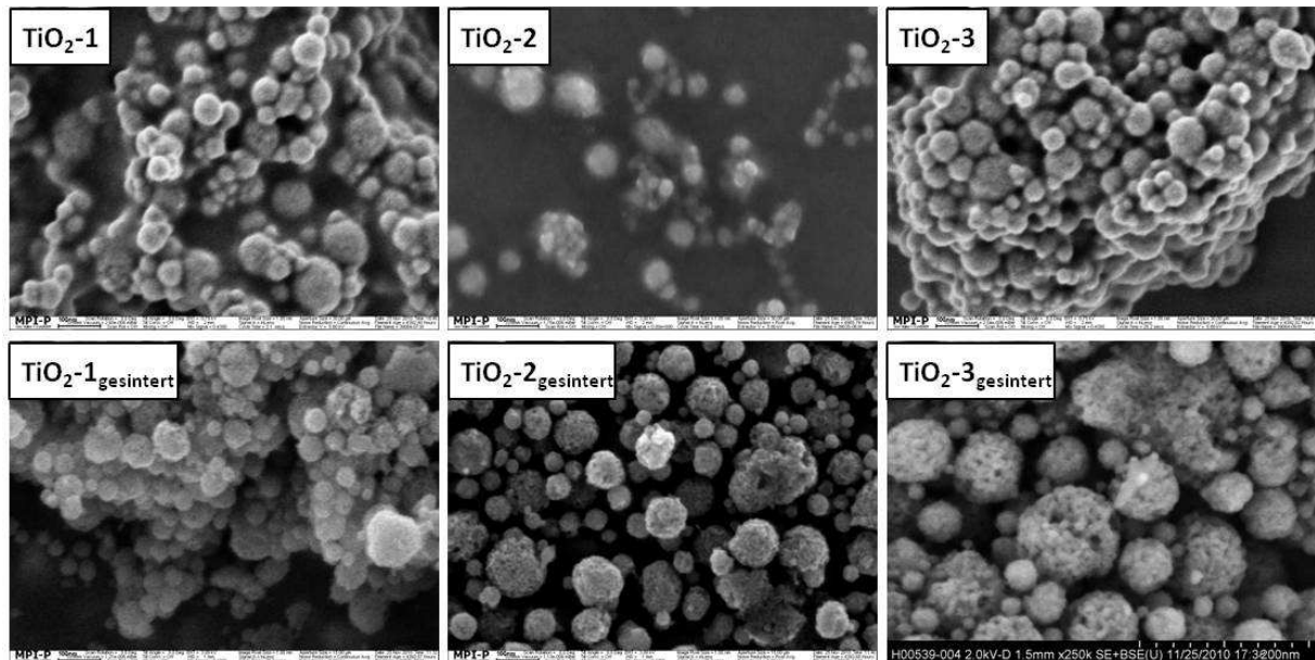
Abb. 6.8: REM-Aufnahmen der Proben TiO 2 -1 bis TiO 2 -3 vor und nach dem Sintern.
