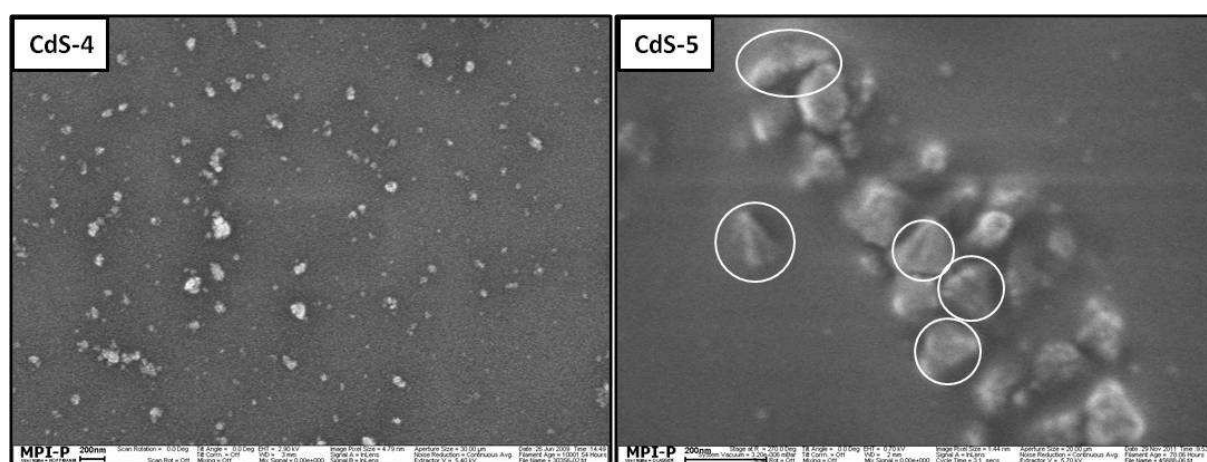
Abb. 4.3: REM-Aufnahmen der Proben CdS-4 und CdS-5 .
