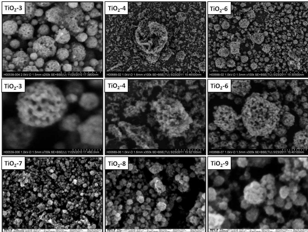
Abb. 6.12: (HR)REM-Aufnahmen der Proben TiO 2 -3 bis TiO 2 -7 und TiO 2 -9 nach dem Sintern.
