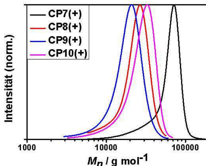
Abb. 8.20: GPC-Kurven der durch ATRP dargestellten Copolymere CP7(+) bis CP10(+) .
