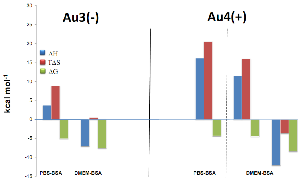
Abb. 8.40: Thermodynamischen Profile der Wechselwirkungen der Au-Nanopartikel Au3(-) bzw. Au4(+) mit PBS-BSA bzw. DMEM-BSA .
