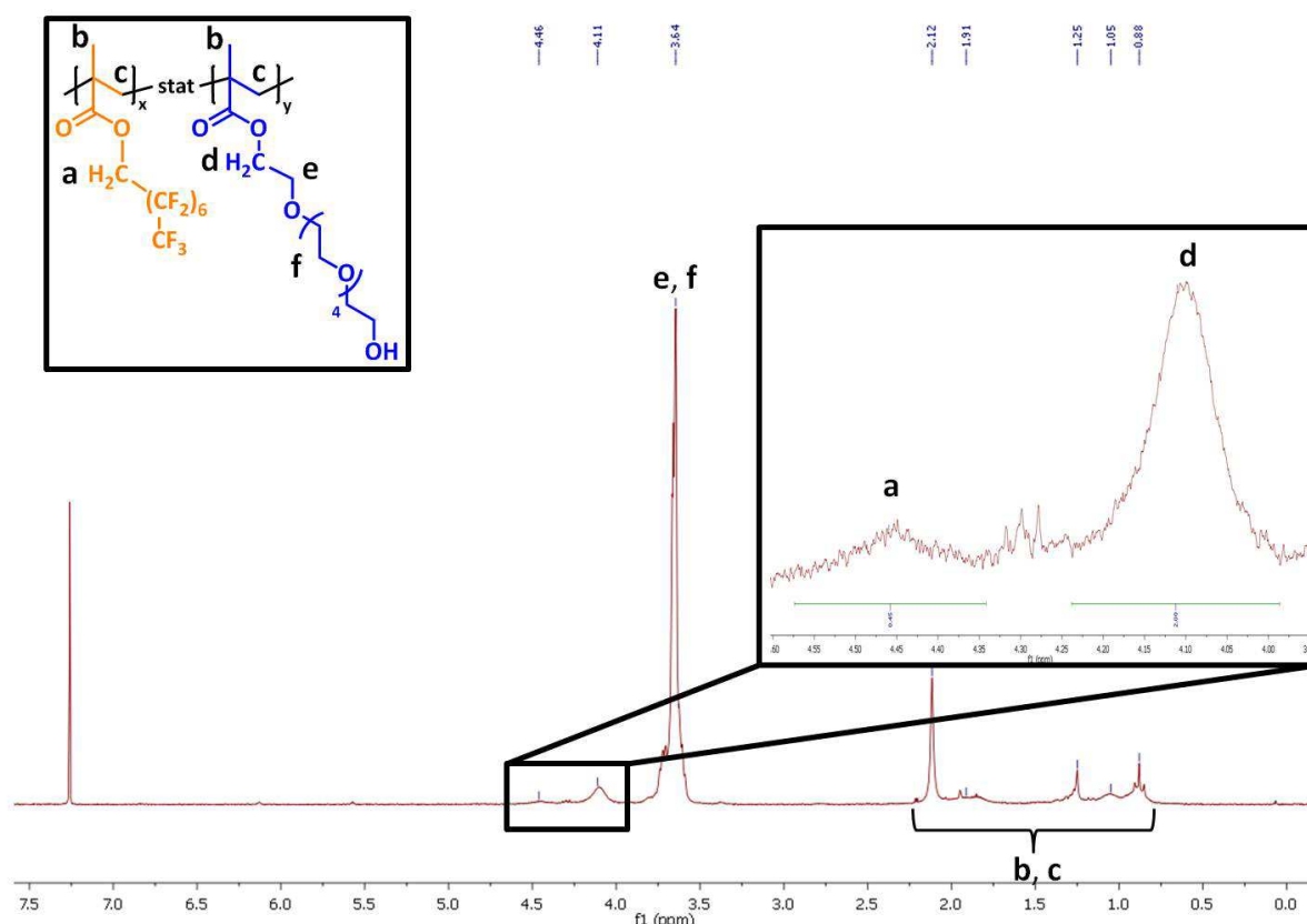
Abb. 7.7: ^1\text{H} -NMR-Spektrum von CP-PEOMA1 .
