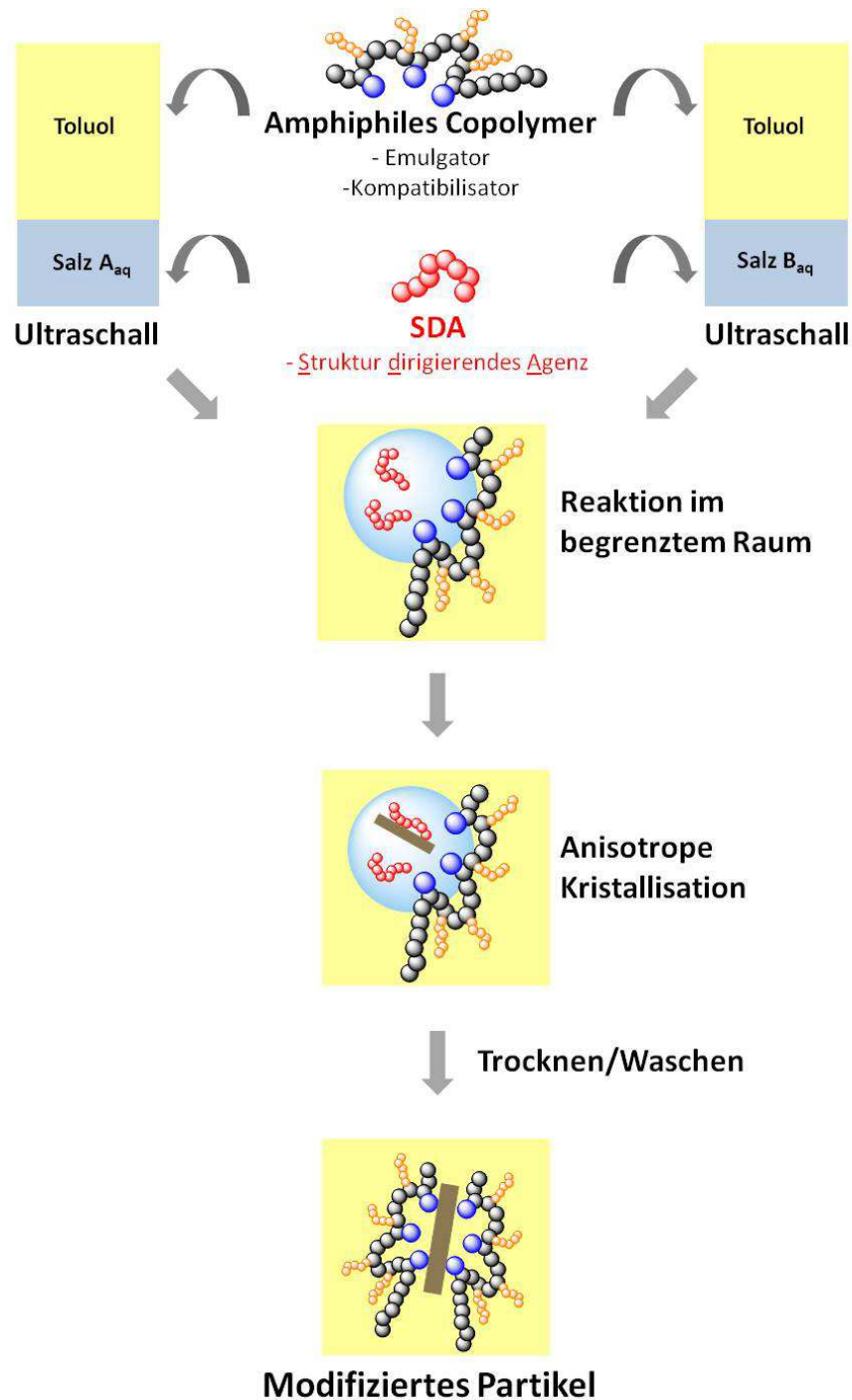
Abb. 2.12: Schematische Abbildung der inversen Emulsionstechnik mit gleichzeitiger Anwendung von Struktur-dirigierender Agenzien (SDA).
