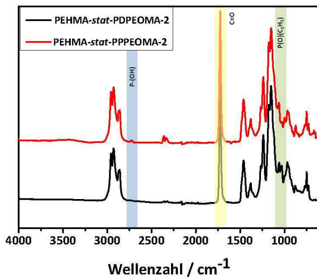
Abb. 2.6: IR-Spektren von PEHMA-stat-PDPEOMA-2 und PEHMA-stat-PPPEOMA-2.
