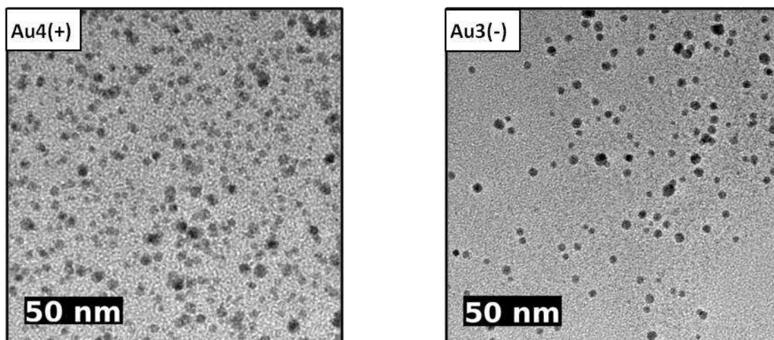
Abb. 8.12: TEM-Bilder der mit CP4(+) und CN3(-) umhüllten Au-Nanopartikel Au4(+) und Au3(-) . Daten von AK Parak.
