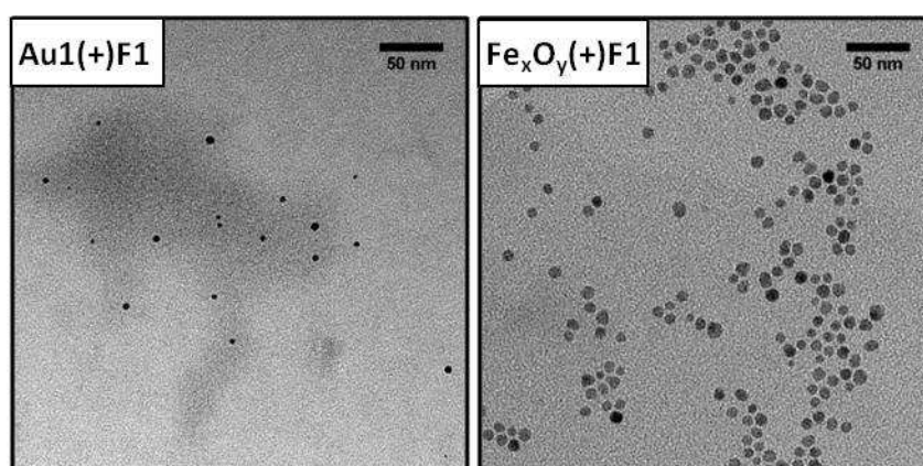
Abb. 8.27: TEM-Bilder der Partikel Au1(+) F1 und Fe x O y (+) F1.
