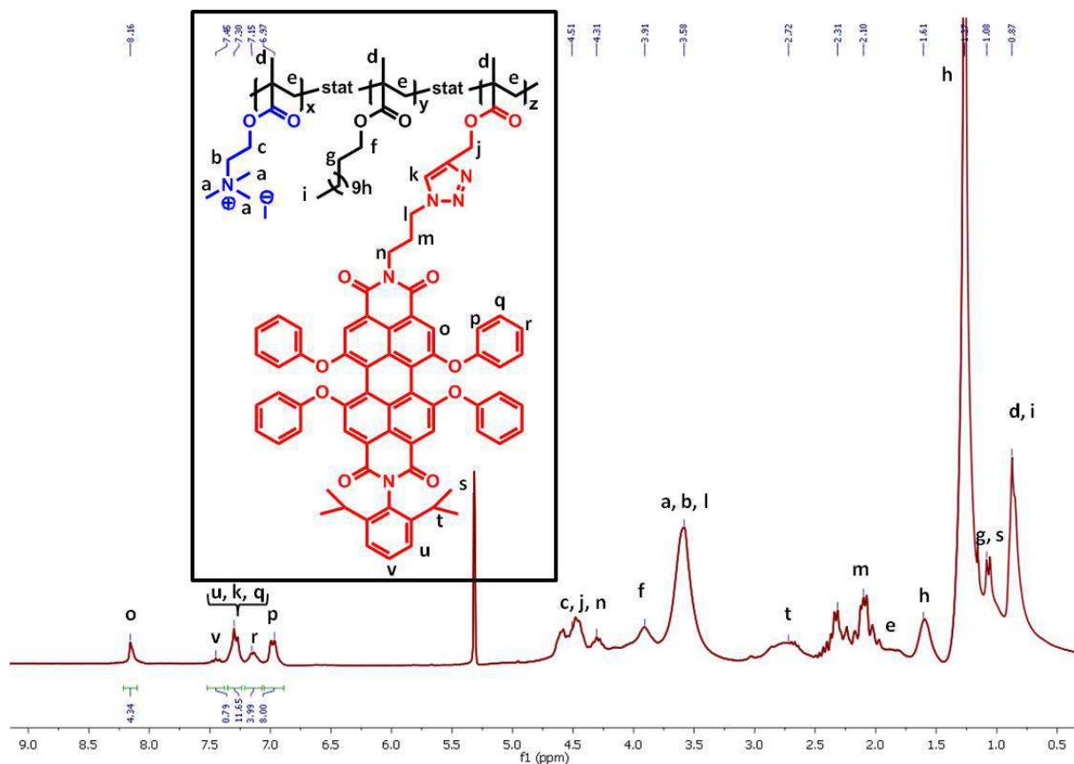
Abb. 8.35: ^1\text{H} -NMR-Spektrum von TP2(+)-F2 in \text{CDCl}_3 .
