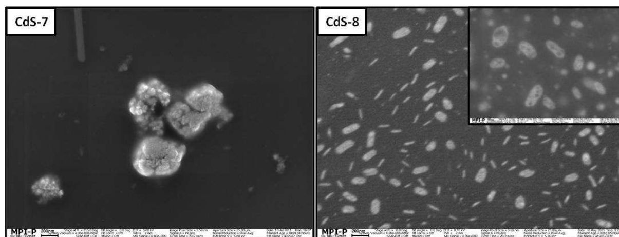
Abb. 4.4: REM-Aufnahmen der Proben CdS-7 und CdS-8 .
