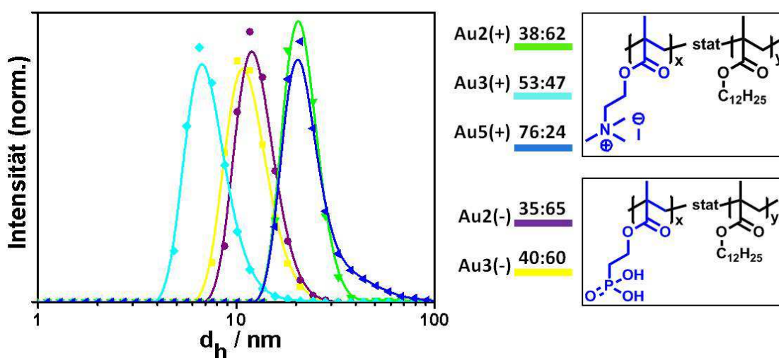
Abb. 8.14: DLS-Kurven der wässrigen Dispersionen der Au-Nanopartikel Au2(+) und Au4(+) und Au5(+) sowie Au2(-) und Au3(-) . Daten von AK Parak.
