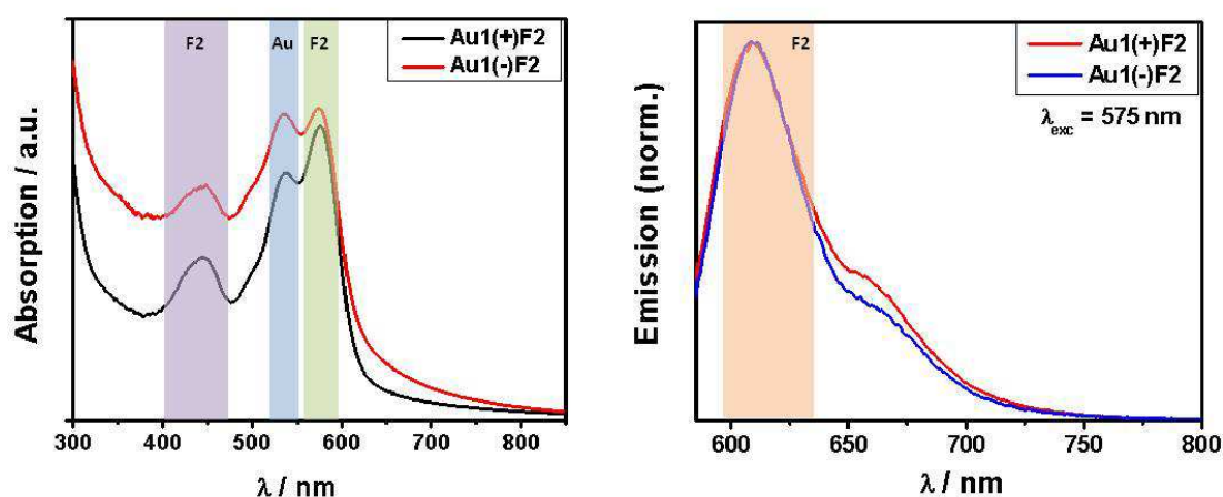
Abb. 8.38: UV-Vis- und PL-Spektren der Partikel Au1(+)-F2 und Au1(-)-F2 . Daten AK Parak.
