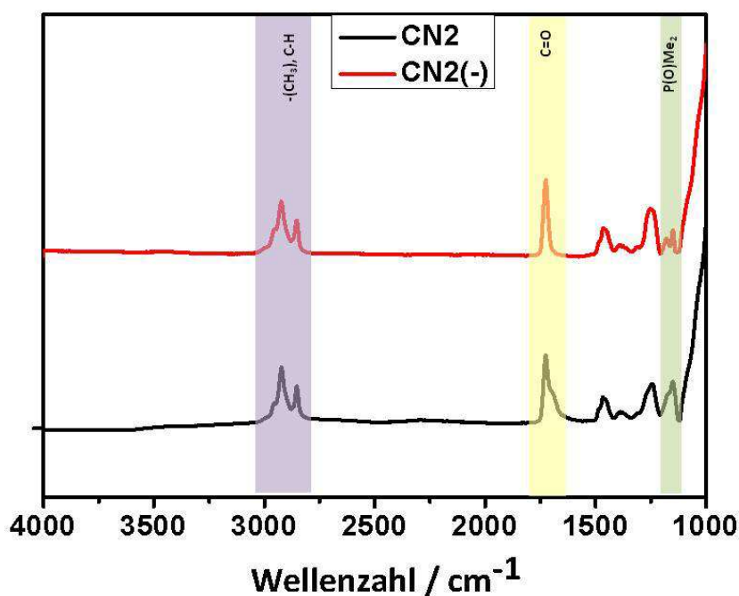
Abb. 8.8: IR-Spektren der amphiphilen Copolymere CN2 und CN2(-).
