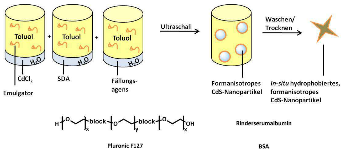
Abb. 4.1: Versuchsaufbau zur Darstellung in-situ hydrophobierter, formanisotroper CdS-Nanopartikel über das inverse Emulsionsverfahren (oben) und die verwendeten SDAs (unten).
