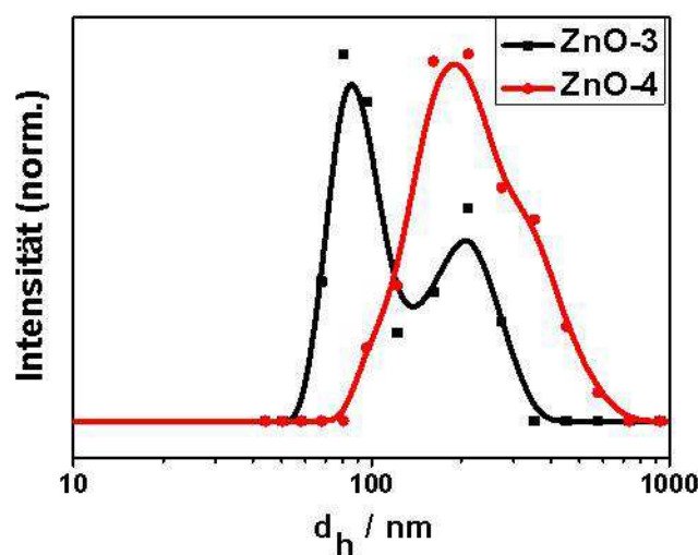
Abb. 2.10: Mittels DLS bestimmte ungewichtete Durchmesser-Verteilung der Proben ZnO-3 und ZnO-4 bei einem Winkel von 90°.
