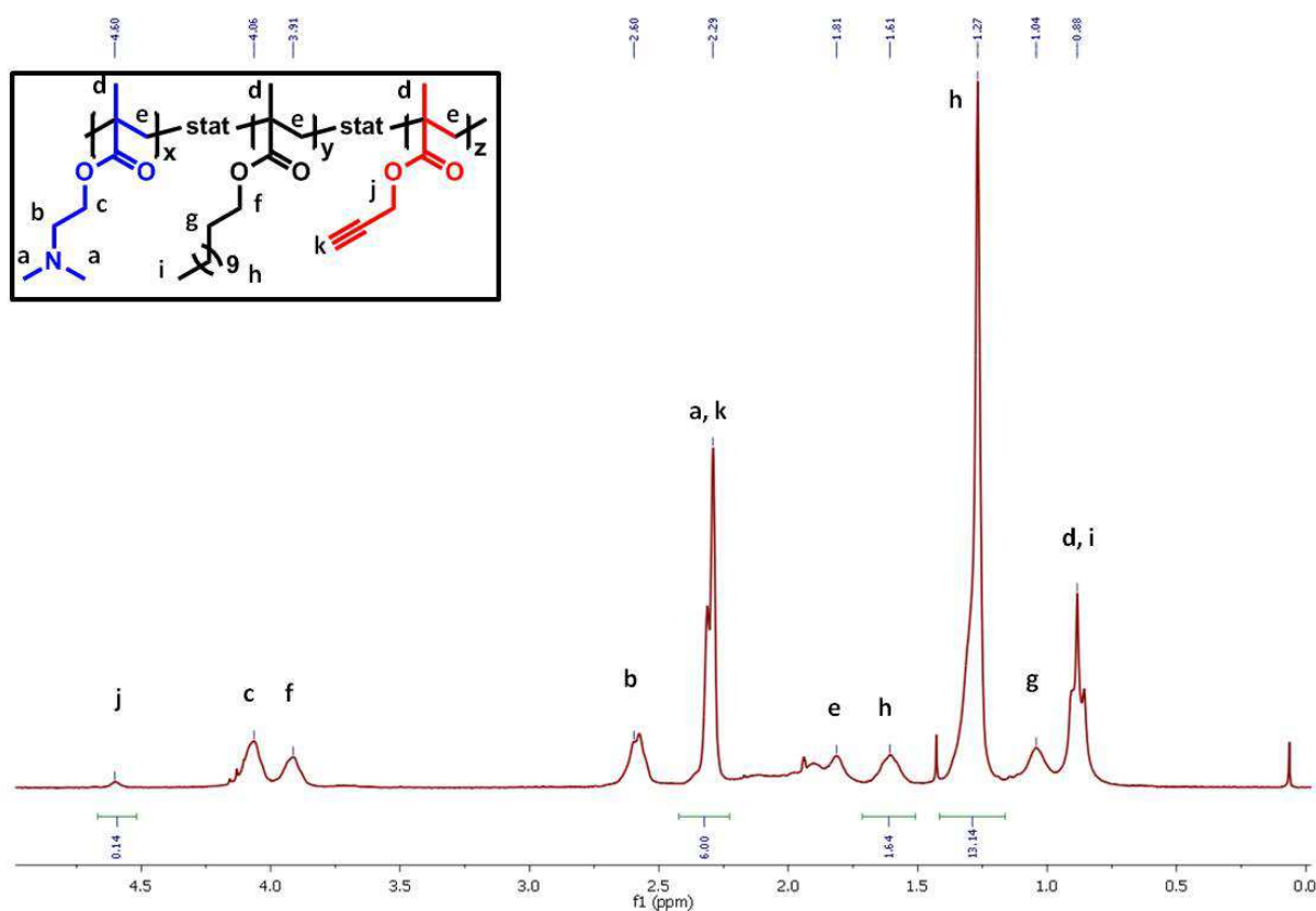
Abb. 8.23: ^1\text{H} -NMR-Spektrum von T2 in \text{CDCl}_3 .
