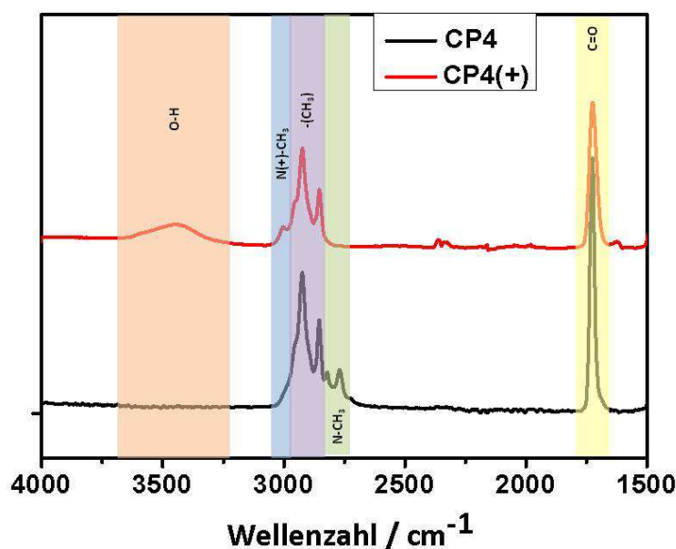
Abb. 8.4: IR-Spektren der amphiphilen Copolymere CP4 und CP4(+) .
