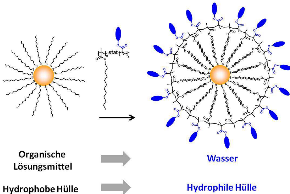
Abb. 8.9: Schematische Darstellung des Umhüllungsprozesses von hydrophoben anorganischen Nanopartikeln mit amphiphilen, statistischen, methacrylatbasierenden Copolymeren.
