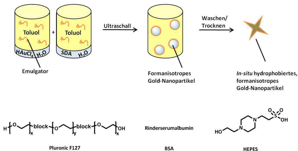
Abb. 3.1: Versuchsaufbau zur Darstellung in-situ hydrophobierter, formanisotroper Gold-Nanopartikel über das inverse Emulsionsverfahren (oben) und die verwendeten SDAs (unten).
