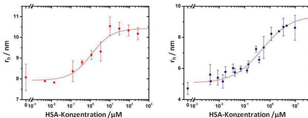
Abb. 8.39: HSA-abhängige Größenzuwächse der negativ geladenen Nanopartikel Au1(-)F2 und positiv geladenen Nanopartikel Au1(+)F2 . Daten AK Nienhaus.
