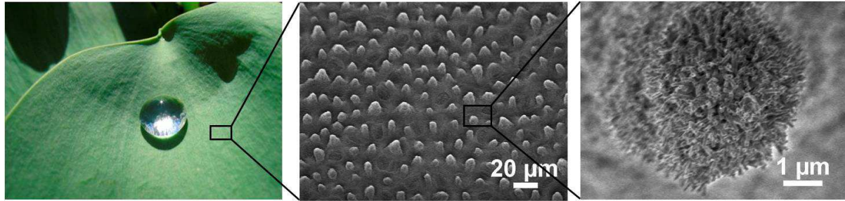
Abb. 7.1: Blatt der Lotusblüte bei verschiedenen Vergrößerungen.
