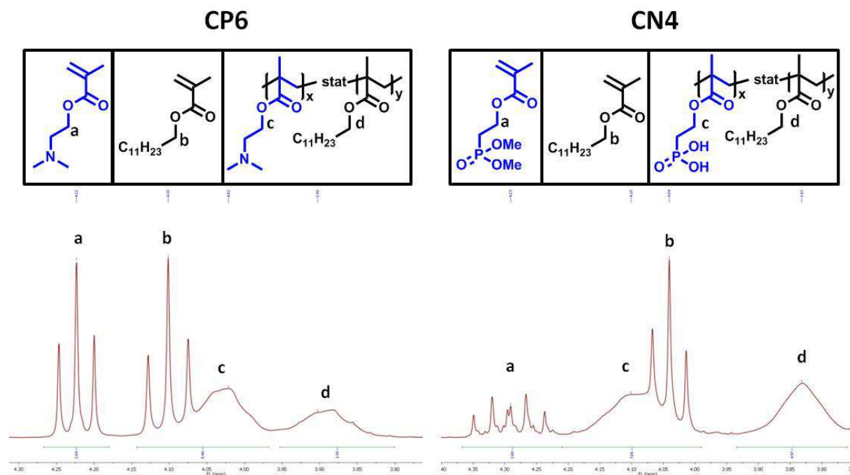
Abb. 8.17: Exemplarische Auswertung der ^1\text{H} -NMR-Spektren der Copolymerisation von CP6 und CN4 nach 150 min.
