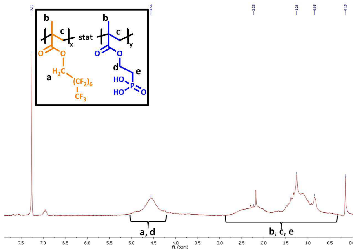
Abb. 7.11: ^1\text{H} -NMR-Spektrum von CP-MAPHOS1.
