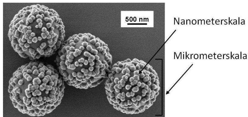
Abb. 7.2: „Himbeerpartikel“ Polystyrol- \text{SiO}_2 -Kern-Schale-Partikel.
