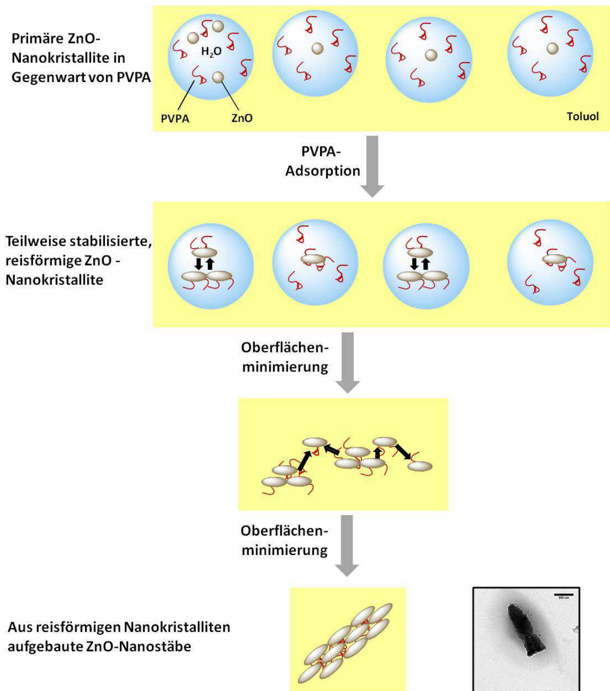
Abb. 2.22: Vermuteter Bildungsmechanismus der ZnO-Nanostäbe in der inversen Emulsion. Der Emulgator ist aufgrund besserer Übersichtlichkeit nicht dargestellt.
