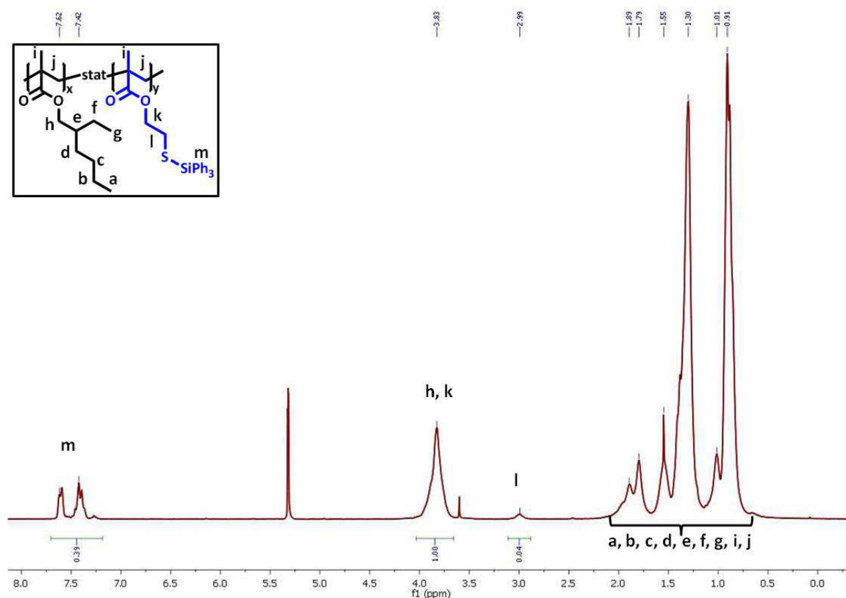
Abb. 3.7: ^1\text{H} -NMR-Spektrum von geschützten Em3 .
