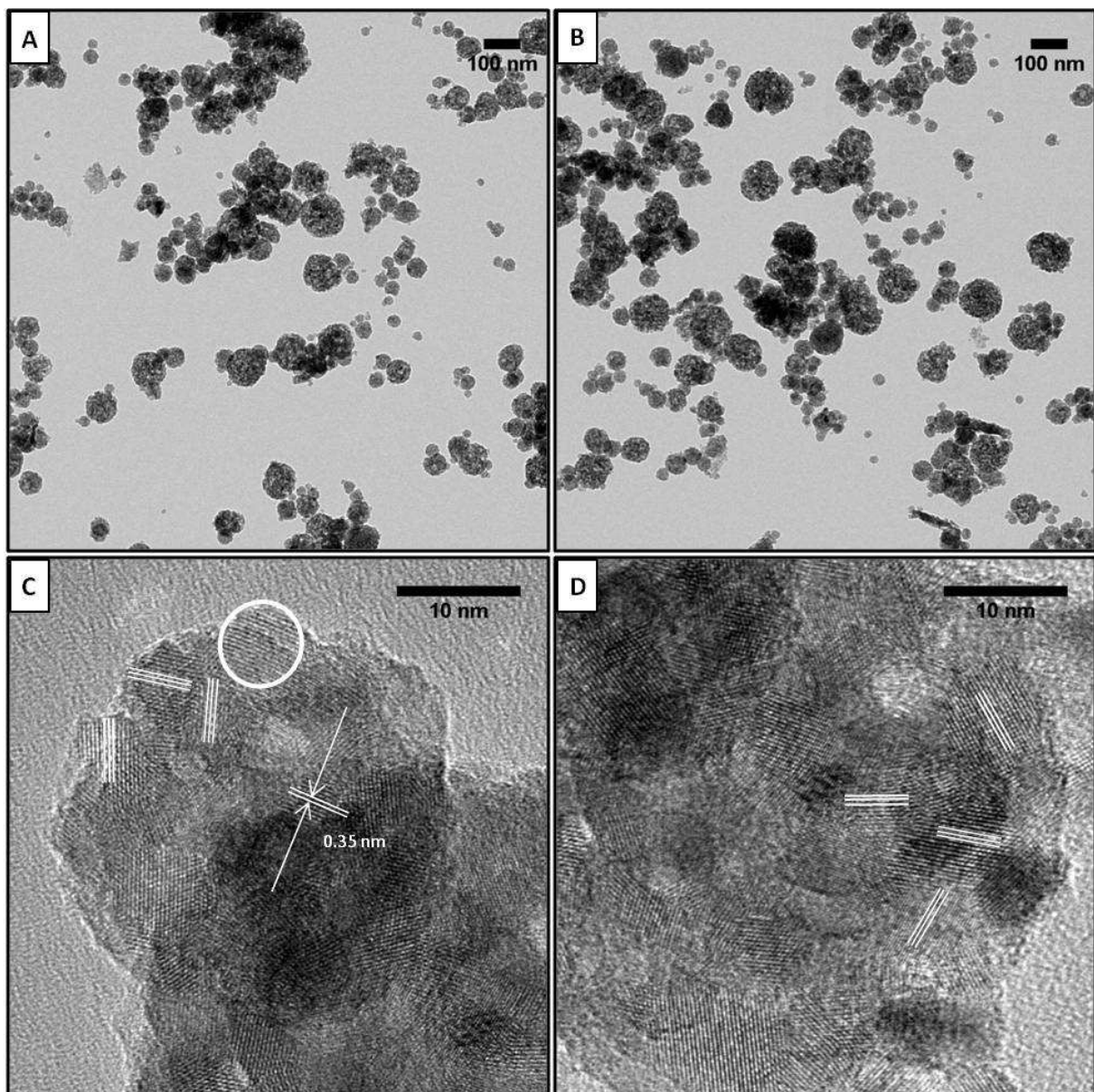
Abb. 6.9: (HR)TEM-Aufnahmen der Probe \text{TiO}_2 -3.
