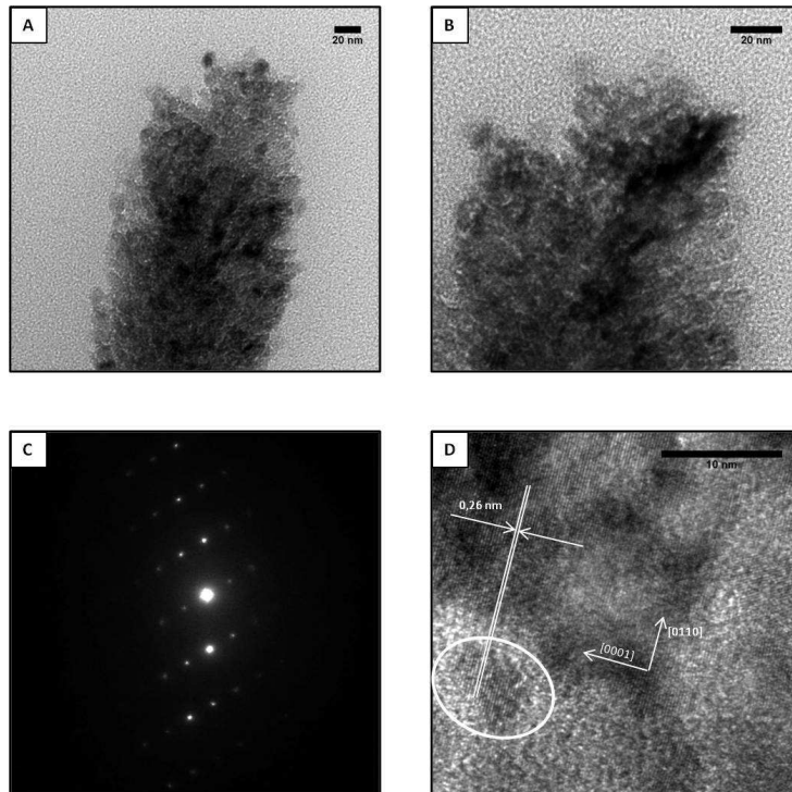
Abb. 2.19: A) TEM-Aufnahmen eines Partikels der Probe ZnO-7 . B) Vergrößerter Ausschnitt der Aufnahme A . C) Elektronenbeugung eines Bereichs des Partikels von B . D) Vergrößerter Ausschnitt von B .
