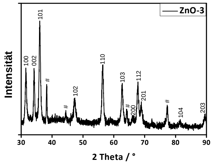
Abb. 2.8: Pulverdiffraktogramm der Probe ZnO-3 . # ... Signale des Al-Probenhalters.
