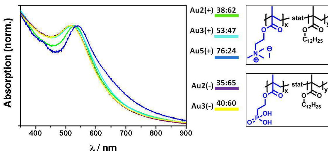
Abb. 8.13: UV-Vis Spektren der wässrigen Dispersionen der Au-Nanopartikel Au2(+) und Au4(+) und Au5(+) sowie Au2(-) und Au3(-) . Daten von AK Parak.
