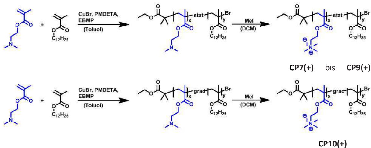
Abb. 8.19: Mittels ATRP hergestellte, positiv geladene Copolymere CP7(+) bis CP10(+) .
