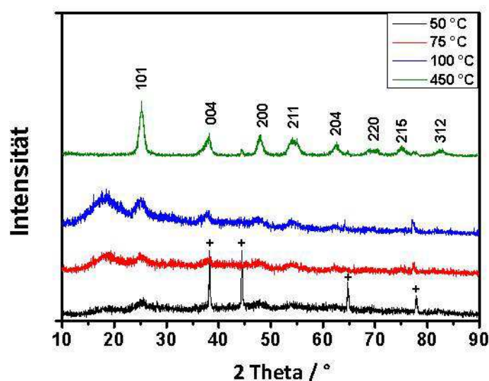
Abb. 6.7: Pulverdiffraktogramme der Proben TiO 2 -1 bis TiO 2 -3 vor und TiO 2 -3 nach dem Sintern.
