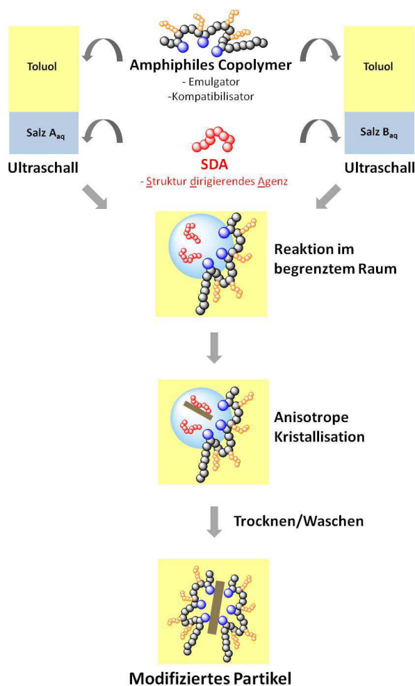
Abb.10.1: Inverse Emulsionstechnik mit gleichzeitiger Anwendung von Struktur-dirigierenden Agenzien (SDA).
