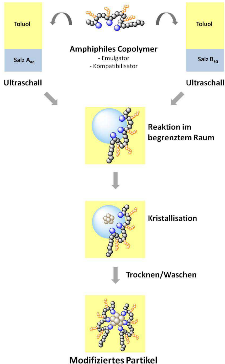
Abb. 1.1: Schematische Abbildung der inversen Emulsionstechnik nach Khrenov et al. [3a, b, c, d]
