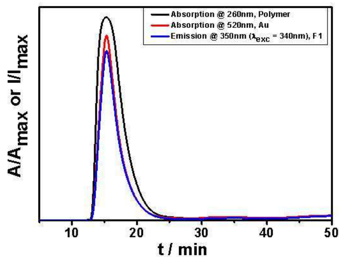
Abb. 8.29: HPLC nach der Postfunktionalisierung.
