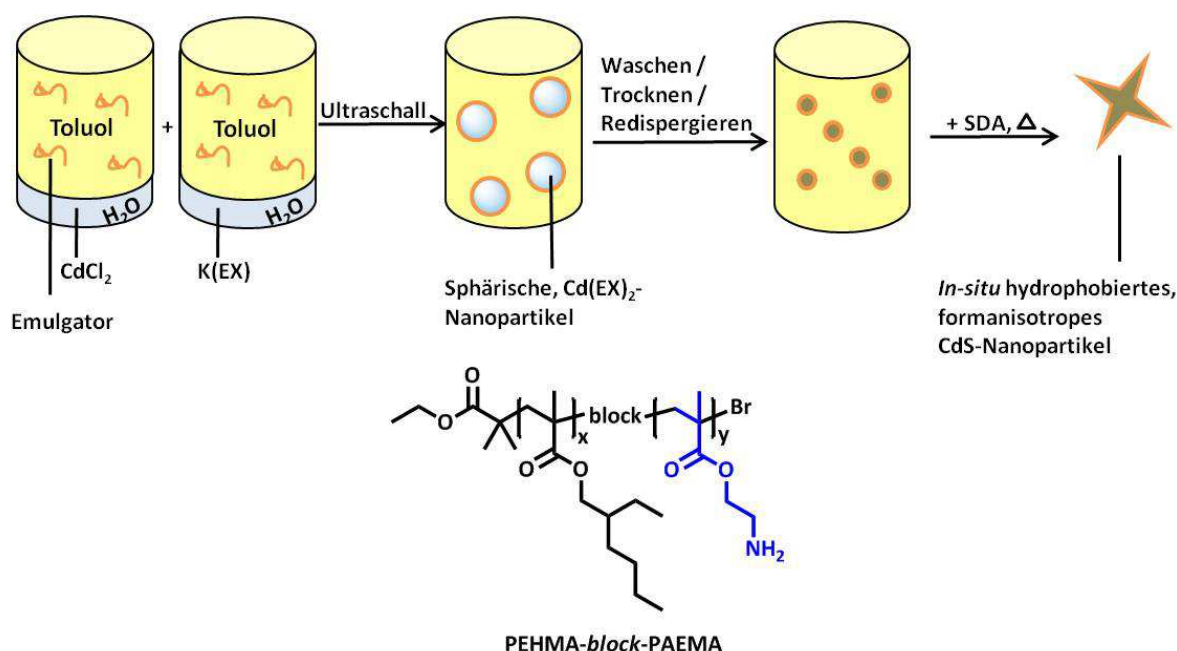
Abb. 4.5: Versuchsaufbau zur Darstellung in-situ hydrophobierter, formanisotroper CdS-Nanopartikel über das inverse Emulsionsverfahren (oben) und die verwendeten SDAs (unten).
