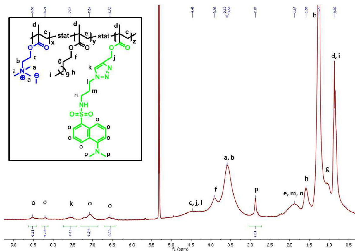
Abb 8.34: ^1\text{H} -NMR-Spektrum von TP2(+)-F1 in \text{CDCl}_3 .
