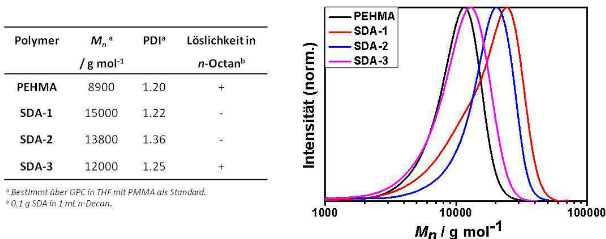
Abb. 4.7: GPC-Daten der Polymere PEHMA , SDA-1 bis SDA-3 .
