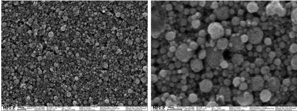
Abb. 6.16: REM-Aufnahmen von TiO 2 -Film4 nach dem Sintern.
