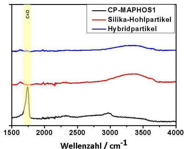
Abb. 7.12: IR-Spektrum von CP-MAPHOS1 , \text{SiO}_2 -Hohlpartikel und Hybridpartikeln.
