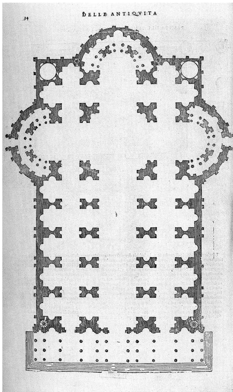
Abb. 12: Grundriss der Peterskirche mit dem gegenüber der Julius-Planung erheblich vergrößerten Projekt von Bramante und Raffael für Leo X. von 1514; Holzschnitt, Sebastiano Serlio, Terzo Libro di architettura , Venedig 1540.
