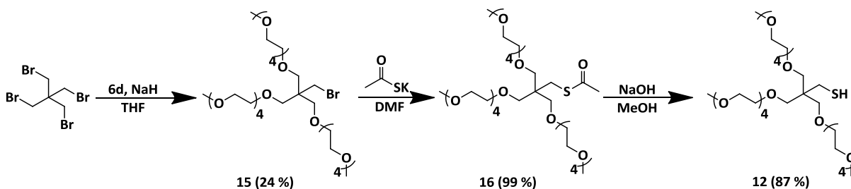
Abb. 3-7: Synthese 3-((( \alpha -Methoxytetra(ethylenglyco)l)oxy)methyl)-2,2-bis(( \alpha -methoxytetra(ethylenglykol)oxy)methyl)-propyl-3-thiol ( 12 ).
