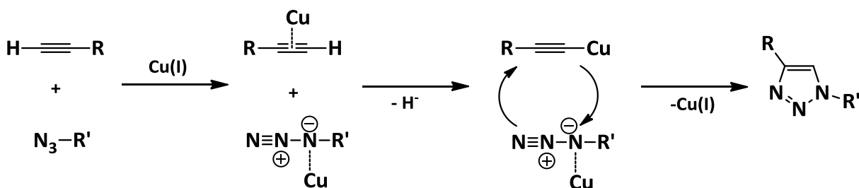
Abb. 3-12: Allgemeiner Mechanismus der 1,3-dipolaren Cycloaddition von Aziden und Alkinen. [50]
