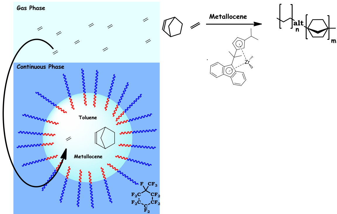
Abb. 7-3: Copolymerisation von Norbornen und Ethylen in fluoridierter Emulsion.
