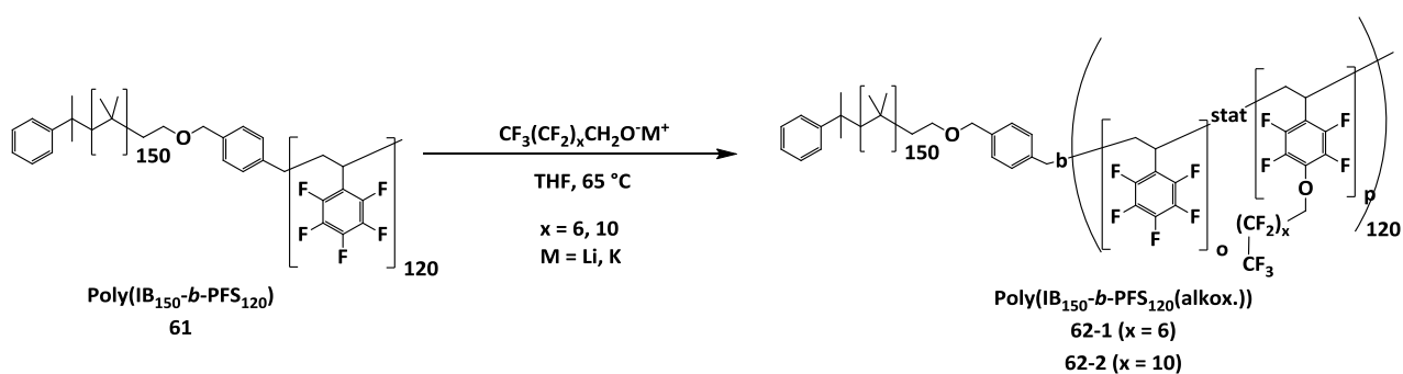
Abb. 5-7: Nucleophile aromatische Substitution von 61 zur Einführung einer 1 H ,1 H -Perfluoralkoxy-Gruppe in den PFS-Block.
