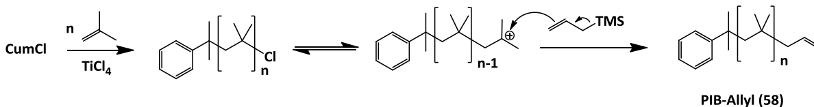
Abb. 5-3: \beta -Desilylierung von Allyltrimethylsilan im Anschluss an die carbo-kationische IB Polymerisation.
