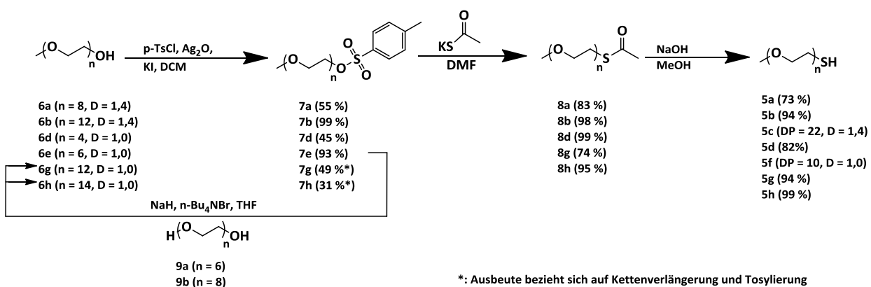
Abb. 3-3: Synthese von \alpha -Methoxy- \omega -mercapto-poly(ethyleneglykol)en ( 5a,b,d,e,g,h ) aus \alpha -Hydroxy- \omega -methoxy-poly(ethyleneglykol)en ( 6a,b,d,e,g,h ) unterschiedlicher Kettenlänge und Polydispersität.
