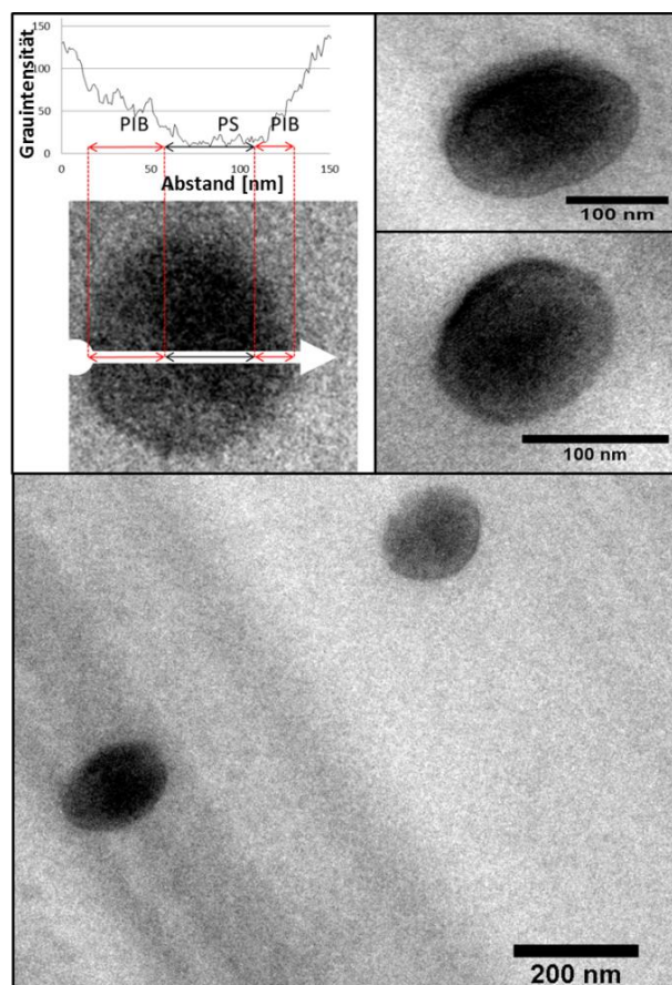
Abb. 5-21: TEM-Aufnahmen von 64-1 und 64-2 , Proben hergestellt durch Einbetten in Epoxy-Matrix, Mikrotomschneiden und Anfärben mit RuO 4 -Dampf.
