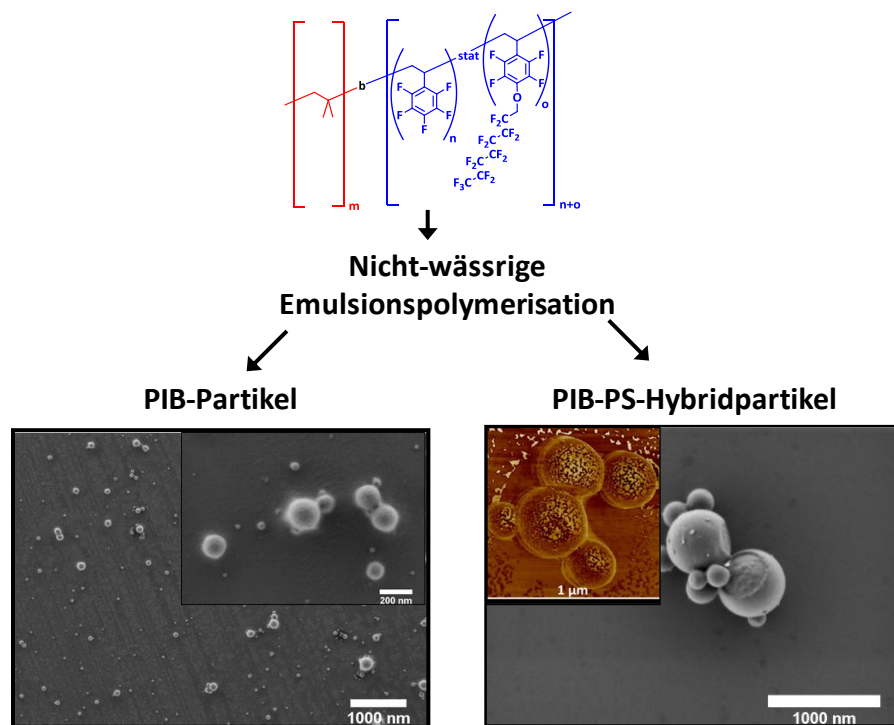
Abb. 7-2: Überblick zur Anwendung des fluorierten Blockcopolymers Poly(IB- b -PFS(alkox.)).
