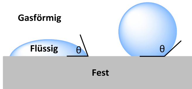
Abb. 1-5: Verhalten von Lösungsmitteln an der festen Grenzfläche: vollständiges und partielles Benetzen.
