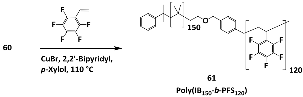
Abb. 5-5: ATRP von PFS mit 60 .
