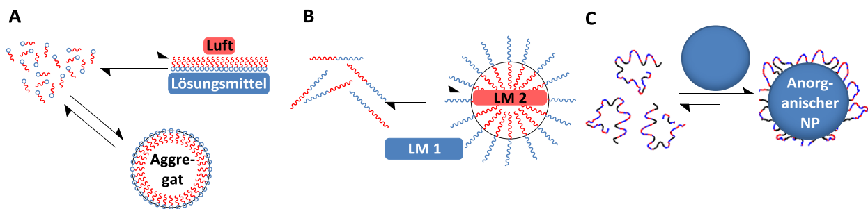
Abb. 1-6: Adsorptionsverhalten von Amphiphilen mit unterschiedlichem Molekulargewicht und Architektur in Lösung: A) niedermolekular, B) Blockcopolymer und C) statistisches Copolymer.
