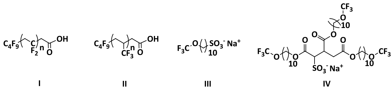
Abb. 3-1: Strukturen von potentiell nicht-bioakkumulativen Fluortensiden. [1]
