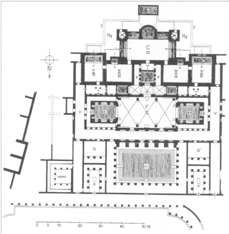
Abbildung 8: Grundriß der großen Thermen in Leptis Magna (aus: Krencker, Kaiserthermen, Abbildung 301).
