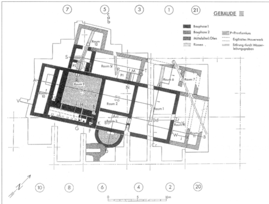
Abbildung 10: Badegebäude in Hochscheid (aus: Weisgerber, Hochscheid, Beilage 4).
