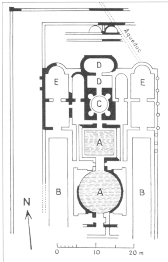
Abbildung 9: Grundriß der Thermen in Neris (aus: Grenier, Manuel IV, Abbildung 136).
