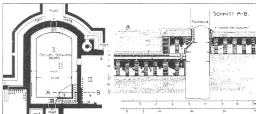
Abbildung 5: Eines der beheizten Schwimmbäder der Trierer Barbarathermen (aus: Krencker, Kaiserthermen, Abbildung 363).
