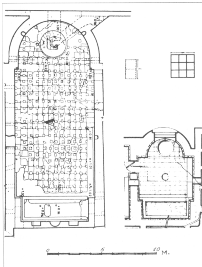
Abbildung 1: Grundrißvergleich des Caldariums der Stabianer Thermen und der Vorstadthermen in Herculaneum unter besonderer Berücksichtigung der Fenstergrößen (nach: Eschbach, Stabianer Thermen und Maiuri, Nuovi Scavi).
