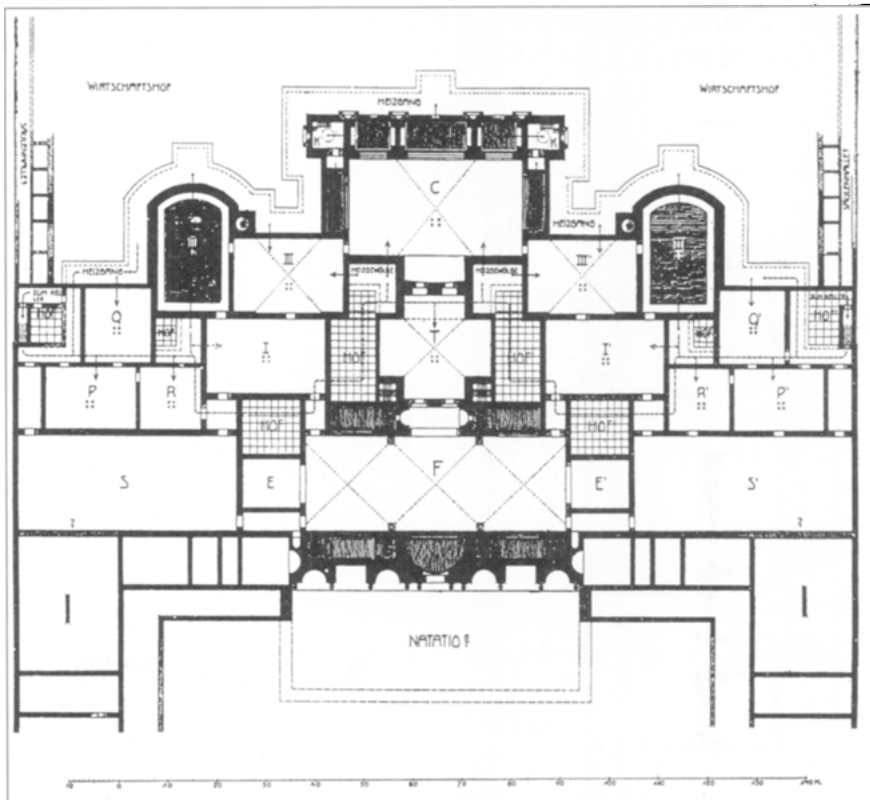
Abbildung 6: Grundriß der Barbarathermen (aus: Krencker, Kaiserthermen, Abbildung 359).
