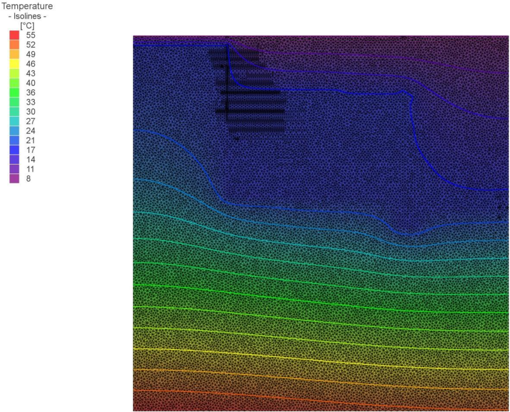
Abbildung 5-9 Temperaturverteilung in Szenario 2
