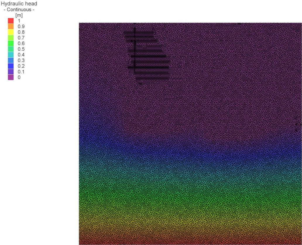
Abbildung 5-14 hydraulische Druckspiegelhöhenverteilung (hydraulic head) in Szenario 4
