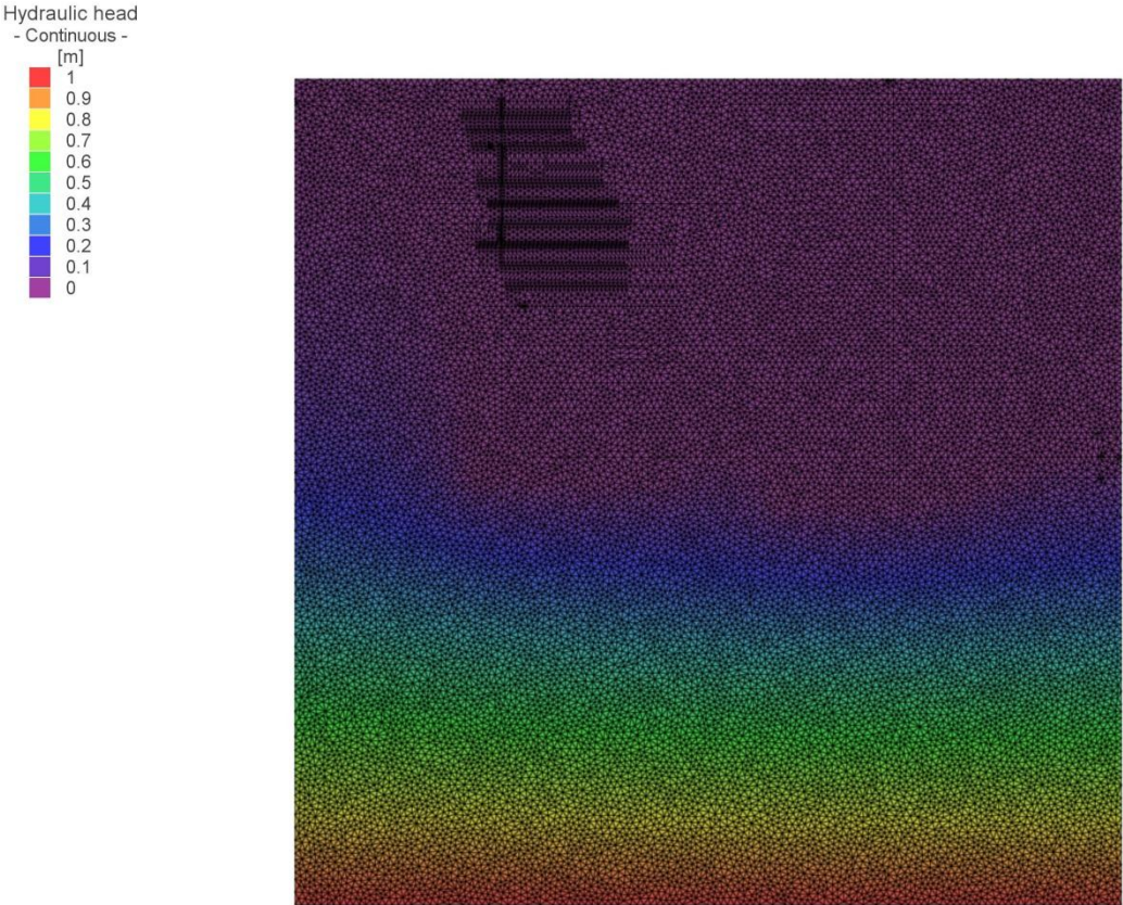
Abbildung 5-11 hydraulische Druckspiegelhöhenverteilung (hydraulic head) in Szenario 3
