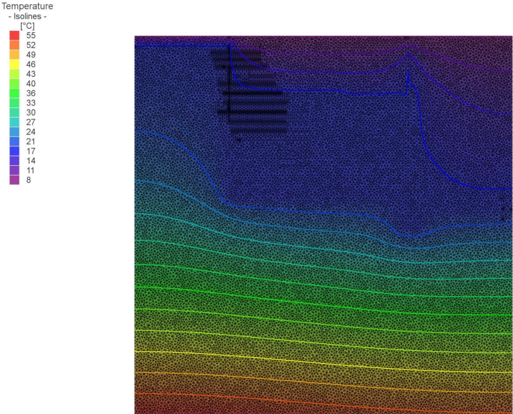
Abbildung 5-12 Temperaturverteilung in Szenario 3
