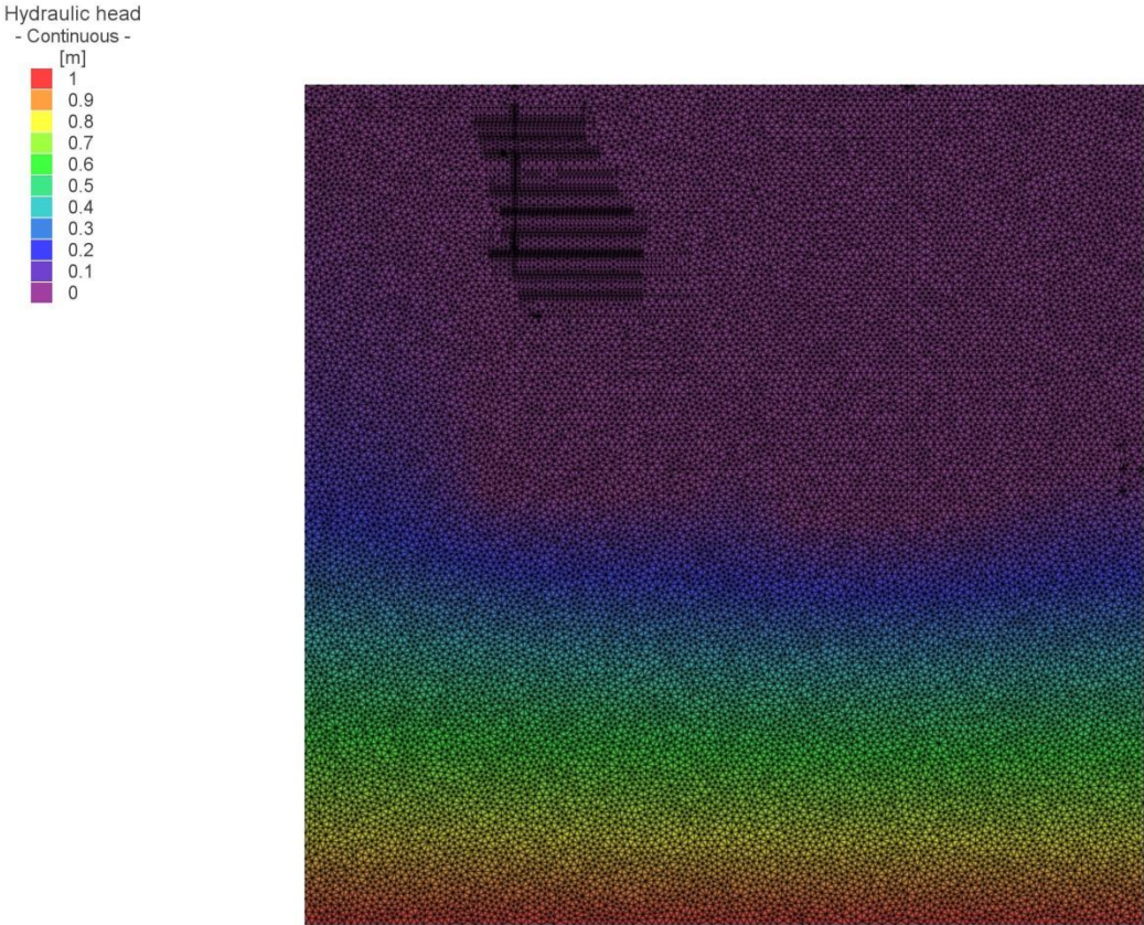
Abbildung 5-5 hydraulische Druckspiegelhöhenverteilung (hydraulic head) in Szenario 1
