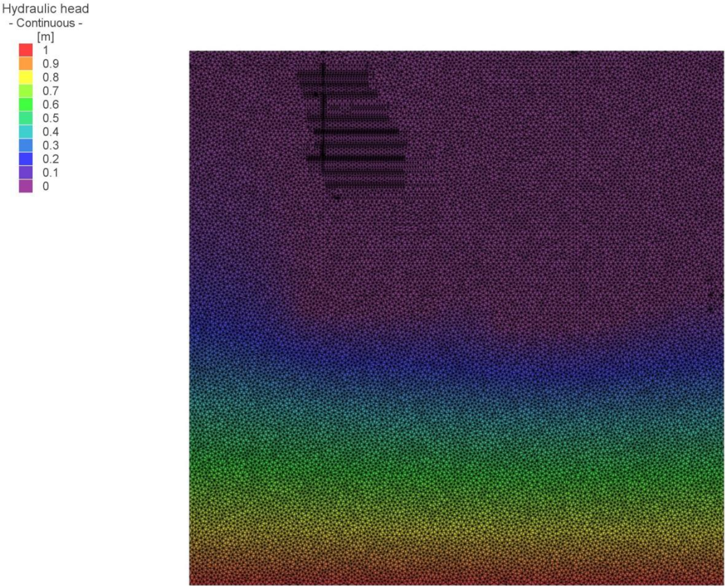
Abbildung 5-8 hydraulische Druckspiegelhöhenverteilung (hydraulic head) in Szenario 2
