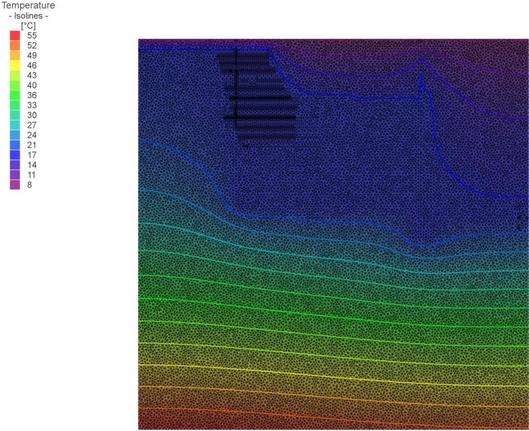
Abbildung 5-15 Temperaturverteilung in Szenario 4
