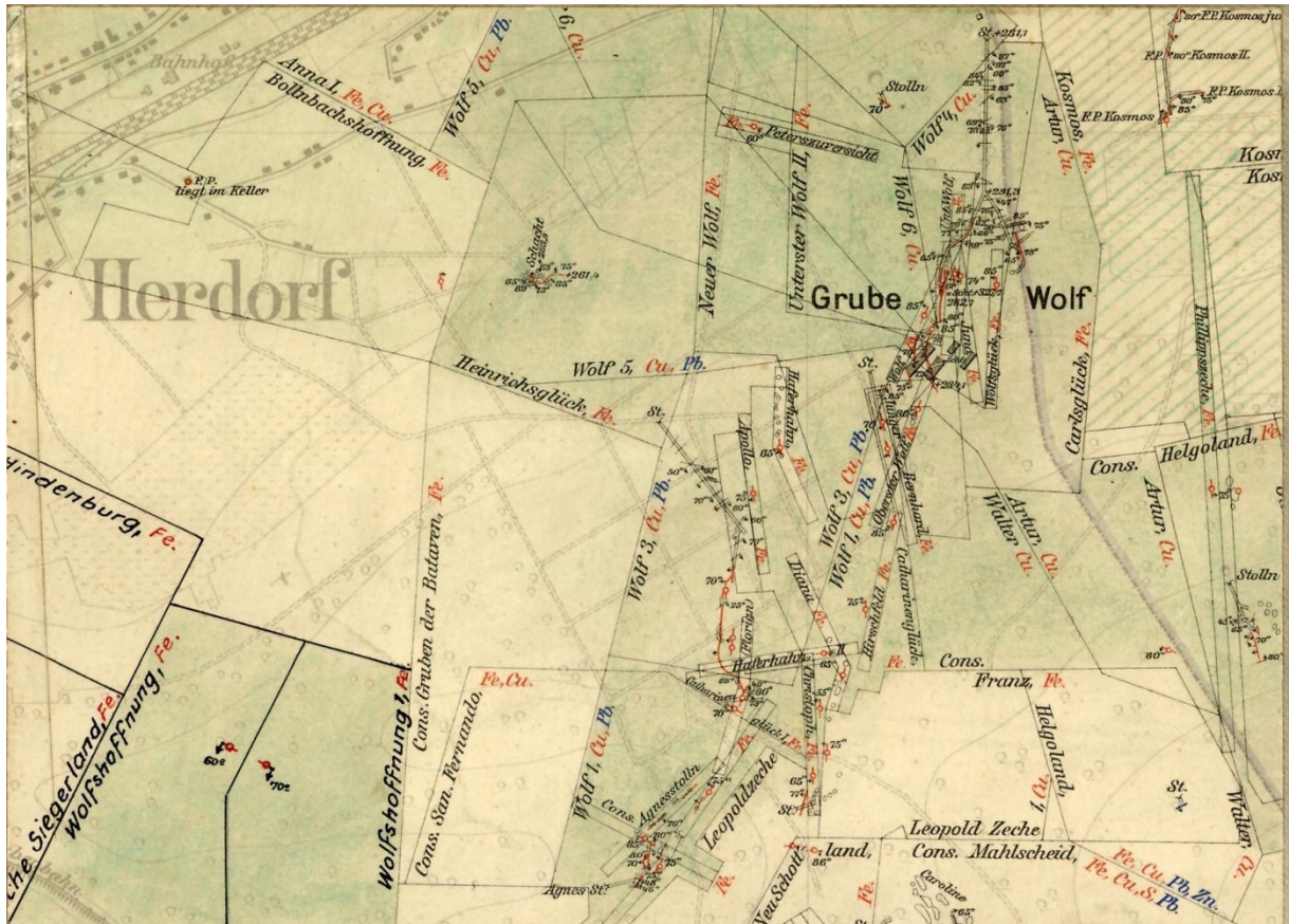
Abbildung 3-15 Gangkarte 1:10.000 (Ausschnitt) der Grube Wolf (1906-1923)
