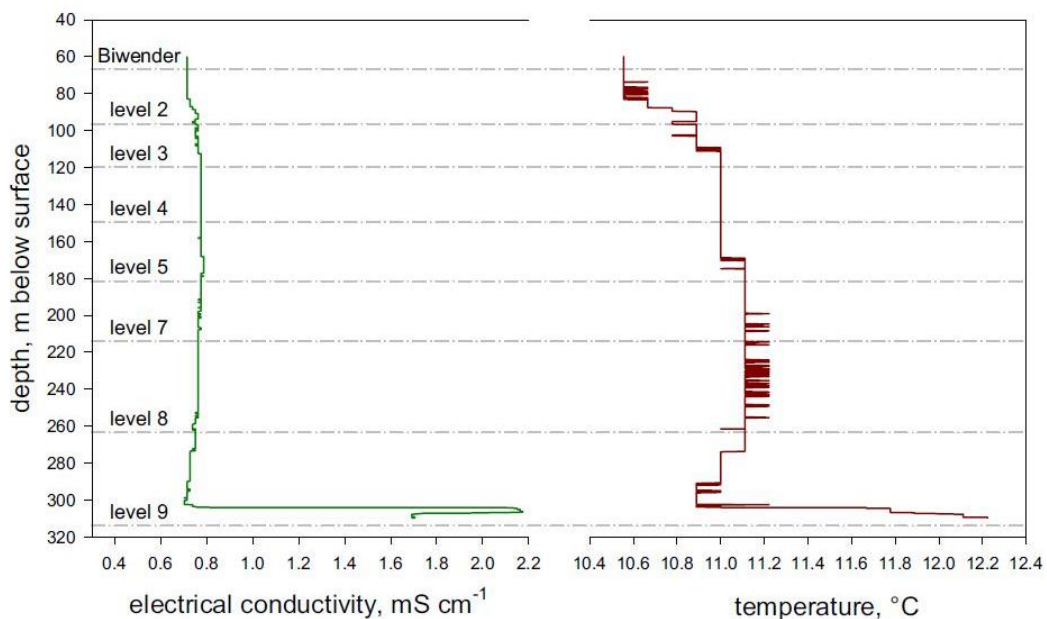
Abbildung 2-1 Leitfähigkeits- und Temperaturprofil des Fluor-Schachtes der Grube Straßberg/Harz (bearbeitet aus WOLKERSDORFER 2008)
