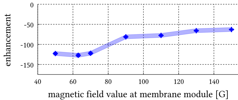
(b) para
