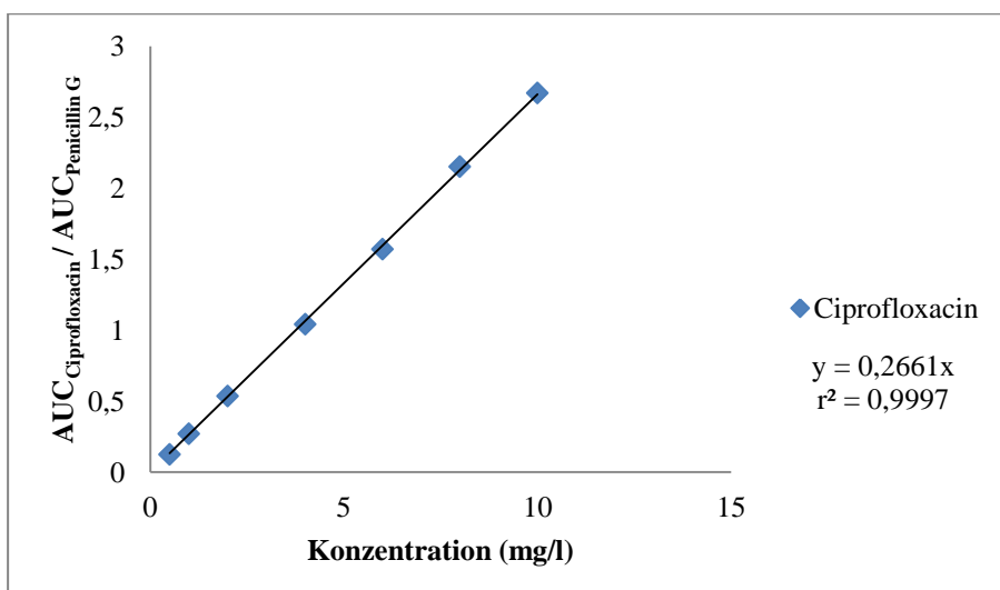
Abbildung 18: Kalibrationsgerade von Ciprofloxacin-Plasmaproben bei 280 nm, dargestellt sind die Mittelwerte der drei Messungen.
