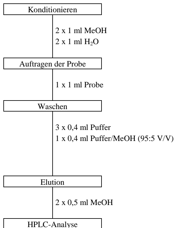
Abbildung 12: Schematische Darstellung der Festphasenextraktion der Plasmaproben für die Bestimmung von Piperacillin und Ciprofloxacin.
