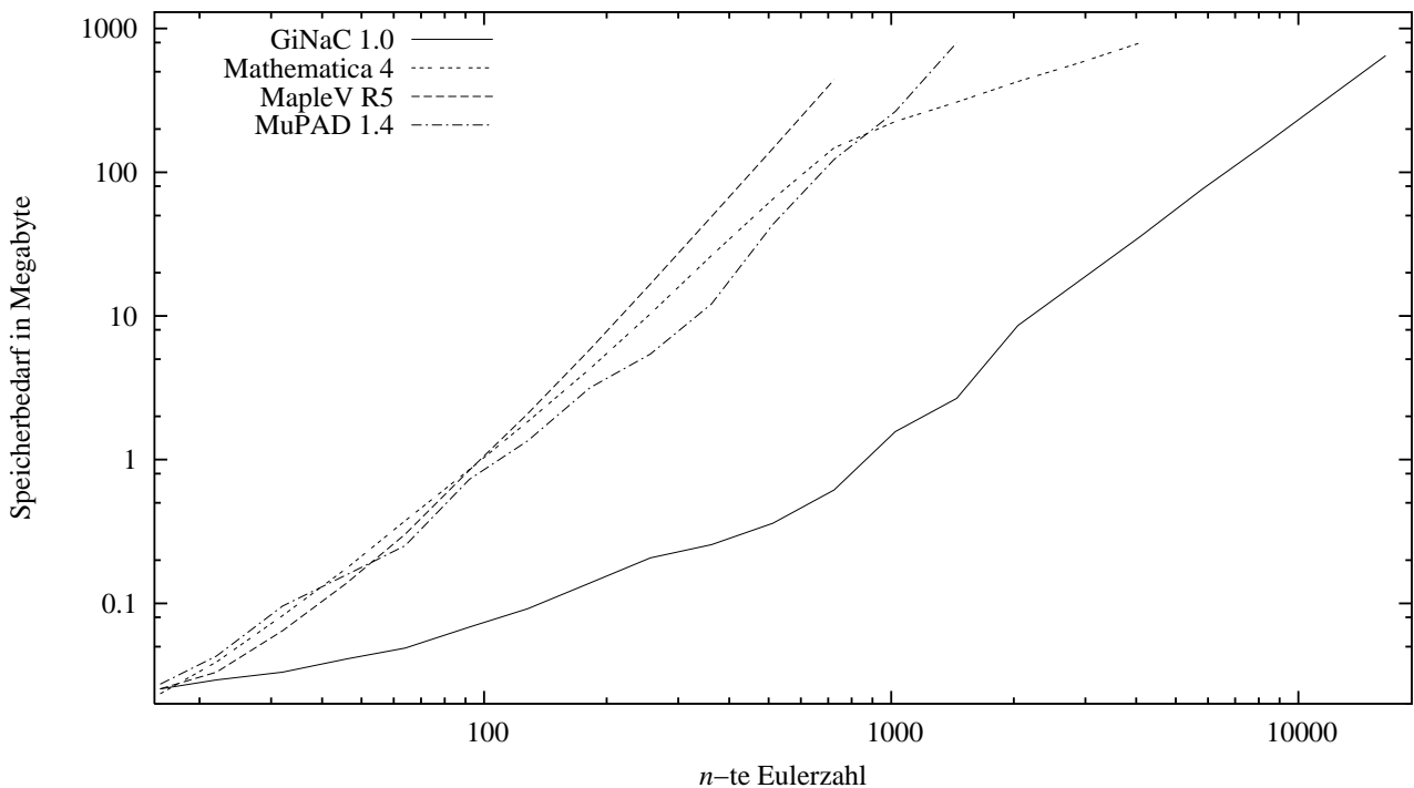
Abbildung 5.2.: Speicherbedarf verschiedener CA-Systeme für die Berechnung von Eulerzahlen. Alle Messungen wurden auf der Architektur Intel-x86 durchgeführt.
