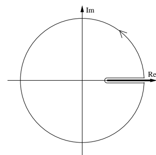
Abbildung A.8.: Integrationsweg zum Schnitt von \text{Li}_2(z)
