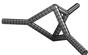
Abbildung 1.2.: Die gekreuzte Dreibeinfunktion
