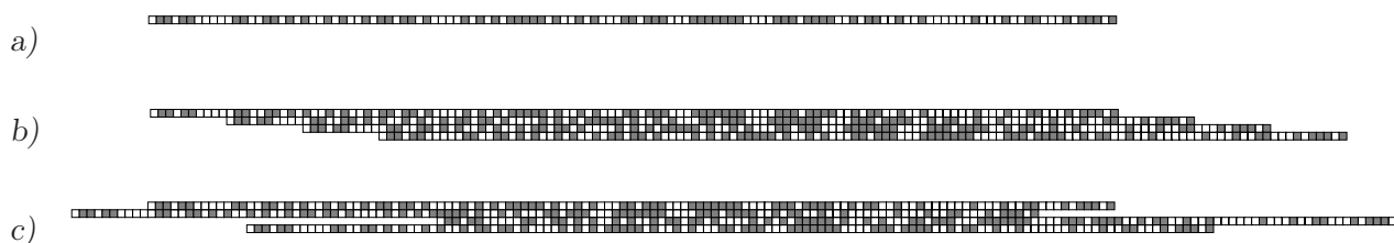
Abbildung B.3.: (a) die 127 Bit der vollständigen Schieberegister-Reihe zum primitiven Polynom x^7 + x^3 + 1 \pmod 2 und zwei verschiedene Wege, daraus Zufallszahlenfolgen aus Wörtern à vier Bit zu bilden: (b) Tausworthe-Reihe aus vier um O = 9 versetzten Schieberegister-Reihen und (c) Kirkpatrick-Stoll-Reihe initialisiert mit \{4, 11, 11, 4, 1, 7, 14\} = \{\text{11}, \text{11}, \text{11}, \text{11}, \text{11}, \text{11}\} .
