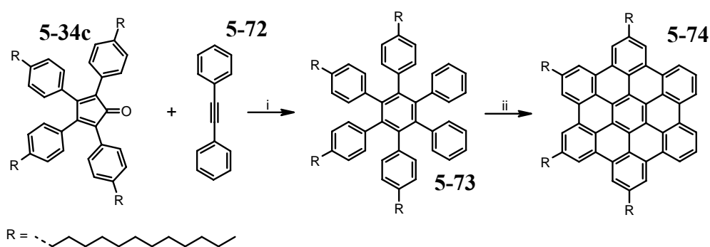
Scheme 5-19: i) 93%; ii) FeCl_3 , 93%.
