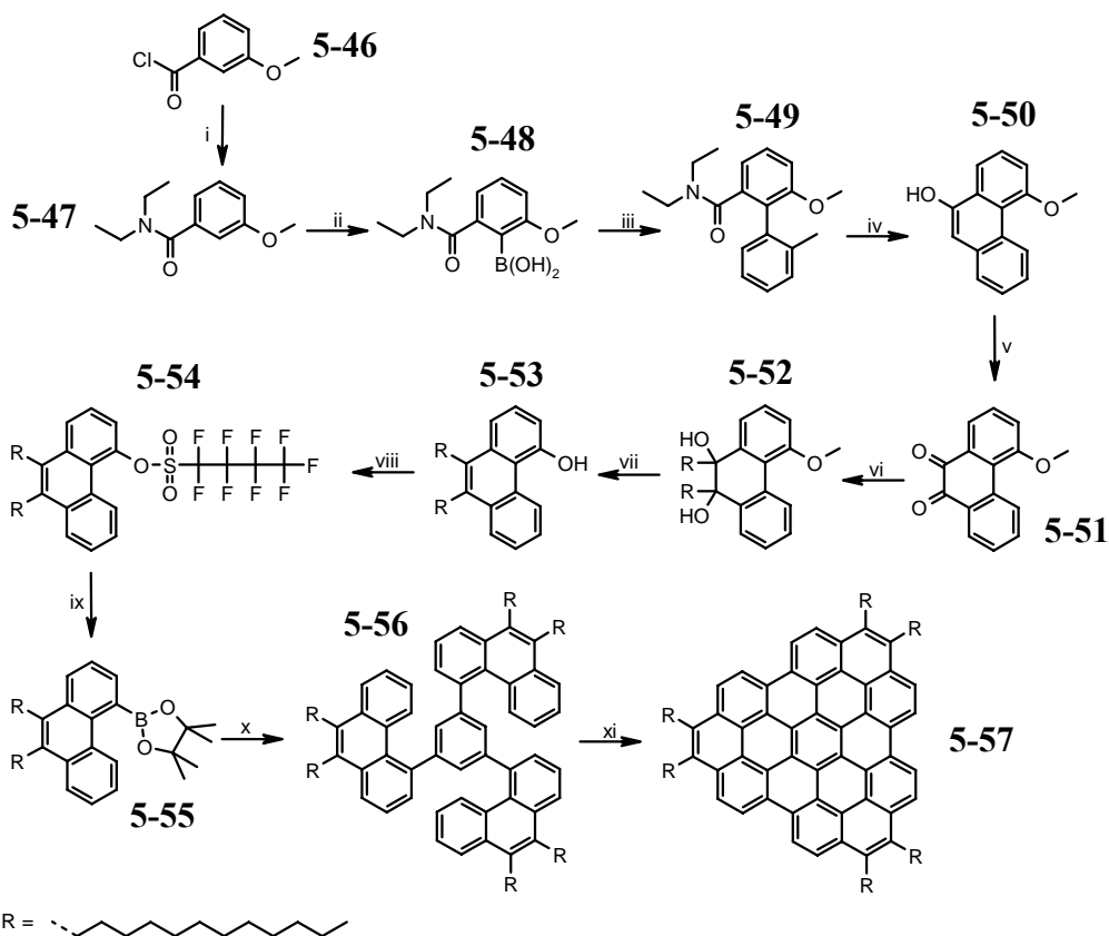
Scheme 5-15: i) \text{NEt}_3 , 99%; ii) ^t\text{BuLi} , \text{B}(\text{OMe})_3 , 62%; iii) \text{Pd}(\text{PPh}_3)_4 , 2-iodotoluene, \text{Na}_2\text{CO}_3 , 81%; iv) \text{LDA} , 94%; v) \text{O}_2 , salcomine, 99%; vi) \text{RMgBr} ; vii) \text{HIO}_3 , \text{AcOH} ; viii) \text{NfF} , 90% (three steps); ix) \text{Pd}(\text{PPh}_3)_4 , bispinacolatodiborane, \text{KOAc} , 72%; x) 1,3,5-tribromobenzene, \text{Pd}(\text{PPh}_3)_4 , \text{Ba}(\text{OH})_2 , 8%; xi) \text{FeCl}_3 , 83%.
