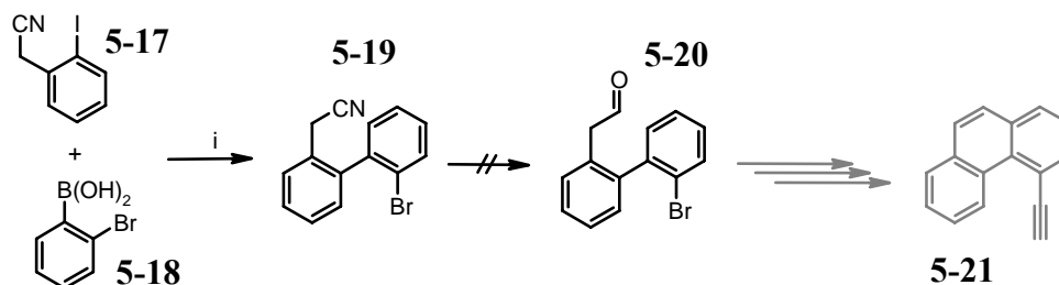
Scheme 5-6: i) Pd(PPh 3 ) 4 , 93%.
