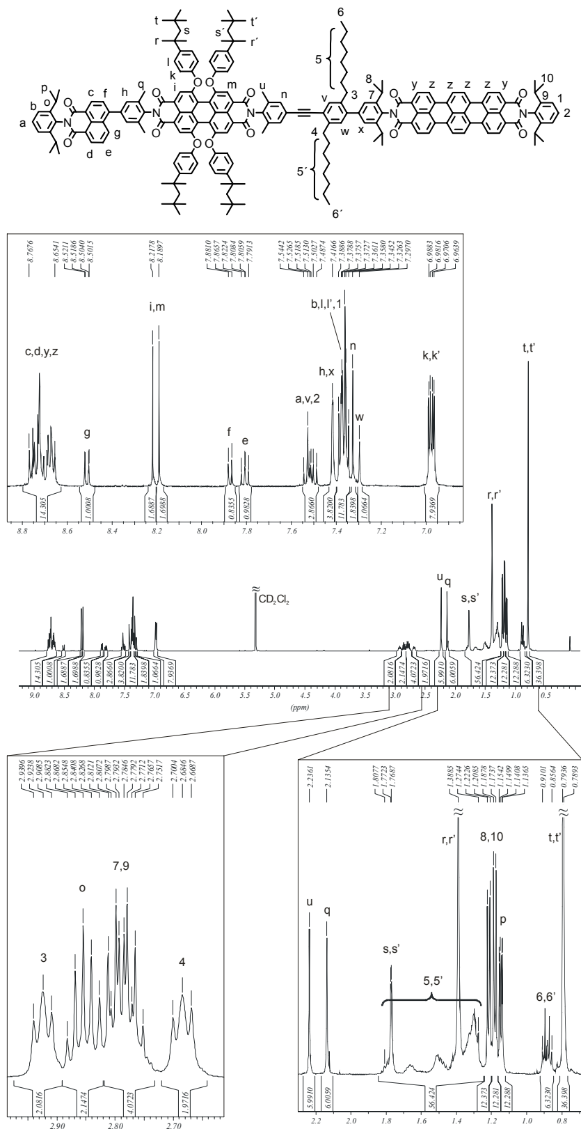
Abbildung 225: 500 MHz 1 H-NMR-Spektrum von 247 (CD 2 Cl 2 , 303 K)
