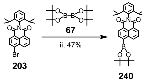
Abbildung 215: Darstellung des Boronsäureester-funktionalisierten NMI-Derivats 240 i) 67 , Kaliumacetat, Dioxan, Pd(dppf), 75 °C, 16 h, 47%
