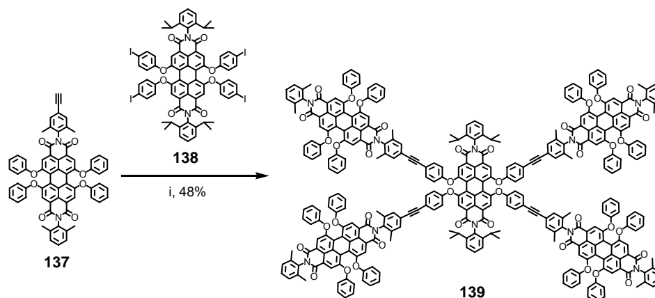
Abbildung 97: Synthese des Multichromophors 139 i) 138 , CuI, PPh 3 , Pd(PPh 3 ) 2 Cl 2 , THF/TEA, RT, 16 h, 48%
