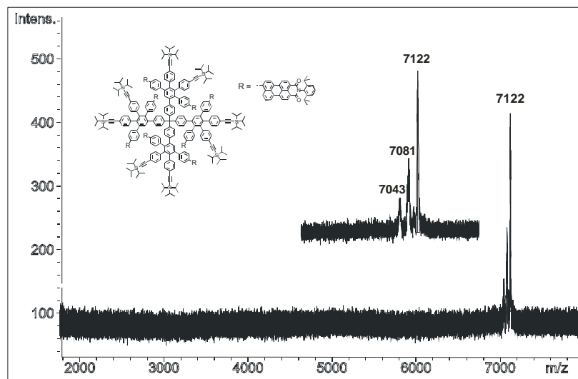
Abbildung 31: MALDI-TOF-Massenspektrum des Dendrimers 74
