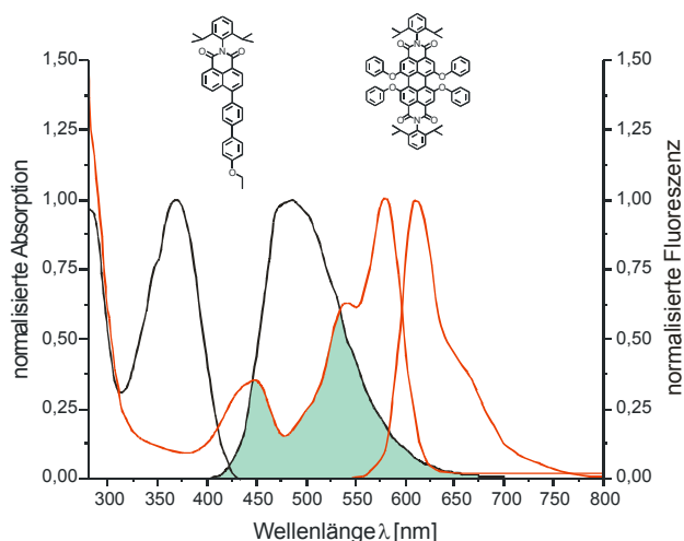
Abbildung 187: Absorptions- und Emissionsspektren des NMI-Chromophors 209 (schwarz) sowie des PDI-Chromophors 17 (rot). Die spektrale Überlappung zwischen der Fluoreszenz des NMI-Donors und der Absorption des PDI-Akzeptors ist grün hervorgehoben
