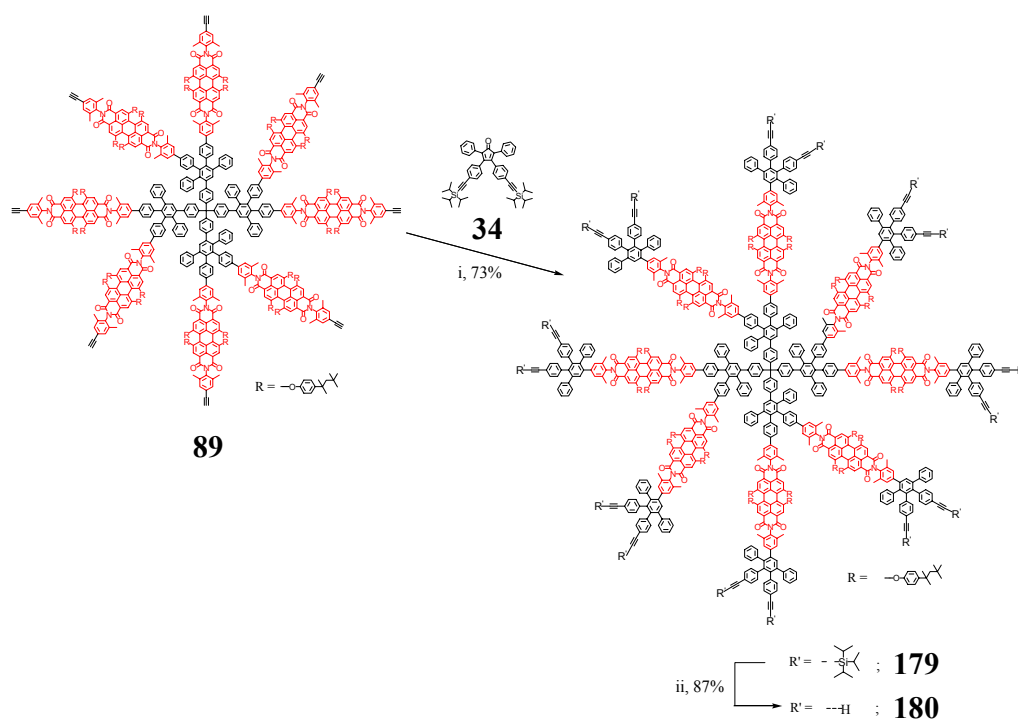
Abbildung 142: Einführung einer zweiten Generation zur Verdoppelung der Ethin-Funktionen i) 34 , Diphenylether, 170 °C, 3 d, 73%; ii) TBAF, THF, RT, 1 h, 87%
