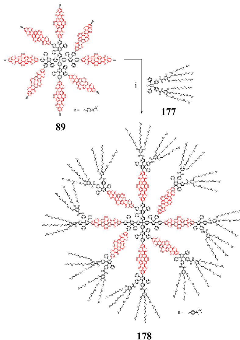
Abbildung 141: Darstellung des TEG-funktionalisierten Polyphenylen-Dendrimers 178 i) 177 , Diphenylether/Tetraethylenglykol, 170 °C, 4 d
