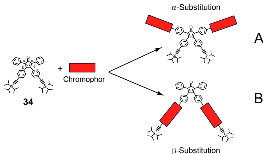
Abbildung 22: Einführung der Chromophore in zwei unterschiedliche Positionen des Cyclopentadienon-Verzweigungsbausteins
