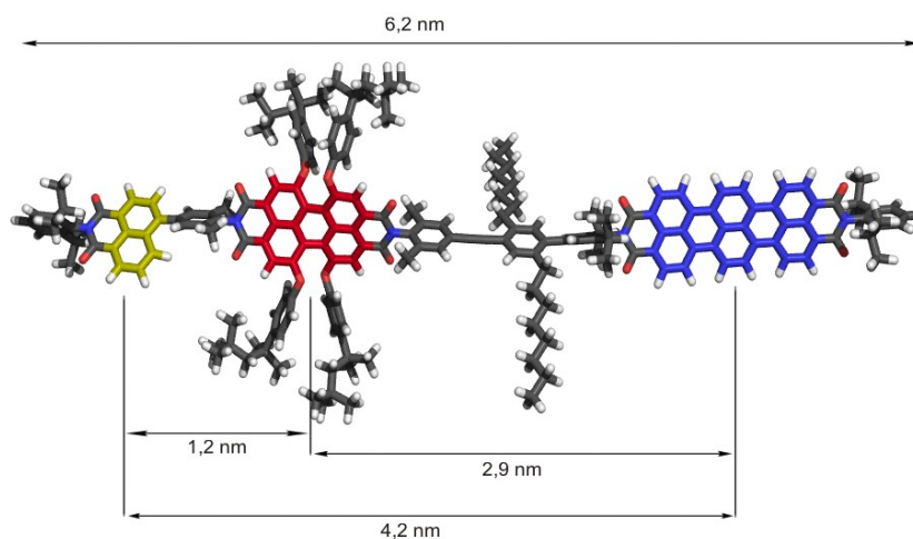
Abbildung 226: Molekularmechanisch optimierte 3D-Struktur von 247
