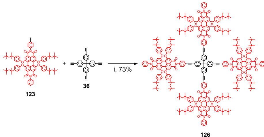
Abbildung 79: Synthese des Multichromophors 126 i) CuI, PPh 3 , Pd(PPh 3 ) 2 Cl 2 , THF/TEA, 40 °C, 16 h, 73%
