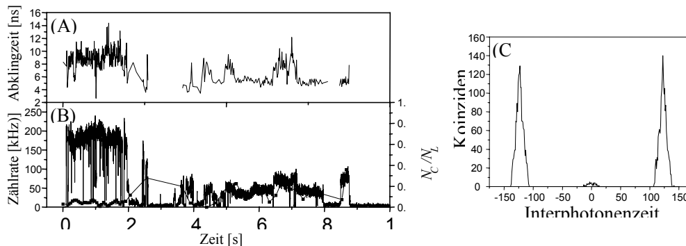
Abbildung 58: Fluoreszenzzeitspur (B, durchgezogenen Line), zeitaufgelöste Fluoreszenzabklingzeiten (A) und N_C/N_L -Werte (B, Quadrate) von 74 in Zeonex sowie die Verteilung der Interphotonenzeiten (C), gemessen innerhalb der ersten Fluoreszenzintensität der Fluoreszenzzeitspur
