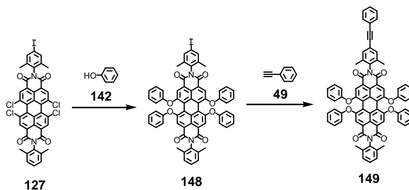
Abbildung 103: Synthese der Modellverbindung 149
