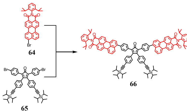
Abbildung 23: Benötigte Bausteine zur Darstellung des zweifach PMI-beladenen Verzweigungsbausteins 66
