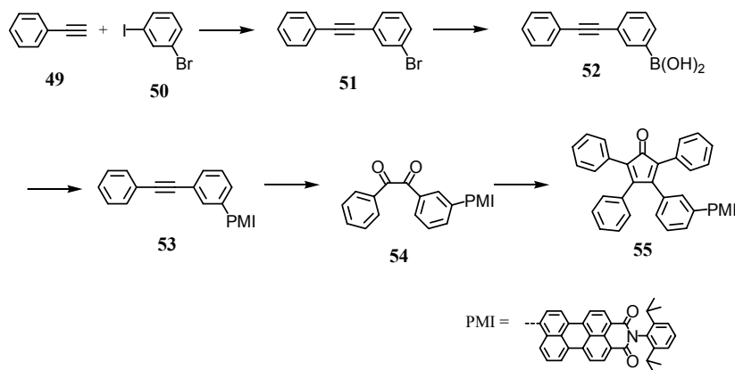
Abbildung 17: Syntheseweg zum Farbstoff-beladenen Cyclopentadienon-Baustein 55
