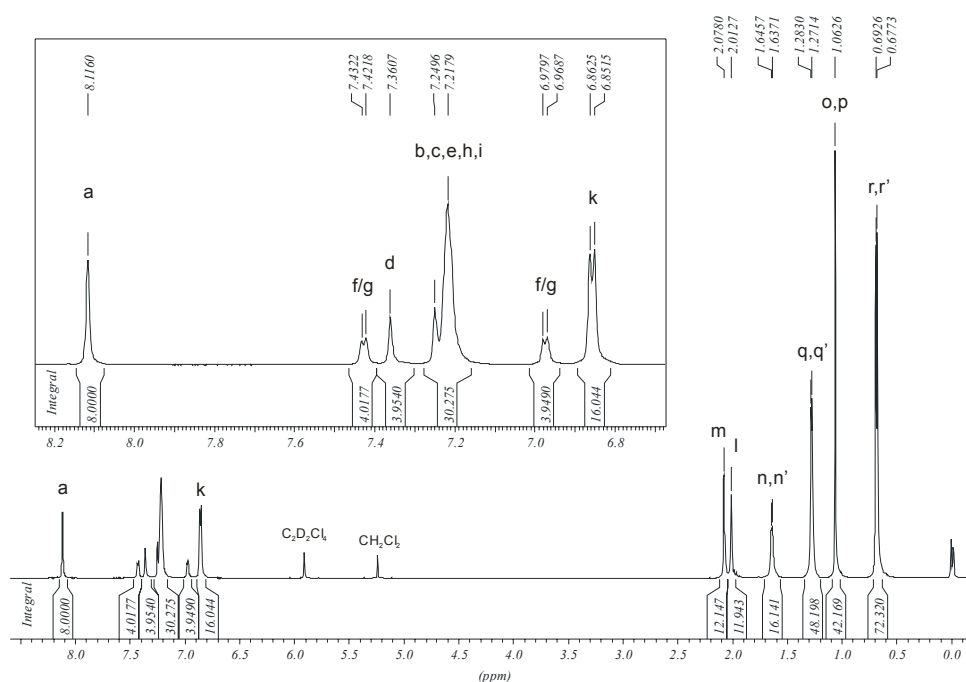
Abbildung 45: 700 MHz ^1H -NMR-Spektrum von 87 ( C_2D_2Cl_4 , 298 K)
