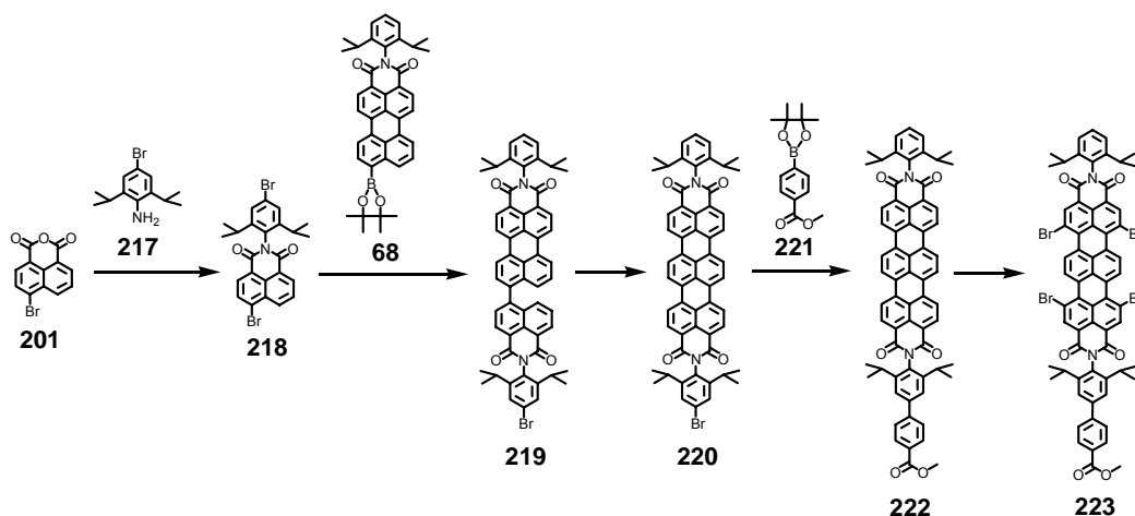
Abbildung 200: Syntheseweg zum Brom-funktionalisierten TDI-Chromophor 223 , der über die Carbonsäure die Anbindung an ein Halbleitermaterial ermöglicht
