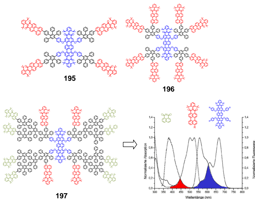
Abbildung 167: Multichromophore Polyphenylen-Dendrimere 195 , 196 und 197 , in denen ein effizienter Energietransfer beobachtet wird. Die spektrale Überlappung zwischen der Emission des NMIs und der Absorption des PMIs sowie zwischen der Emission des PMIs und der Absorption des TDIs ist in dem Spektrum rot bzw. blau hervorgehoben
