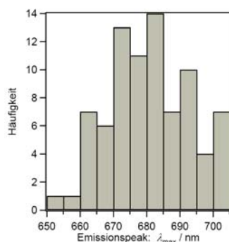
Abbildung 180: Histogramm der gemittelten TDI-Emissionsmaxima im vorderen Bereich der Fluoreszenzzeitpur. Die Emissionsmaxima (Integrationszeit: 1 s) können im Verlauf der Zeitspur um bis zu 10 nm variieren (vergleiche Abbildung 179)
