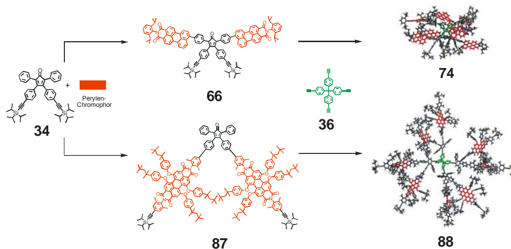
Abbildung 231: Strukturformeln der \alpha - bzw. \beta -verknüpften Verzweigungsbausteine 66 und 87 sowie die 3D-Strukturen der resultierenden ersten Generationen 74 und 88
