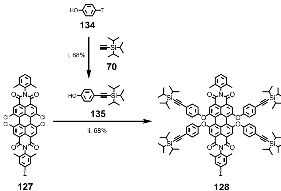
Abbildung 87: Synthese des A 4 B-Verzweigungsbausteins 128 i) 70 , CuI, PPh 3 , Pd(PPh 3 ) 2 Cl 2 , THF/TEA, RT, 16 h, 88%; ii) 135 , K 2 CO 3 , NMP, 90 °C, 24 h; 68%
