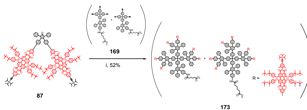
Abbildung 137: Synthese des sechsfach PDI-beladenen Dendrimers mit einer Carbonsäure-Funktion 173 i) 169 , Diphenylether, 170 °C, 5 d, 52%
