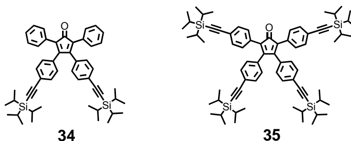
Abbildung 11: A 2 B Baustein 34 und A 4 B Baustein 35
