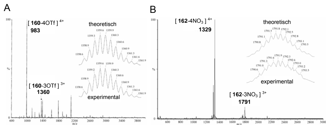
Abbildung 124: ESI-Massenspektren von 160 (A) und 162 (B). Als Einschub sind jeweils die theoretisch und experimentell bestimmten Molekular-massensignale angegeben.
