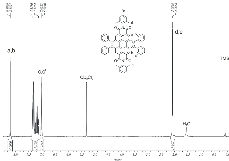
Abbildung 92: 300 MHz ^1\text{H} -NMR-Spektrum von 143 ( \text{CD}_2\text{Cl}_2 , 298 K)
