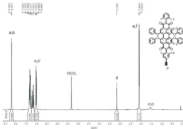
Abbildung 95: 300 MHz ^1\text{H-NMR} -Spektrum von 137 ( \text{CD}_2\text{Cl}_2 , 298 K)
