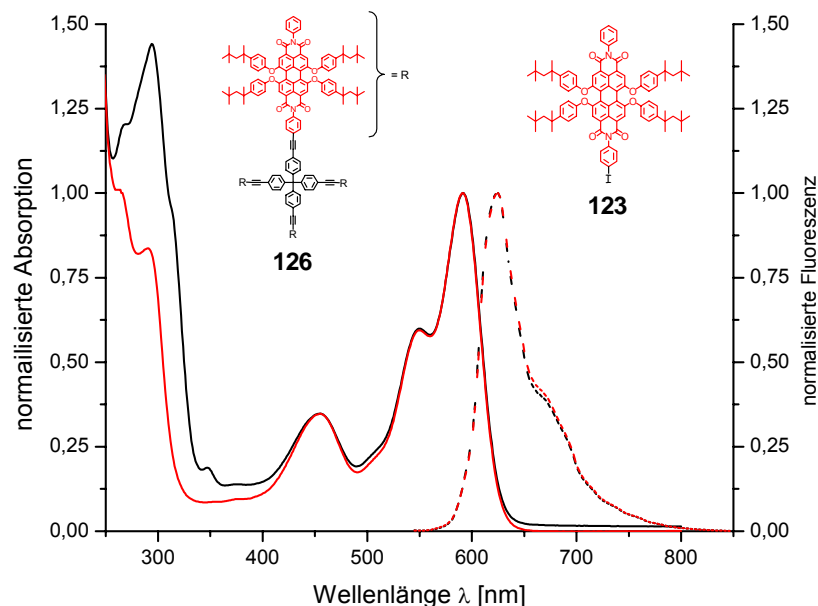
Abbildung 83: Normalisierte Absorptions- (durchgezogen) und Fluoreszenz-spektren (gestrichelt, Anregung: 540 nm) von 123 (rot) und 126 (schwarz) in \text{CHCl}_3
