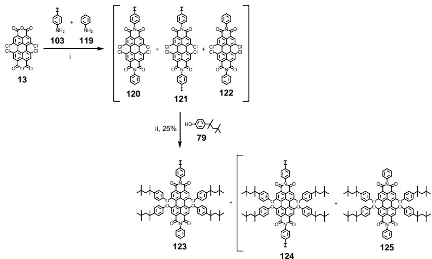
Abbildung 76: Synthese des desymmetrisierten PDI-Chromophors 13 i) 4-Iodanilin ( 103 ), Anilin ( 119 ), Propionsäure, 150 °C, 16 h; ii) 79 , NMP, K 2 CO 3 , 64 h, 90 °C, 25%
