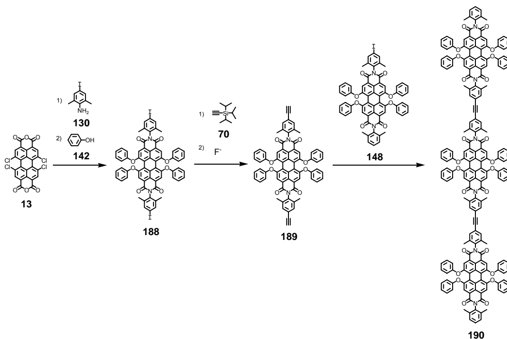
Abbildung 159: Darstellung des Trimers 190
