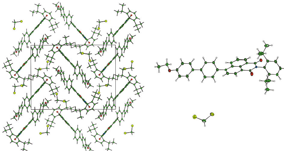
Abbildung 185: Kristallstruktur des NMI-Chromophors 209
