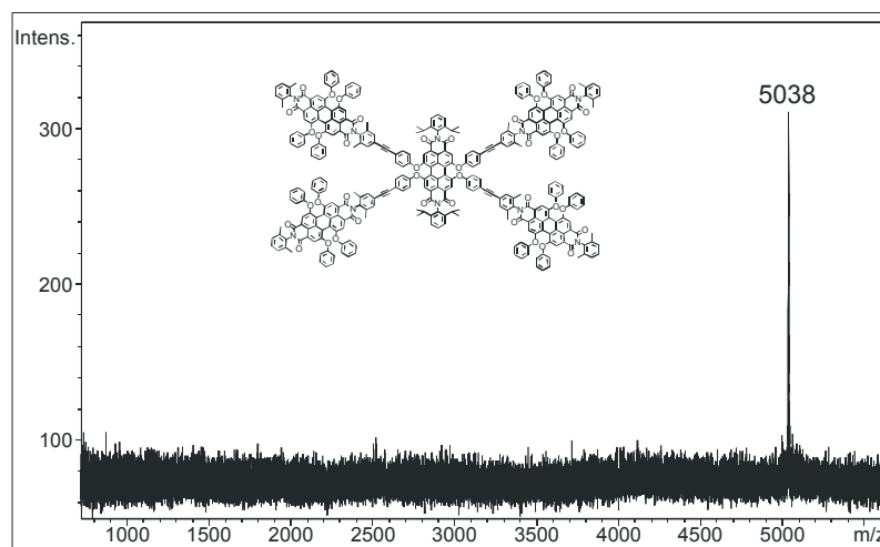
Abbildung 98: MALDI-TOF-Massenspektrum von 139
