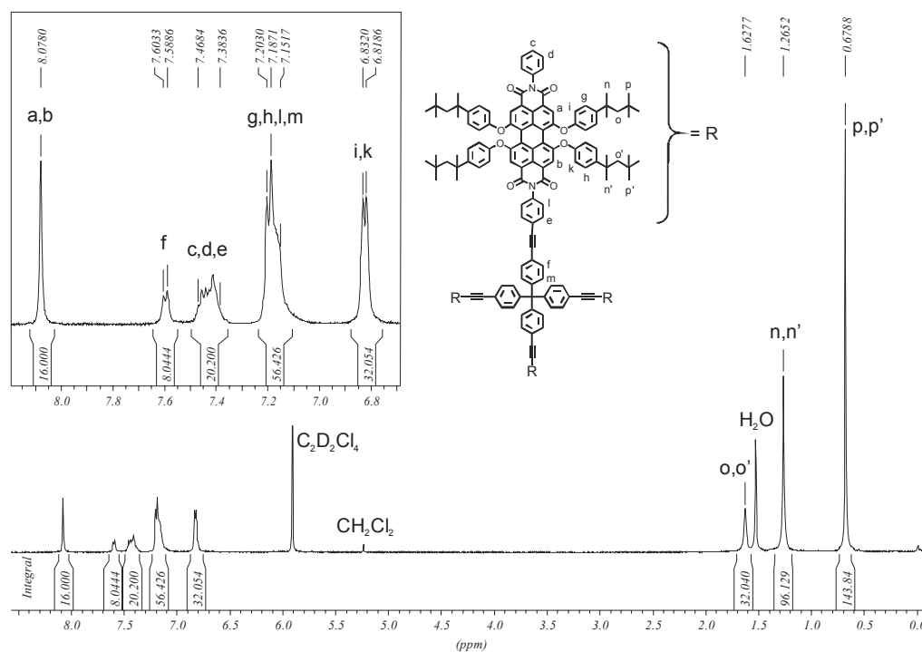
Abbildung 81: 500 MHz ^1\text{H-NMR} -Spektrum von 126 ( \text{C}_2\text{D}_2\text{Cl}_4 , 298 K)
