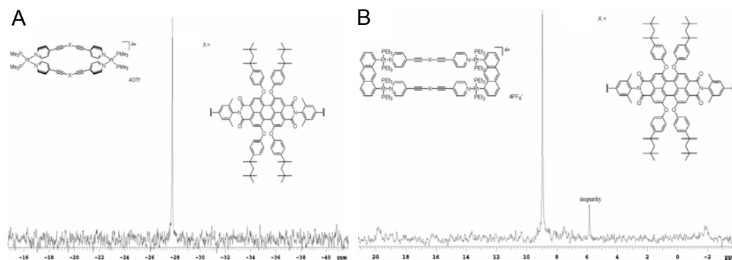
Abbildung 125: ^{31}\text{P} -NMR-Spektren von 160 (A) und 162 (B)
