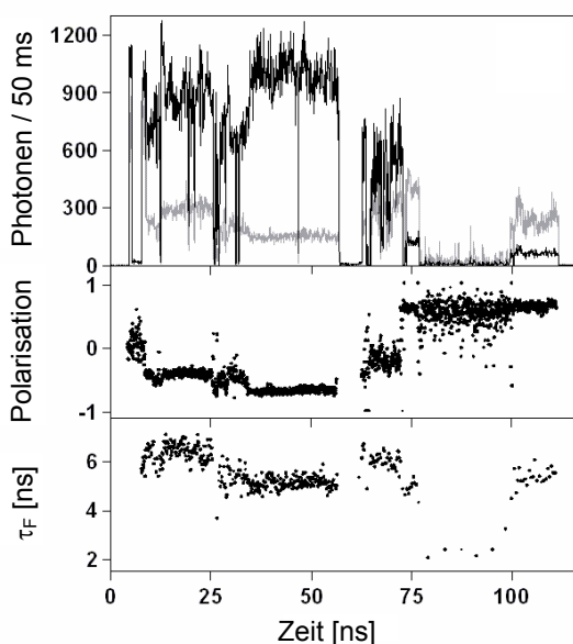
Abbildung 108: Fluoreszenzzeitkurve von 139 in PMMA und Umgebungsbedingungen (die Signale der beiden Detektoren sind in grau und schwarz wiedergegeben) mit den zeitaufgelösten Polarisationen und Fluoreszenzlebensdauern
