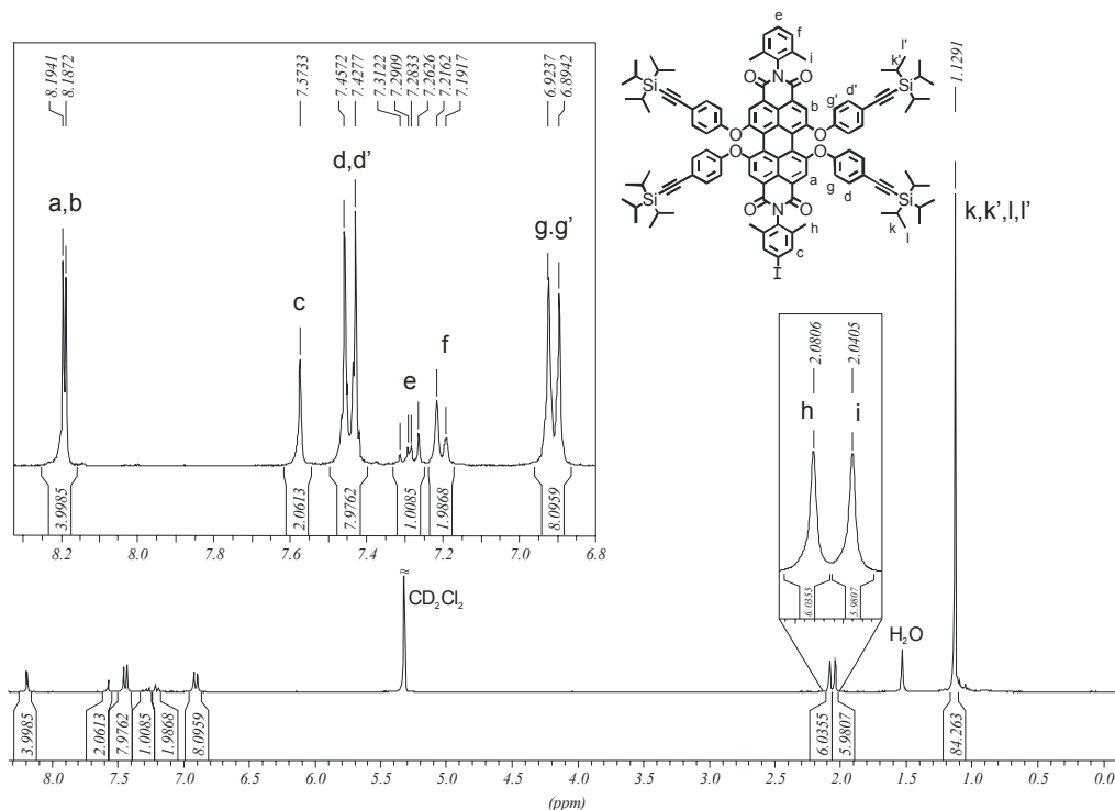
Abbildung 88: 300 MHz ^1\text{H-NMR} -Spektrum von 128 ( \text{CD}_2\text{Cl}_2 , 298 K)
