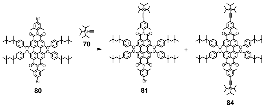
Abbildung 38: Reaktionsprodukte der statistische Hagihara-Reaktion
