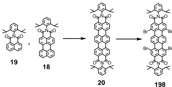
Abbildung 169: Darstellung des vierfach Brom-funktionalisierten TDI-Chromophors 198
