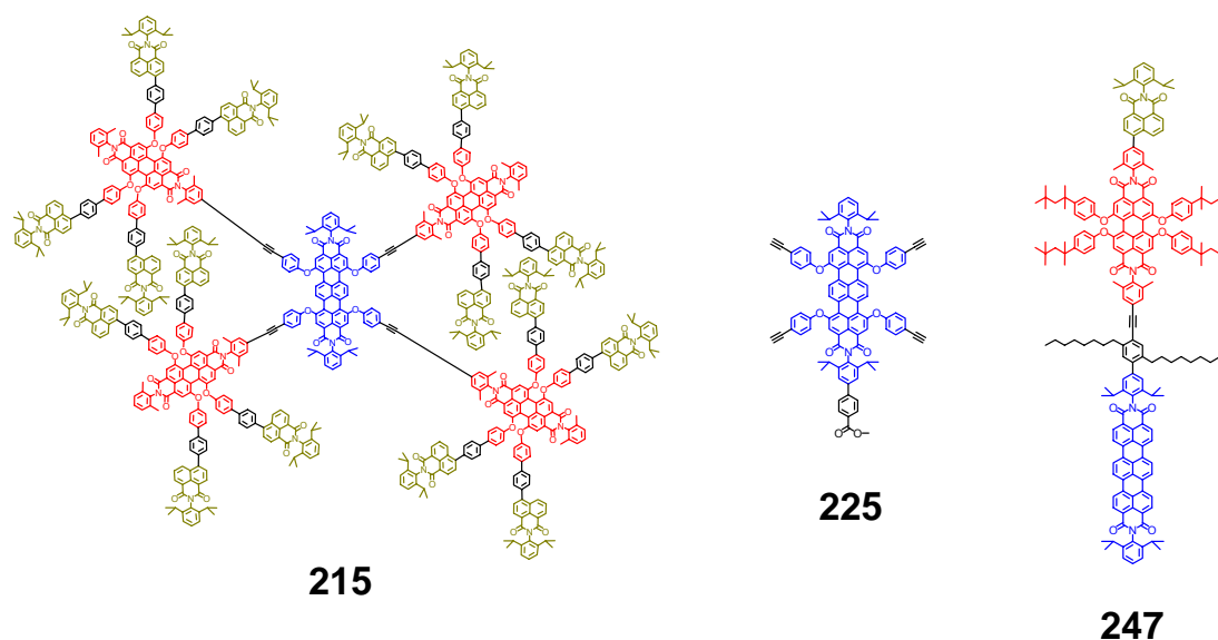
Abbildung 235: Strukturformeln der Triaden 215 und 247 sowie des Carbonsäurefunktionalisierten TDI-Kernbausteins 225
