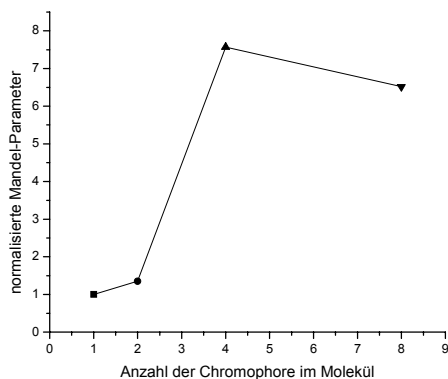
Abbildung 59: Auf 91 (■) normalisierte Mandel-Parameter von 92 (●), 93 (▲) und 74 (▼) ( 3 \mu\text{W} , gepulste Anregung, Zeonex, Umgebungsbedingungen)
