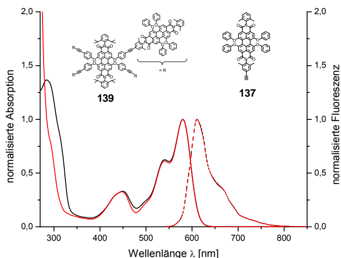
Abbildung 101: Absorptions- (durchgezogen) und Fluoreszenzspektren (gestrichelt, Anregung: 540 nm) von 137 (rot) und 139 (schwarz) in \text{CHCl}_3
