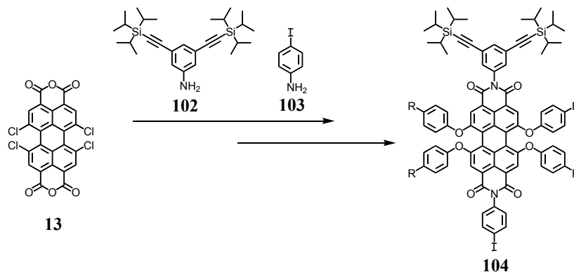
Abbildung 68: Angestrebter Syntheseweg zum Verzweigungsbaustein 104
