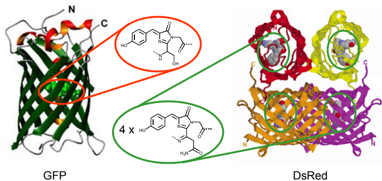
Abbildung 131: 3D-Struktur der fluoreszenten Proteine GFP (links) und DsRed (rechts) mit den Strukturformeln der entsprechenden Chromophore
