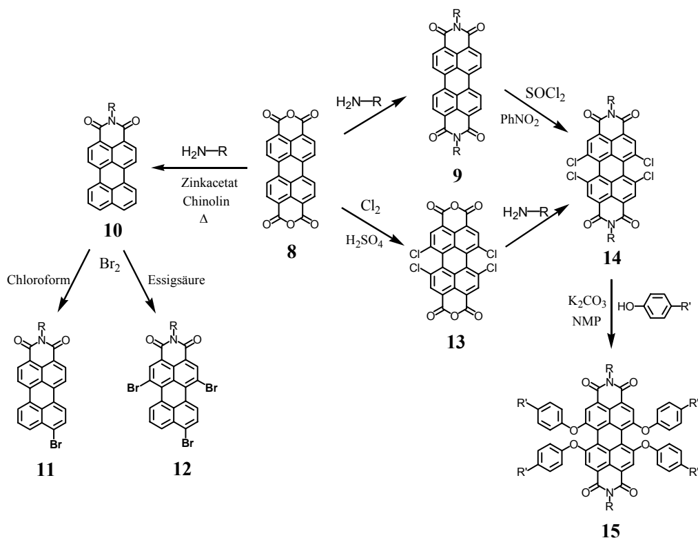
Abbildung 3: Darstellung von Perylenmonoimid- und Perylendiimid-Derivaten
