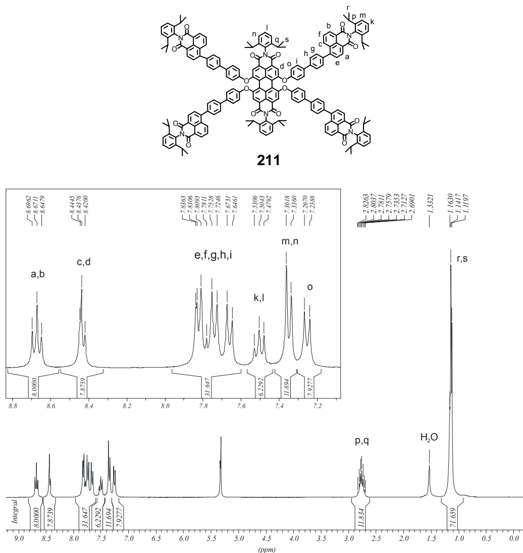
Abbildung 183: 300 MHz ^1\text{H-NMR} -Spektrum von 211 ( \text{CD}_2\text{Cl}_2 , 298 K)
