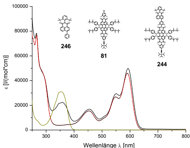
Abbildung 220: Absorptionsspektren der NMI-PDI-Diade 244 (schwarz) sowie der beiden als Modell-Farbstoff verwendeten Chromophore 246 (olivgrün) und 81 (rot)
