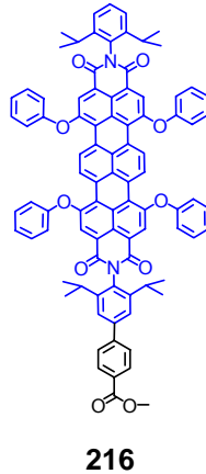
Abbildung 199: TDI-Chromophor 216 , der sich zur Fixierung auf einem Halbleitermaterial eignet
