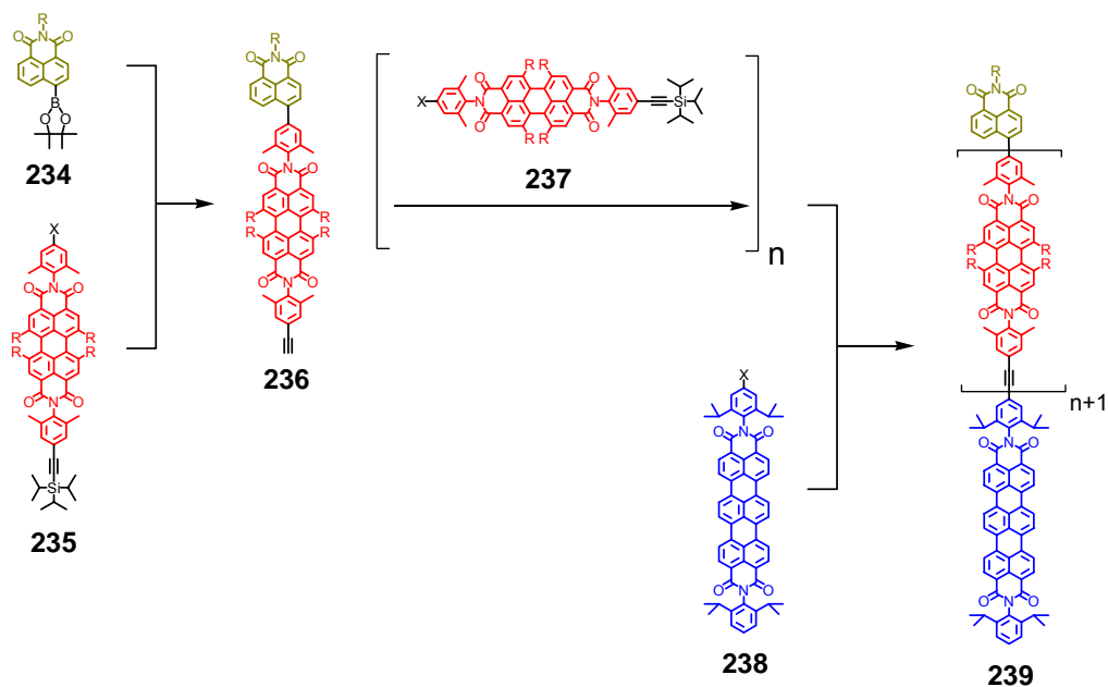
Abbildung 208: Geplanter Synthesepfad zur Darstellung eines molekularen Drahtes
