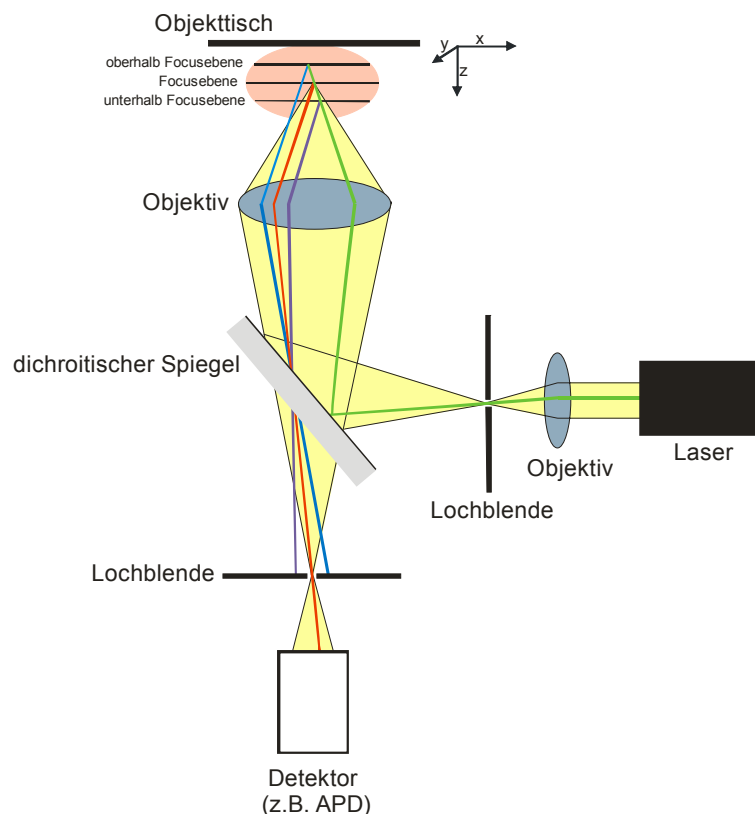
Abbildung 242: Schematischer Aufbau eines konfokalen Fluoreszenzmikroskops
