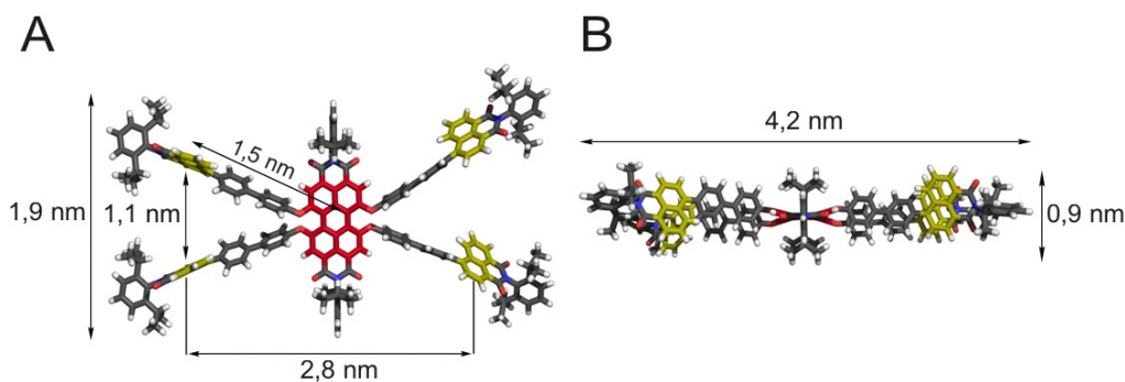
Abbildung 184: Molekularmechanisch optimierte 3D-Struktur von 211
