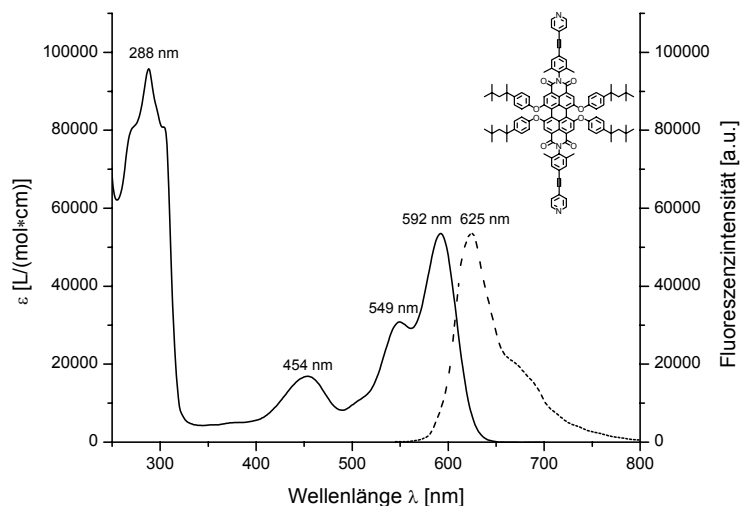
Abbildung 122: Absorptions- (durchgezogen) und Fluoreszenzspektrum (gestrichelt, Anregung: 540 nm) von 155 in \text{CHCl}_3
