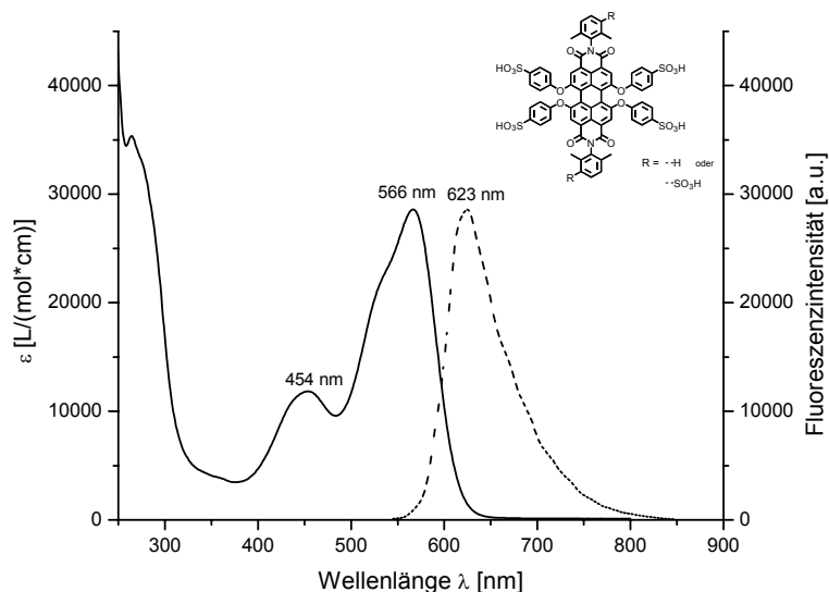
Abbildung 150: Absorptions- (durchgezogen) und Emissionsspektrum (gestrichelt, Anregung: 540 nm) von 182 in Wasser
