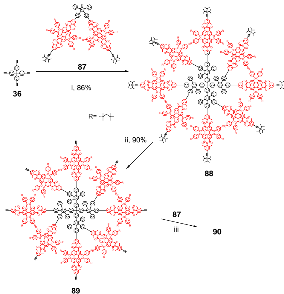
Abbildung 46: Darstellung der ersten ( 88 ) und zweiten Generation ( 90 ) \beta -verknüpfter, multichromophorer Polyphenylen-Dendrimere i) 87 , o -Xylol, 150 °C, 5d, 86%; ii) TBAF, THF, 1 h, 90 %; iii) 87 , Diphenylether, 200 °C, 18 d
