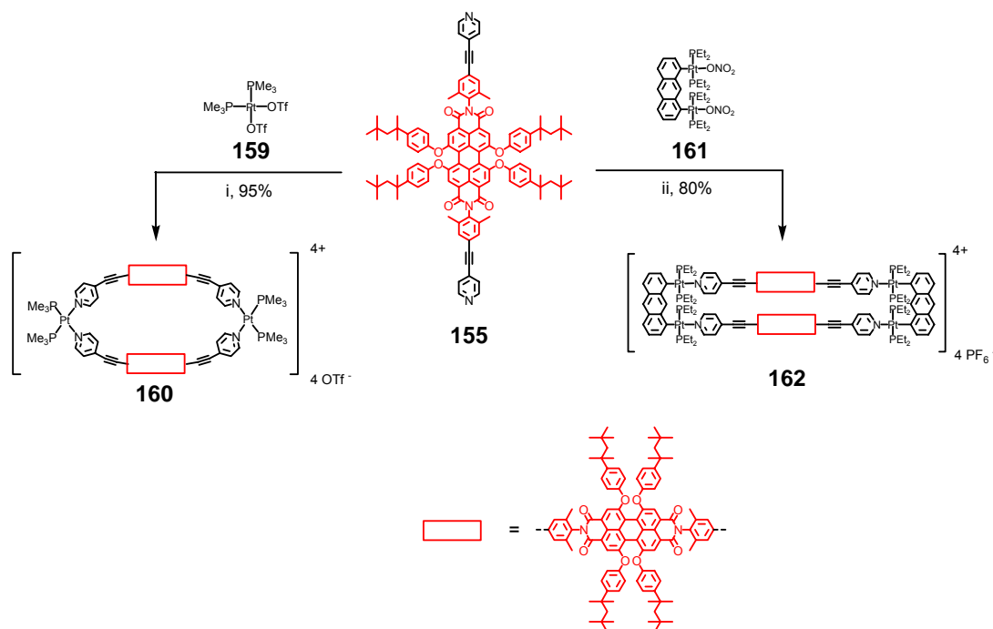
Abbildung 123: Darstellung der supramolekularen Strukturen 160 und 162 i) 159 , Aceton-d 6 , RT, 20 h, 95%; ii) 161 , \text{KPF}_6 , D 2 O/Aceton-d 6 , 50 °C, 5 d, 80%
