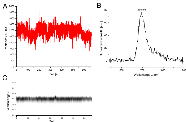
Abbildung 179: Einzelmolekülspektroskopische Ergebnisse einer PDI-TDI-Diade 200 , die ausschließlich TDI-Emission zeigt. A: Fluoreszenzzeitstrace von 200 in PMMA; B: Fluoreszenzspektrum zu dem in A mit einem schwarzen Balken gekennzeichneten Zeitpunkt; C: Zeitliche Veränderung der Emissionswellenlängen
