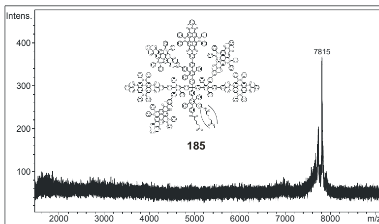
Abbildung 154: MALDI-TOF-Massenspektrum des Multichromophors 185 . Die Messung erfolgte unter Zusatz eines Natriumsalzes
