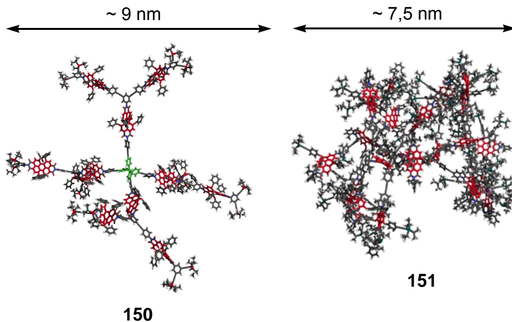
Abbildung 116: Molekularmechanisch optimierte 3D-Strukturen der zweiten Generationen 150 und 151 , die sich aus den Verzweigungsbausteinen 116 (links) und 128 (rechts) ergeben. Zur besseren Orientierung sind die Chromophore rot und der Kernbaustein (links) grün hervorgehoben
