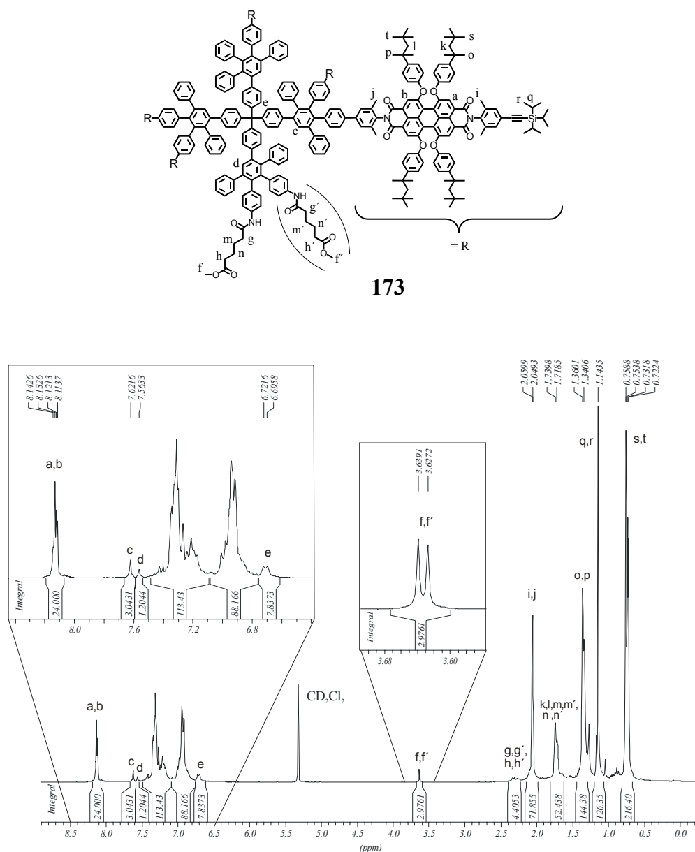
Abbildung 138: 300-MHz ^1H -NMR-Spektrum von 173 ( CD_2Cl_2 , 298 K)
