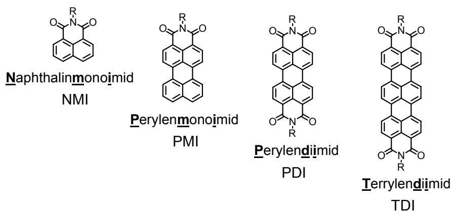
Abbildung 7: Übersicht über die Strukturformeln, Namen und Abkürzungen der in dieser Arbeit verwendeten Rylen-carbonsäureimide
