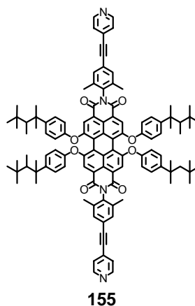
Abbildung 118: Strukturformel des angestrebten Pyridin-funktionalisierten PDI-Chromophors 155
