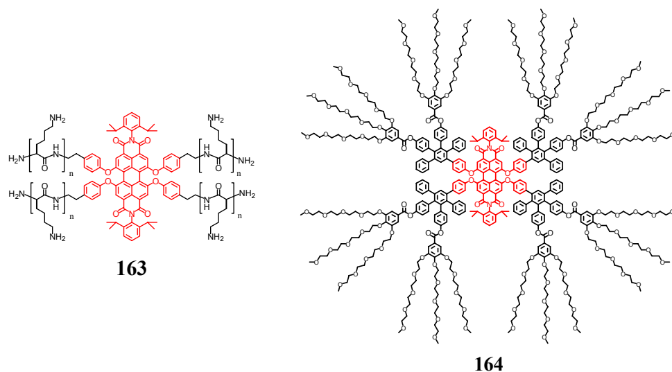
Abbildung 133: Wasserlösliche PDI-Chromophore durch die Einführung wasserlöslicher Polymerketten
