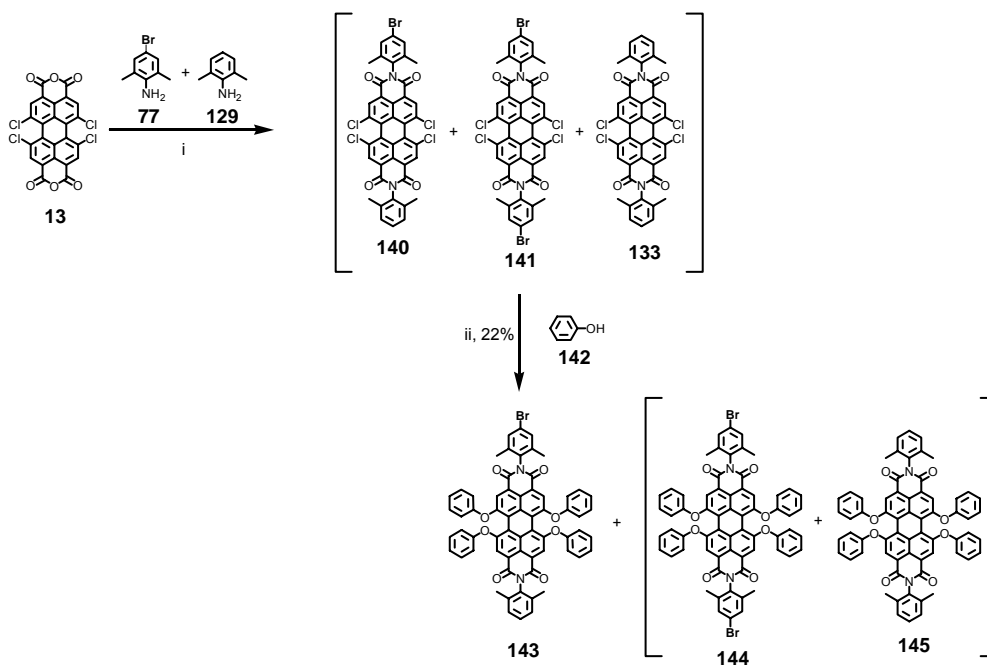
Abbildung 91: Synthese des desymmetrisierten PDI-Chromophors 143 i) 4-Brom-2,6-Dimethylanilin ( 77 ), 2,6-Dimethylanilin ( 129 ), Propionsäure, 150 °C, 16 h; ii) Phenol ( 142 ), NMP, K 2 CO 3 , 16 h, 90 °C, 22%
