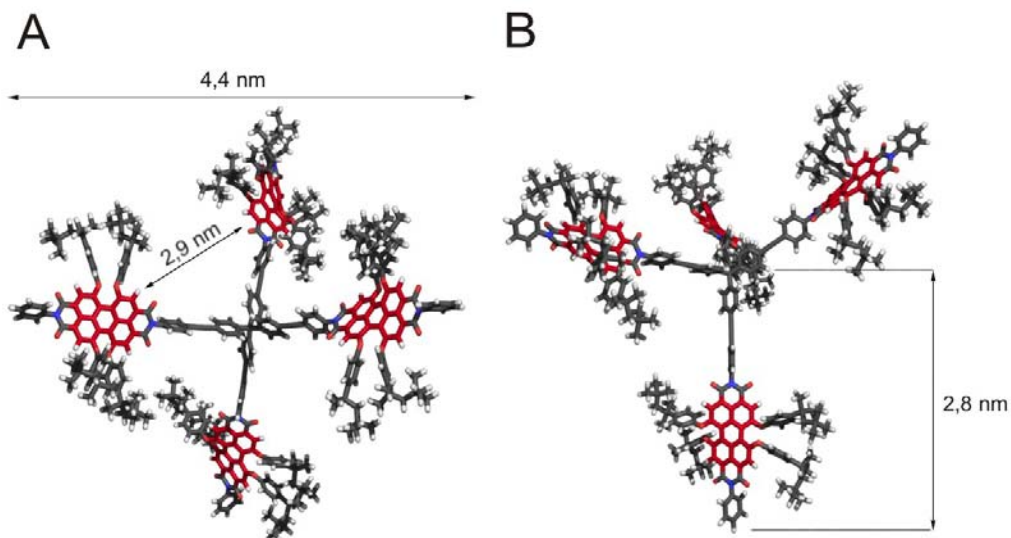
Abbildung 82: Molekularmechanisch optimierte 3D-Struktur von 126
