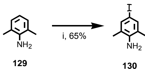
Abbildung 85: Synthese von 4-Iod-2,6-dimethylanilin ( 130 ) i) KI, KIO 3 , H 2 O, Methanol, HCl, RT, 3h
