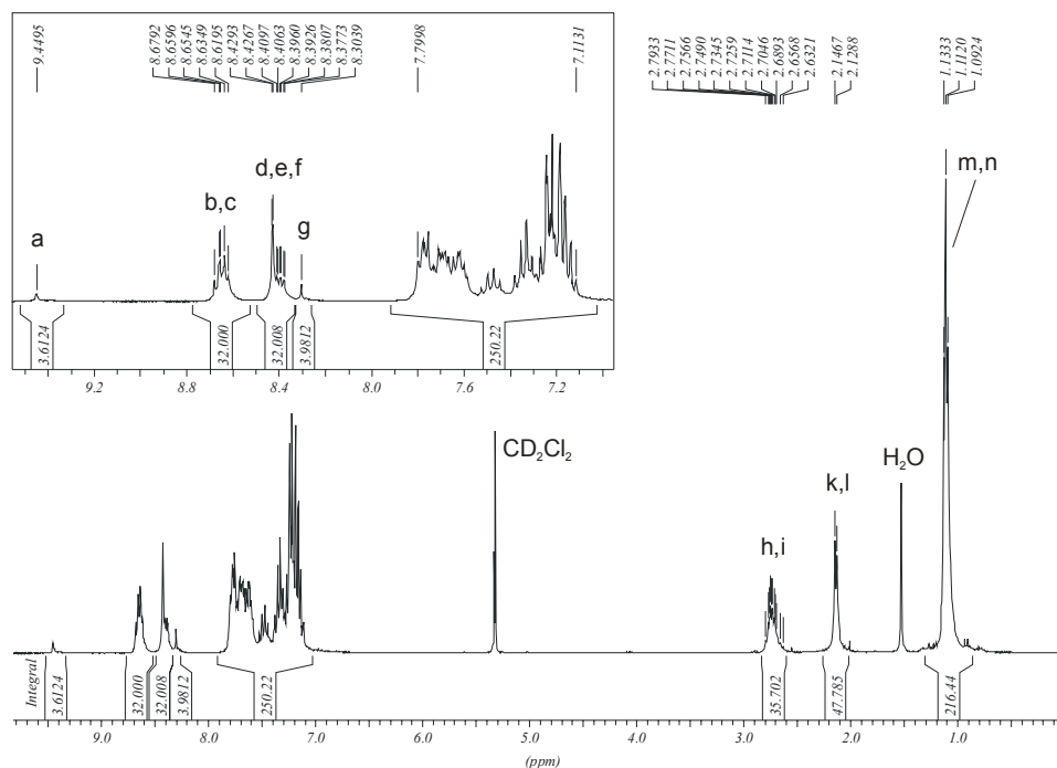
Abbildung 194: 250 MHz ^1\text{H} -NMR-Spektrum von 215 ( \text{CD}_2\text{Cl}_2 , 298 K)
