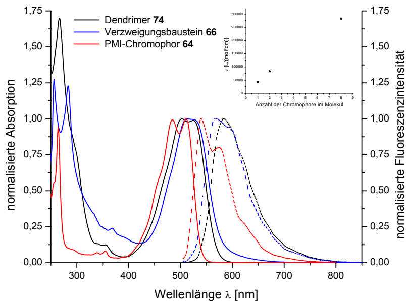
Abbildung 34: Normalisierte Absorptions- (durchgezogen) und Fluoreszenzspektren (gestrichelt, Anregung: 540 nm) von PMI 64 (rot), Verzweigungsbaustein 66 (blau) und erster Generation 74 (schwarz) in \text{CHCl}_3 . Einschub: Extinktionskoeffizienten in Abhängigkeit zur Anzahl der PMI-Chromophore im Molekül
