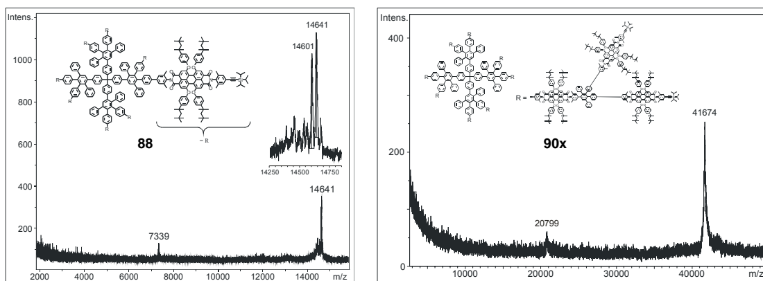
Abbildung 48: MALDI-TOF-Massenspektren von 88 und 90 . Die Messungen erfolgten unter Zusatz eines Natriumsalzes
