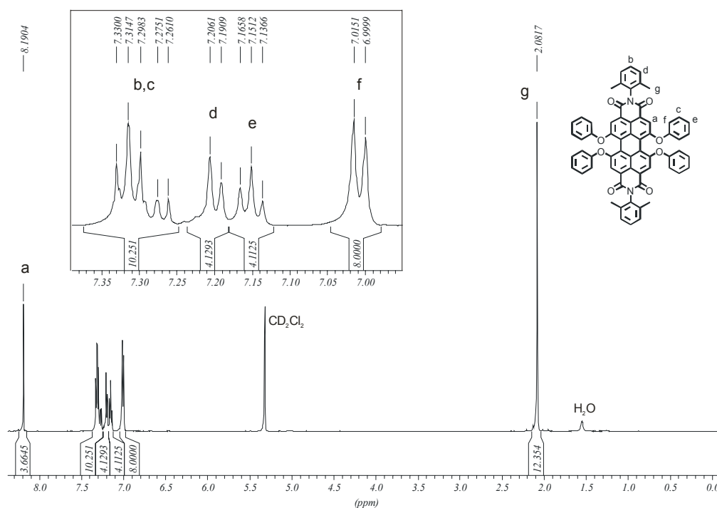
Abbildung 146: 300 MHz ^1\text{H-NMR} -Spektrum von 145 ( \text{CD}_2\text{Cl}_2 , 298 K)
