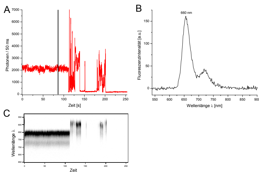
Abbildung 177: Einzelmolekülspektroskopische Ergebnisse einer PDI-TDI-Diade 200, die zuerst TDI-Emission eines Intensitätsniveaus und danach PDI-Emission zeigt. A: Fluoreszenzzeitkurve von 200 in PMMA; B: Fluoreszenzspektrum zu dem in A mit einem schwarzen Balken gekennzeichneten Zeitpunkt; C: Zeitliche Veränderung der Emissionswellenlängen
