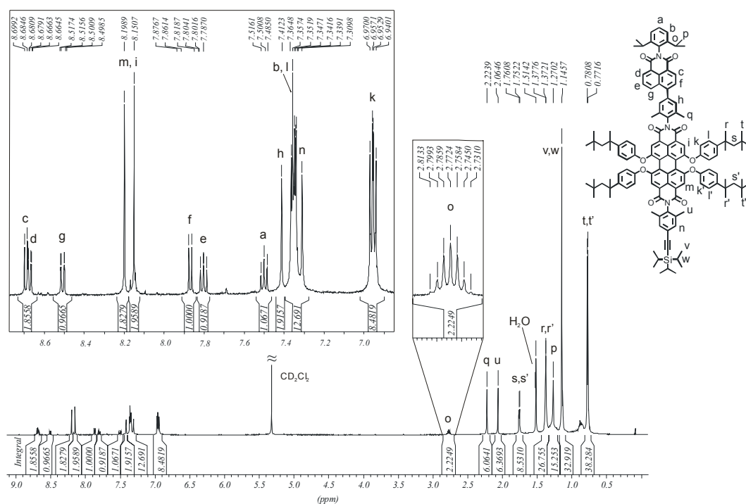
Abbildung 219: 500 MHz ^1\text{H-NMR} -Spektrum von 244 ( \text{CD}_2\text{Cl}_2 , 306 K)
