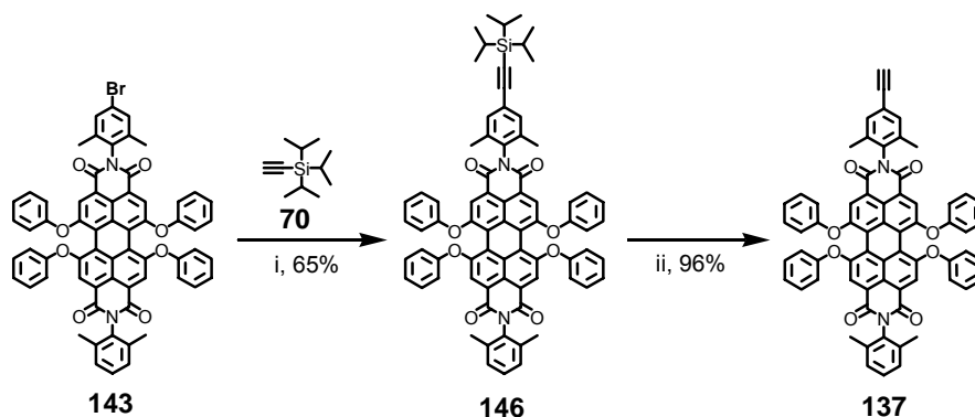
Abbildung 94: Synthese des Ethin-funktionalisierten PDI-Chromophors 137 i) 70 , \text{CuI} , \text{PPh}_3 , \text{Pd}(\text{PPh}_3)_2\text{Cl}_2 , THF/TEA, 90 °C, 16 h, 65%; ii) TBAF, THF, RT, 1 h, 96%
