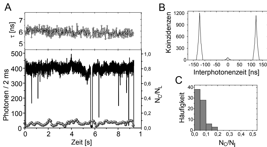
Abbildung 63: A) Fluoreszenzzeitspur von 88 in Zeonex unter Umgebungsbedingungen ( 3 \mu\text{W} , Anregung: 543 nm, 8.13 MHz) mit den entsprechenden zeitaufgelösten Fluoreszenzlebenszeiten (oben) und den N_C/N_L -Werten (gemessen alle 50000 Photonen) (unten); B) Interphotonenzeiten über die gesamte Zeitspur betrachtet; C) Histogramm der N_C/N_L -Werte von 75 Molekülen
