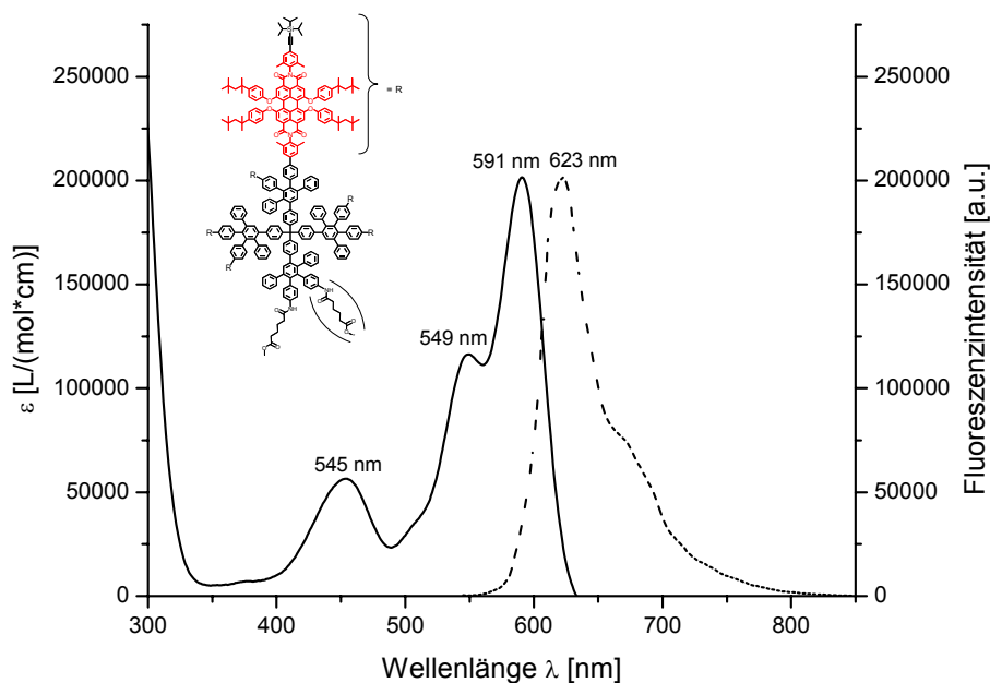
Abbildung 139: Absorptions- (durchgezogen) und Emissionsspektrum (gestrichelt, Anregung: 540 nm) von 173 in \text{CH}_3\text{Cl}
