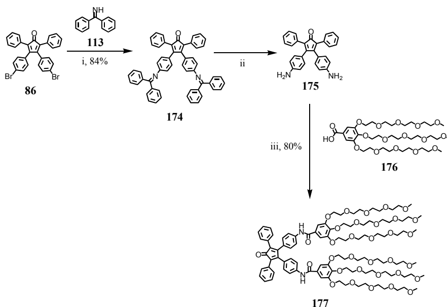
Abbildung 140: Darstellung des TEG-funktionalisierten Cyclopentadienonbausteins 177 i) Benzophenonimin ( 113 ), \text{Cs}_2\text{CO}_3 , \text{Pd}_2(\text{dba})_3 , BINAP, Toluol, 80\text{ }^\circ\text{C} , 6 d, 84%; ii) HCl, THF, 0\text{ }^\circ\text{C} , 30 min; iii) 176 , EDC, Dimethylaminopyridin, DMF/ \text{CH}_2\text{Cl}_2 , TEA, RT, 7 d, 80%
