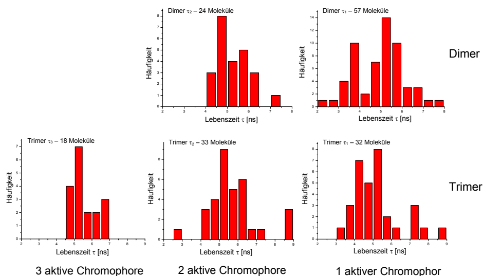
Abbildung 213: Histogramme der Fluoreszenzlebensdauern von 187 und 190 in Anwesenheit unterschiedlich vieler aktiver Chromophore
