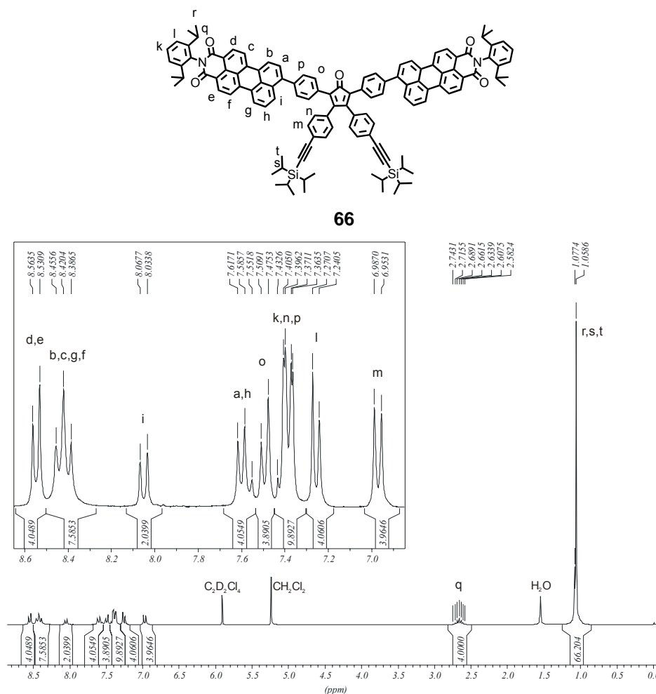
Abbildung 28: 250 MHz ^1\text{H} -NMR-Spektrum von 66 ( \text{C}_2\text{D}_2\text{Cl}_4 , 298 K)
