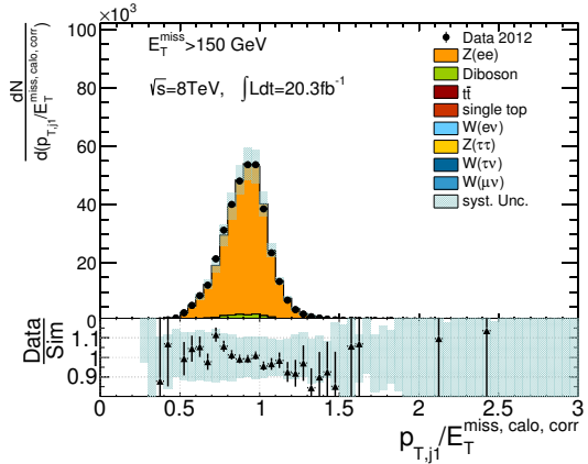
(d) p_T/E_T^{\text{miss}}
