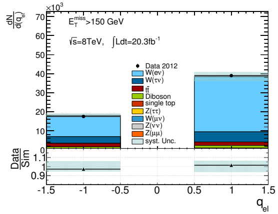
(d) Charge
